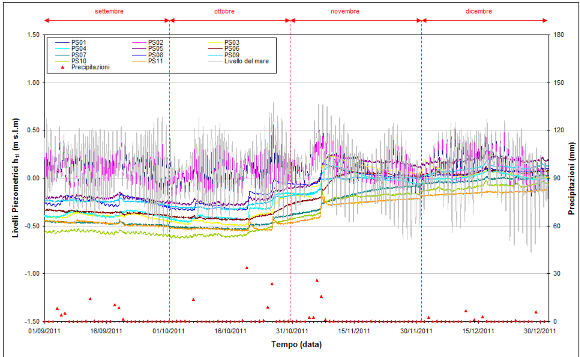
Fig. 2.6 - Livelli piezometrici ( h_u ) relativi ai piezometri superficiali nel periodo di monitoraggio 01/09/2011 - 31/12/2011.
