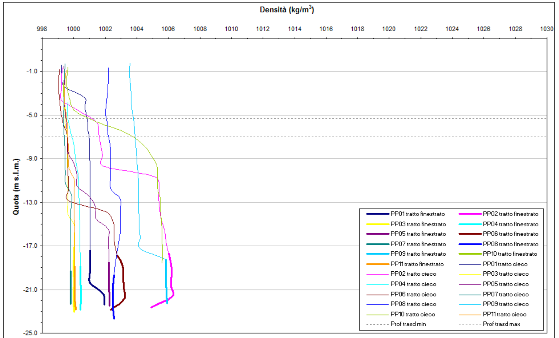
Fig. 4.7 - Profili verticali di densità piezometri profondi - 6-7 dicembre 2011.
