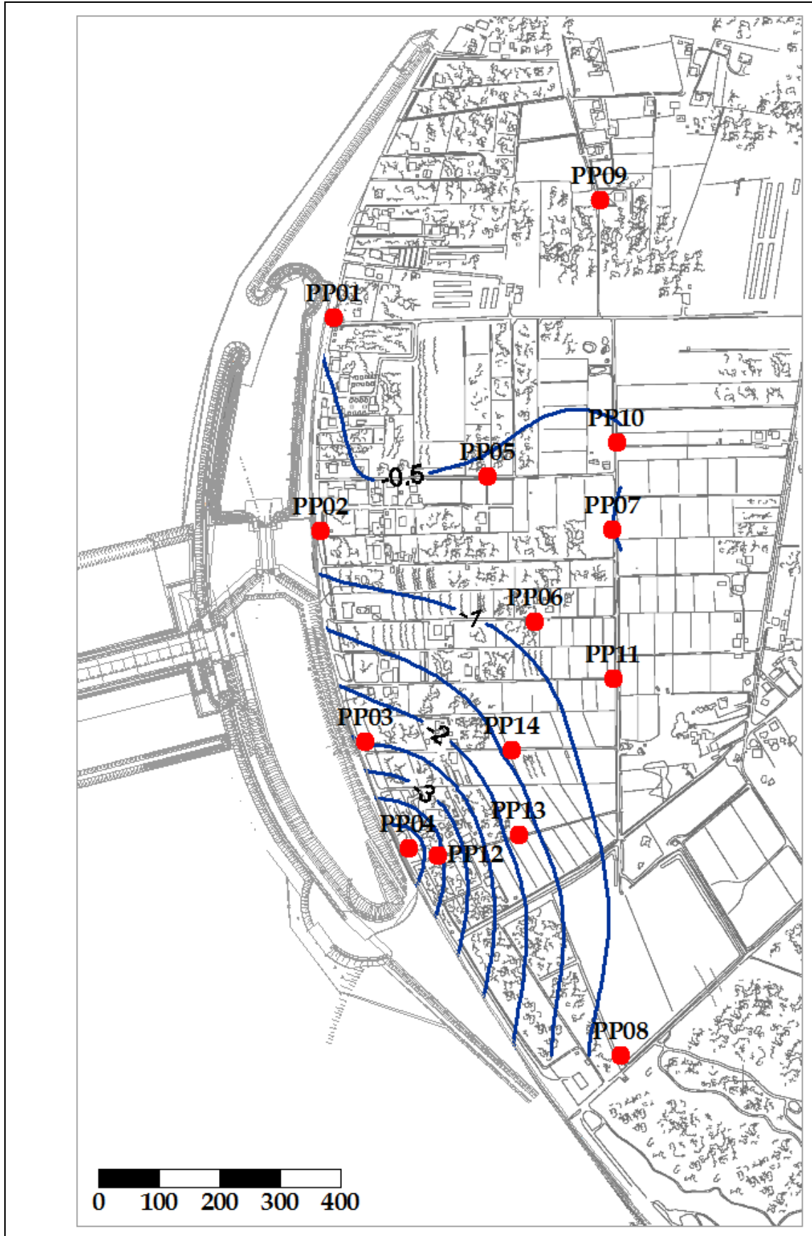
Fig. 5.9 - Piezometria profonda - settembre 2011 ( h_U - m s.l.m.).
