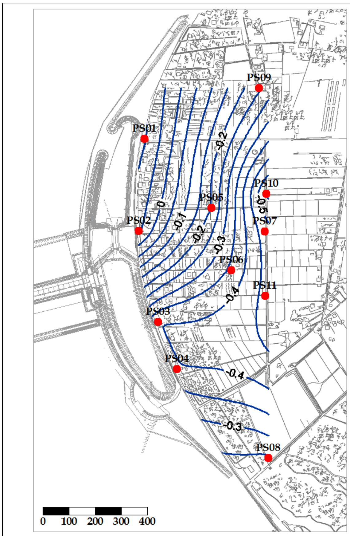
Fig. 5.4 - Piezometria superficiale - settembre 2011 ( h_{d1} - m s.l.m.).
