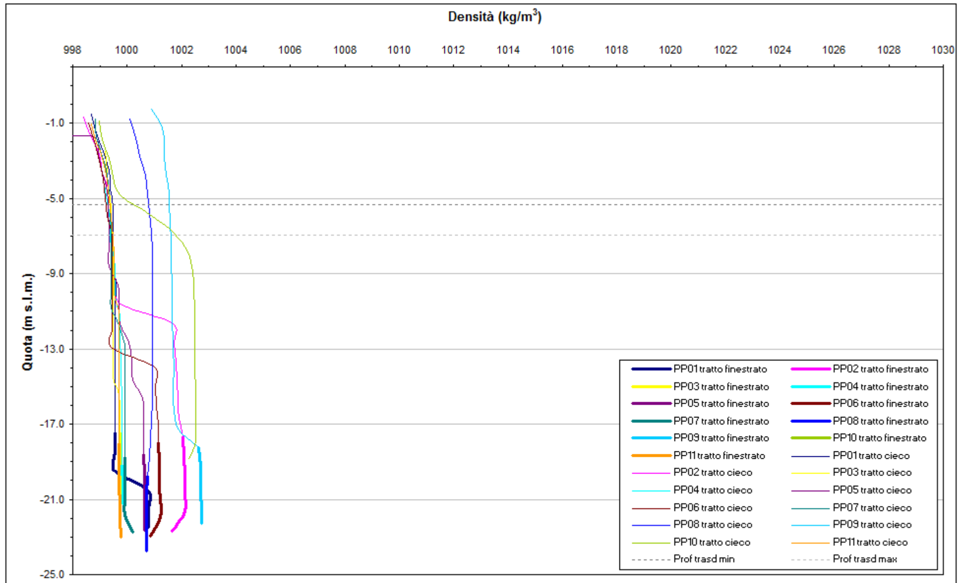
Fig. 4.5 - Profili verticali di densità piezometri profondi - 6 ottobre 2011.
