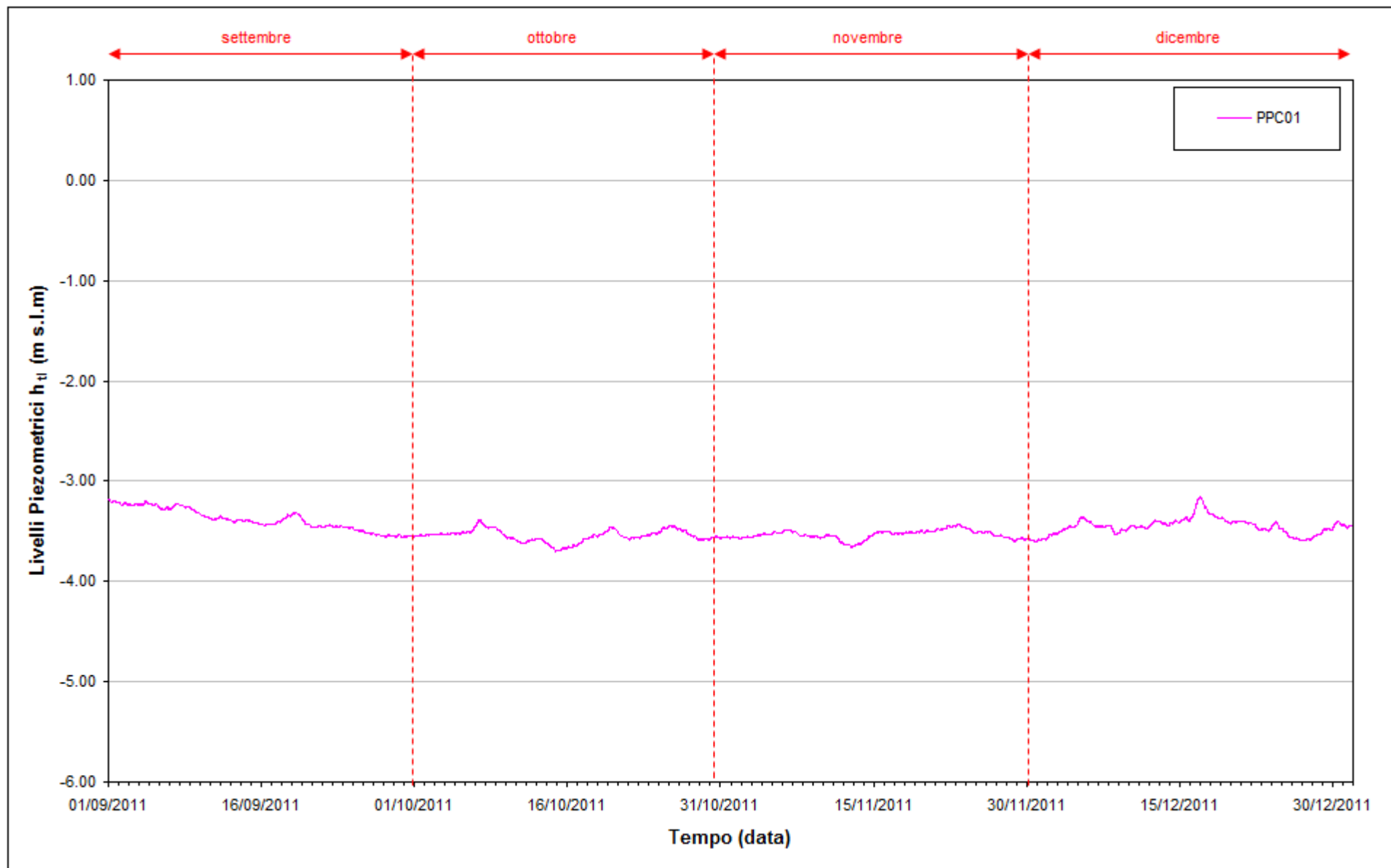
Fig. 9.10 - Livelli piezometrici ( h_U ) relativi al piezometro profondo.
