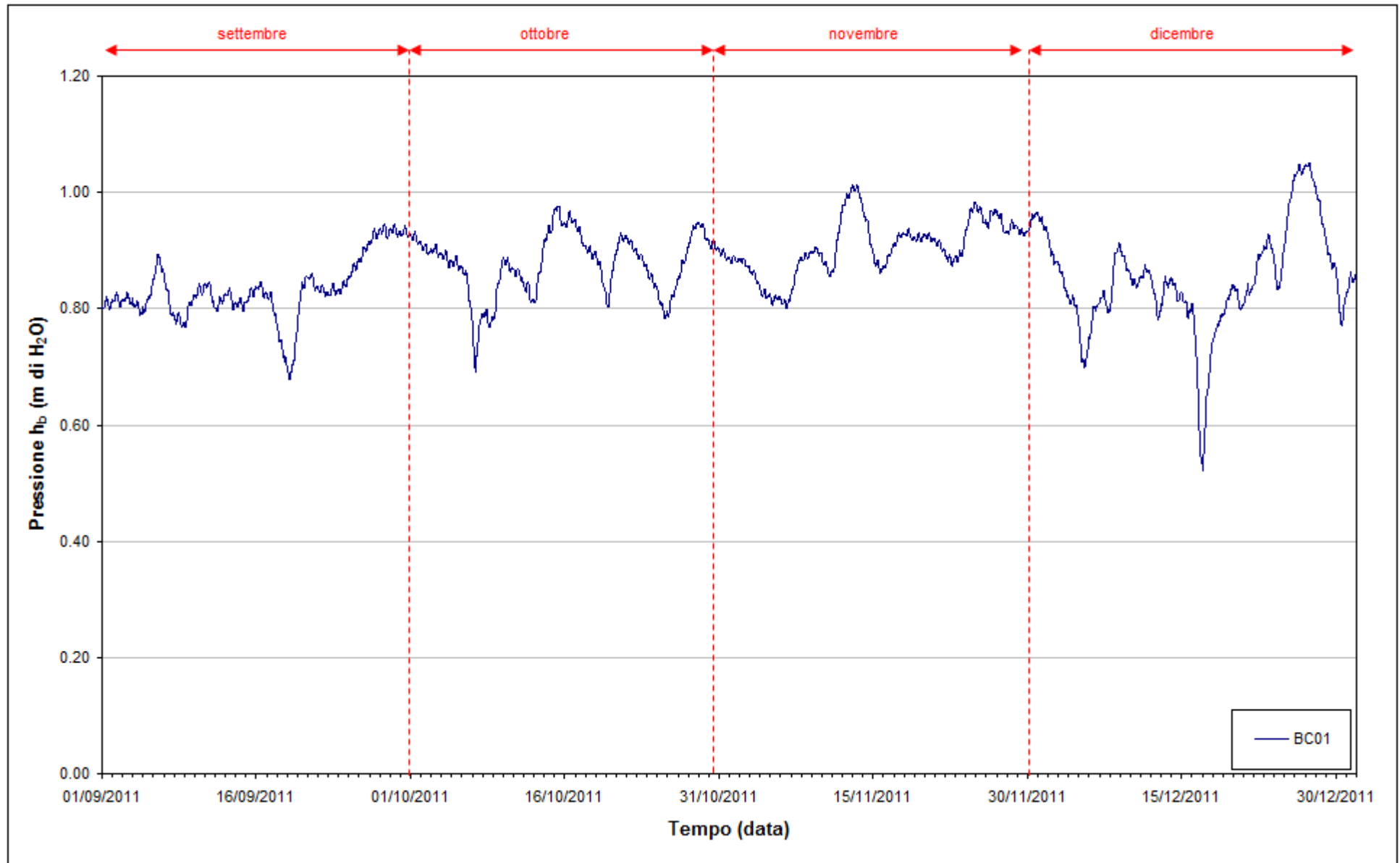
Fig. 9.4- Tracciato di misura del Barologger BC01 (h b ).
