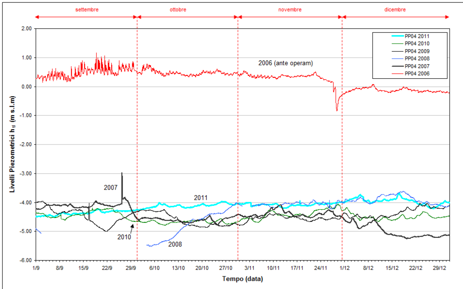
Fig. 2.15 - Confronto tra i livelli piezometrici ( h_u ) nel piezometro PP04 nel periodo settembre - dicembre degli anni 2006÷2011.
