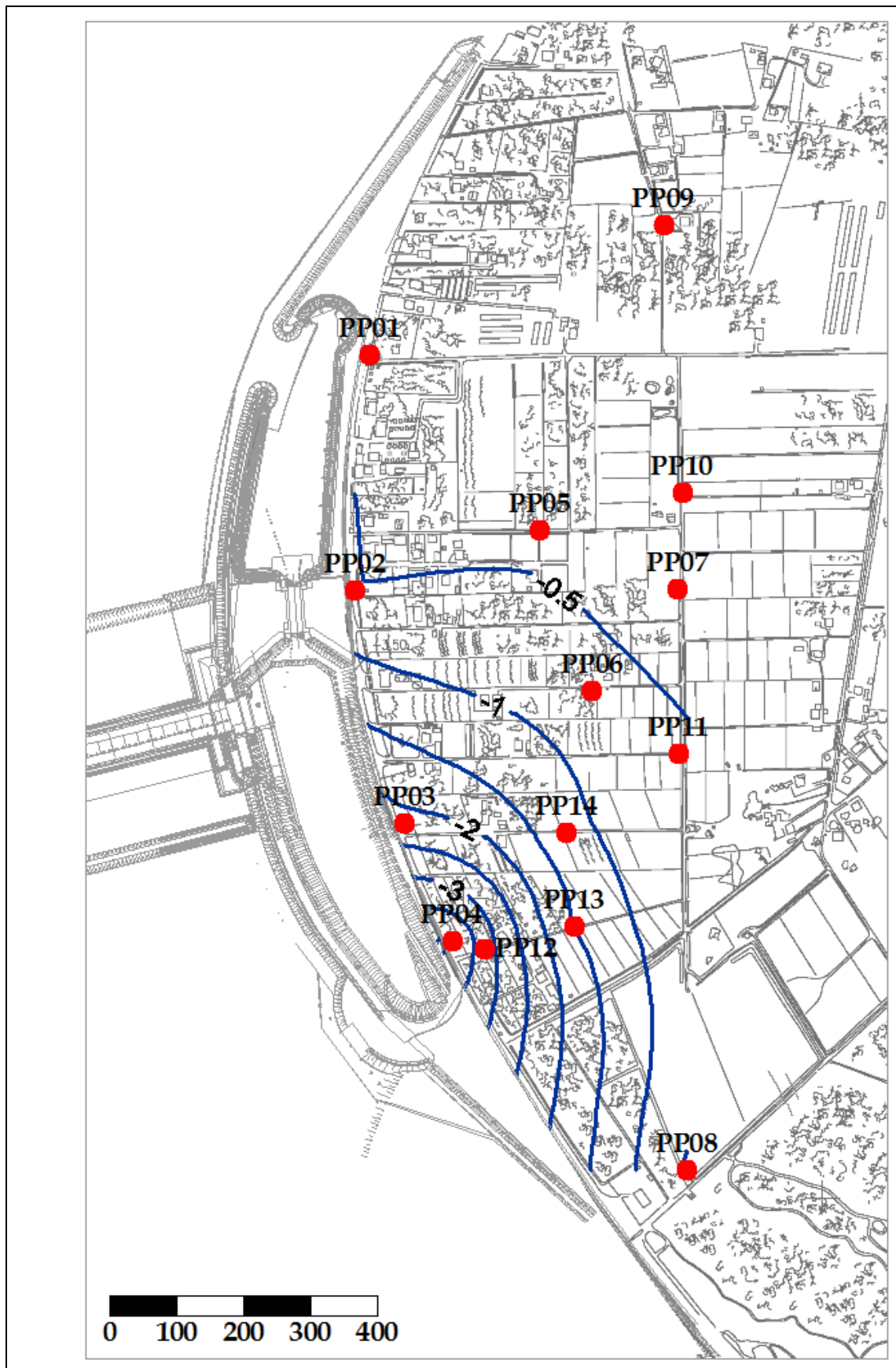
Fig. 5.12 - Piezometria profonda - dicembre 2011 ( h_{hl} - m s.l.m.).
