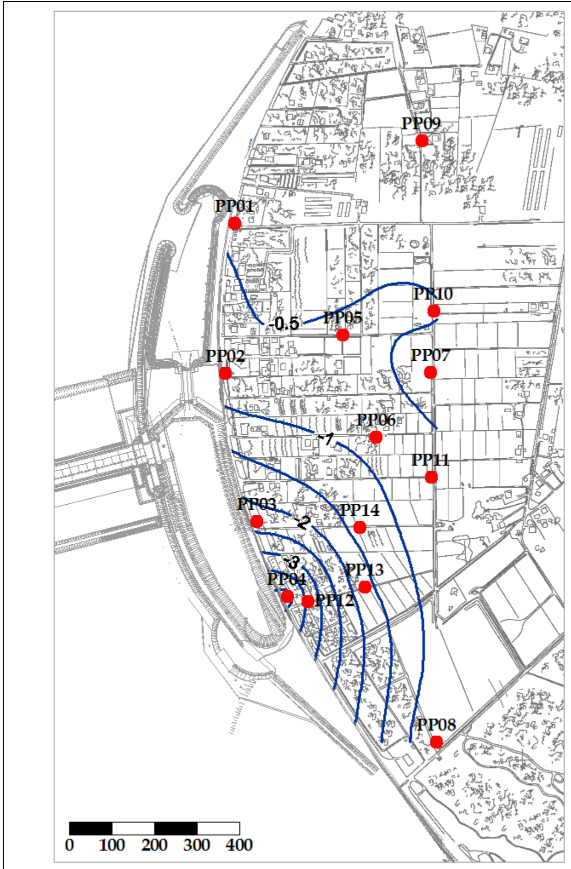
Fig. 5.11 - Piezometria profonda - novembre 2011 ( h_{tl} - m s.l.m.).
