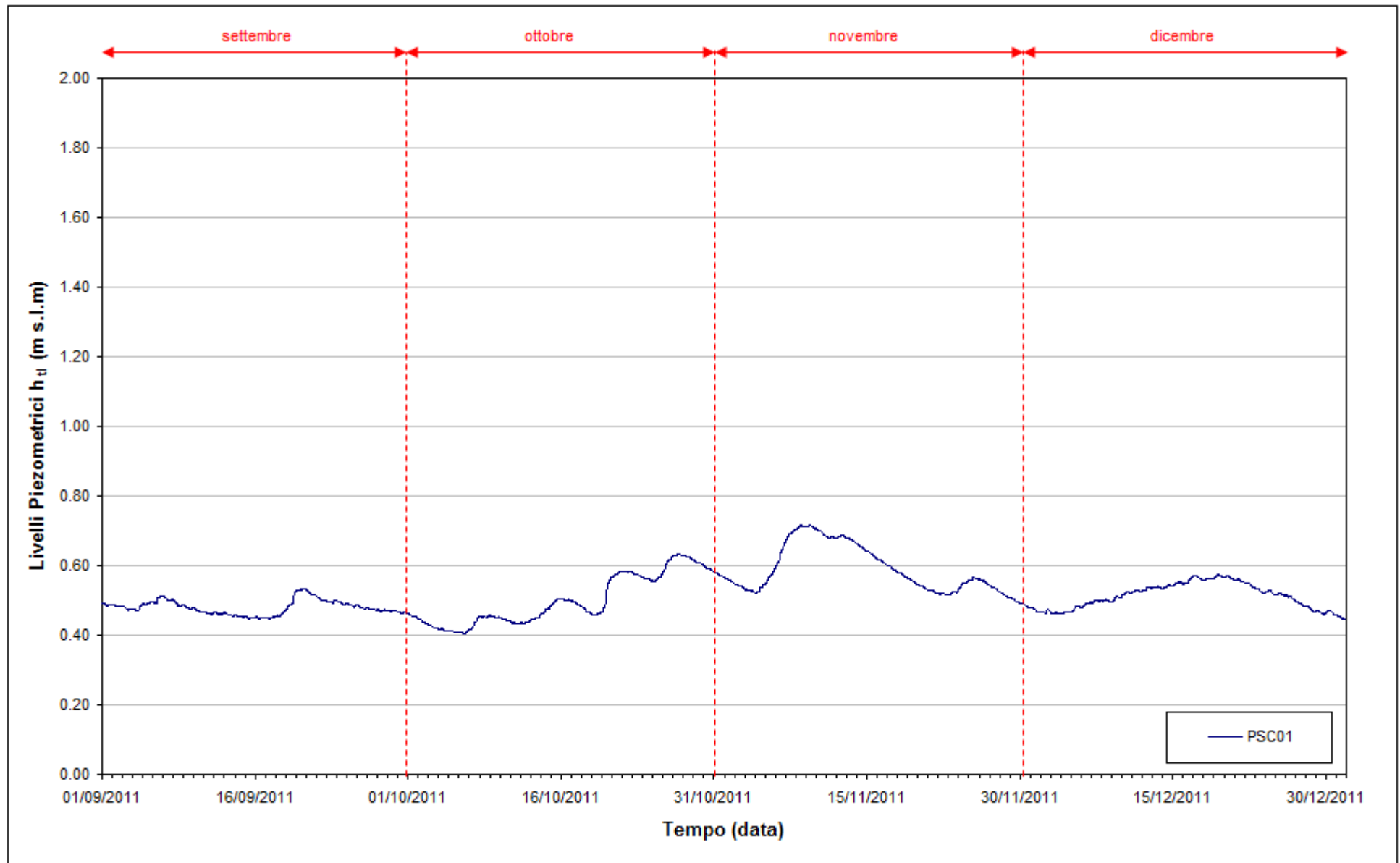
Fig. 9.6- Livelli piezometrici ( h_{11} ) relativi al piezometro superficiale nel quadrimestre di monitoraggio.
