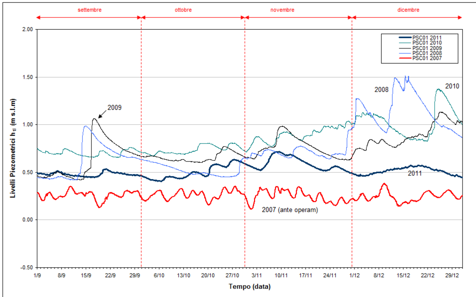
Fig. 9.8 - Confronto tra i livelli piezometrici ( h_u ) nel piezometro PSC01 nel periodo settembre - dicembre degli anni 2007+2011.
