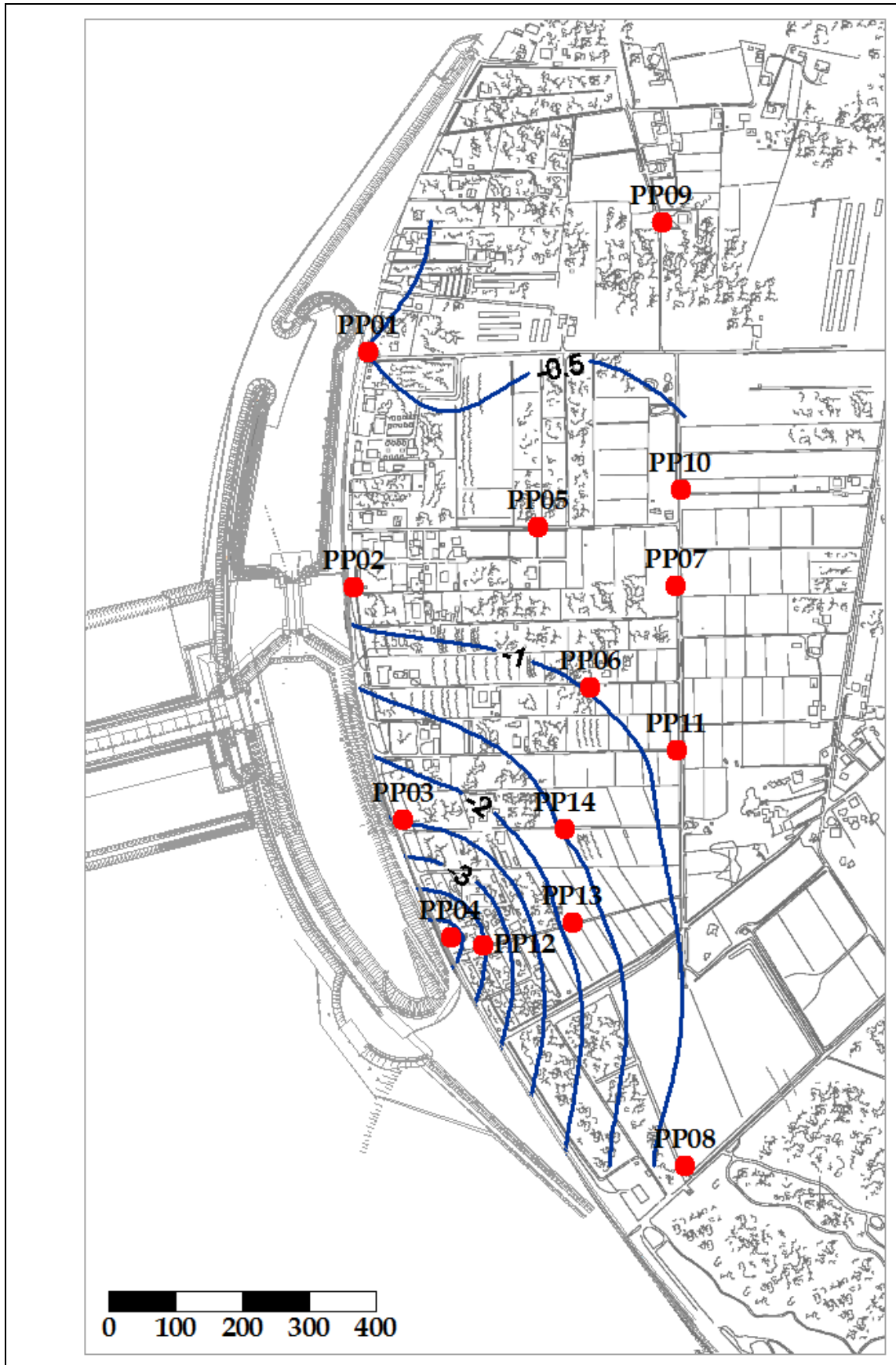
Fig. 5.10 - Piezometria profonda - ottobre 2011 ( h_{PI} - m s.l.m.).
