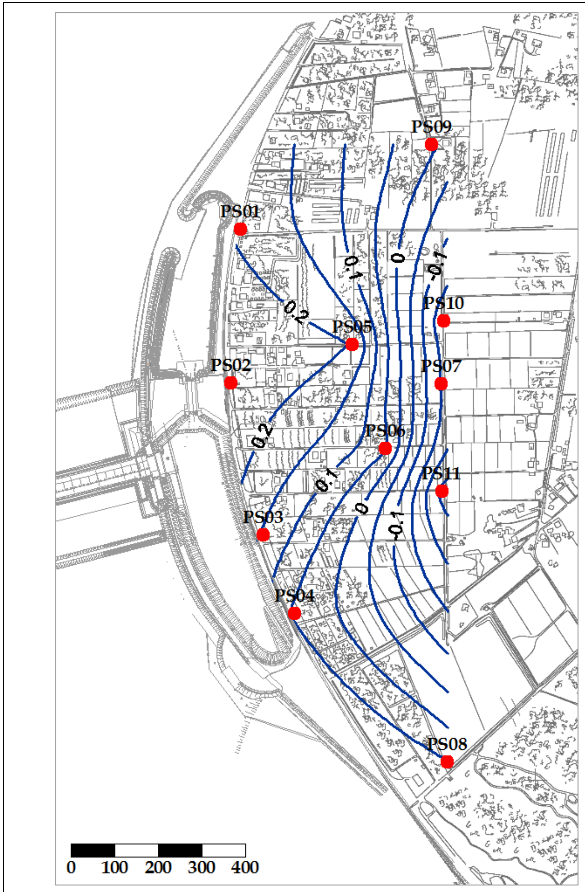
Fig. 5.6 - Piezometria superficiale - novembre 2011 ( h_{fl} - m s.l.m.).
