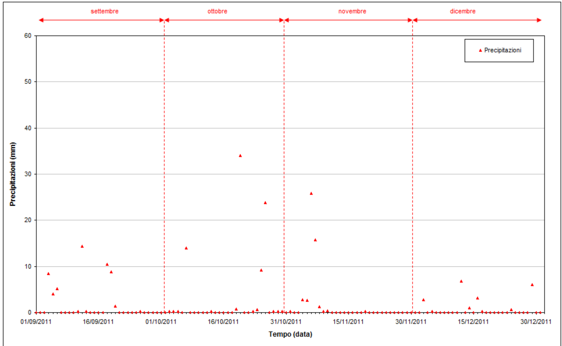
Fig. 2.2 - Precipitazioni registrate nel periodo di monitoraggio 01/09/2011 - 31/12/2011.
