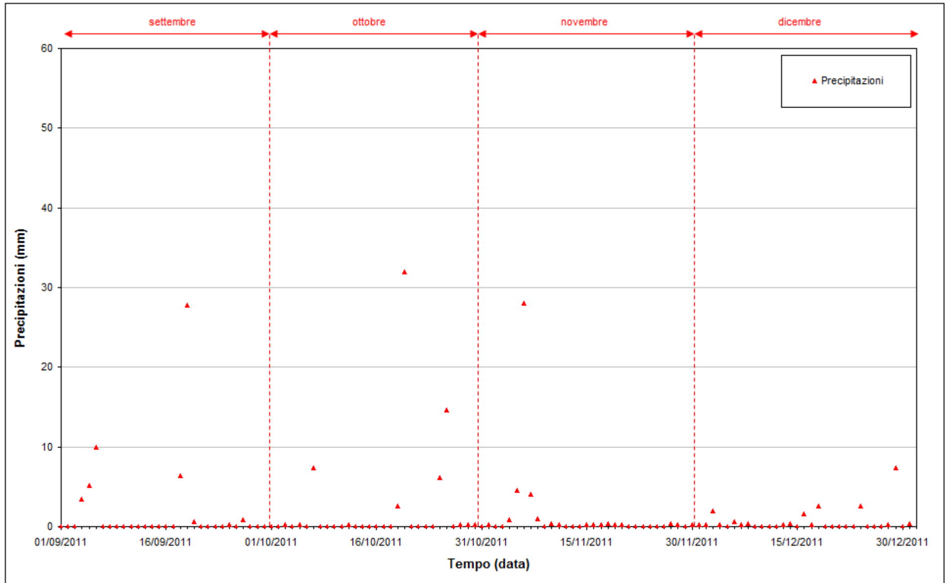
Fig. 9.2 - Precipitazioni registrate nel periodo di monitoraggio 01/09/2011 - 31/12/2011.
