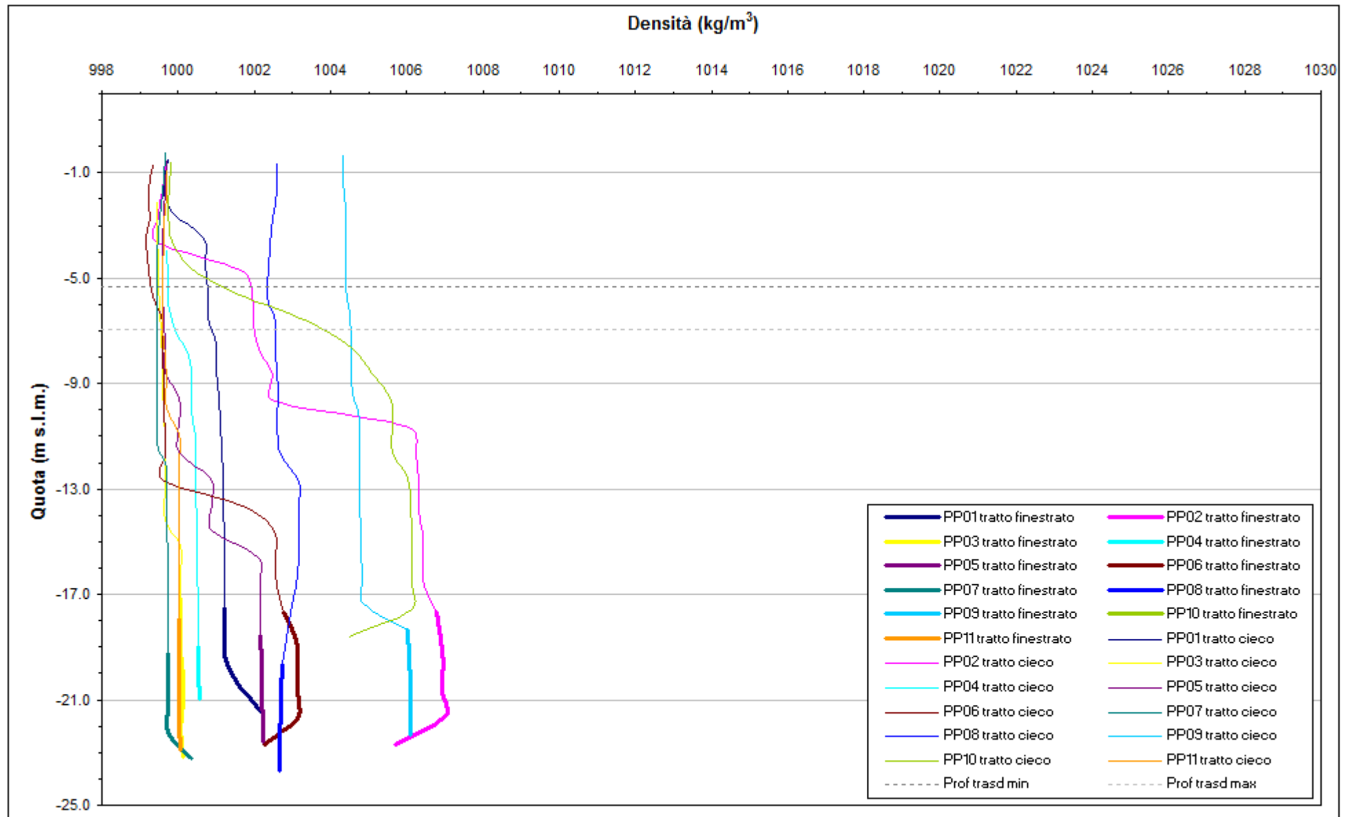
Fig. 4.8 - Profili verticali di densità piezometri profondi - 4-5 gennaio 2012.
