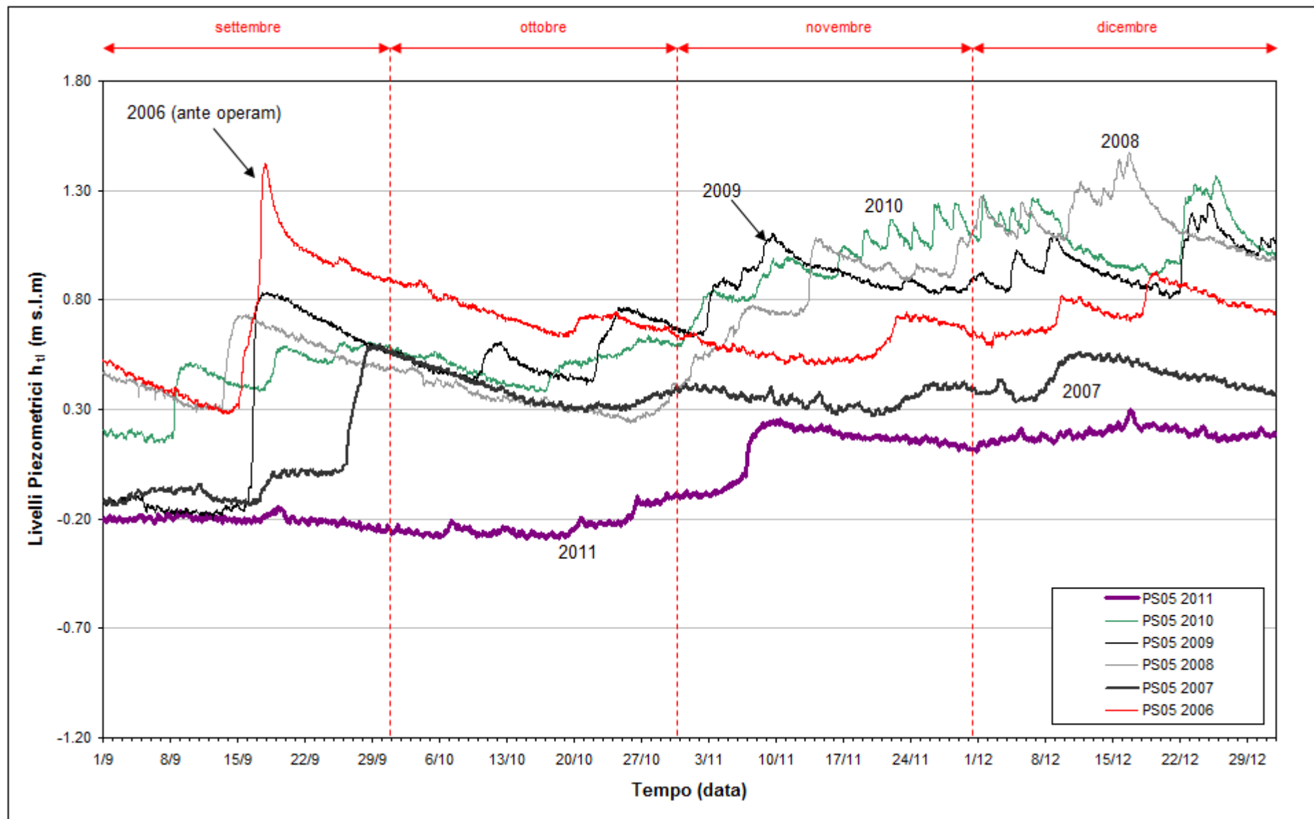
Fig. 2.8 - Confronto tra i livelli piezometrici ( h_t ) nel piezometro PS05 nel periodo settembre - dicembre degli anni 2006÷2011.
