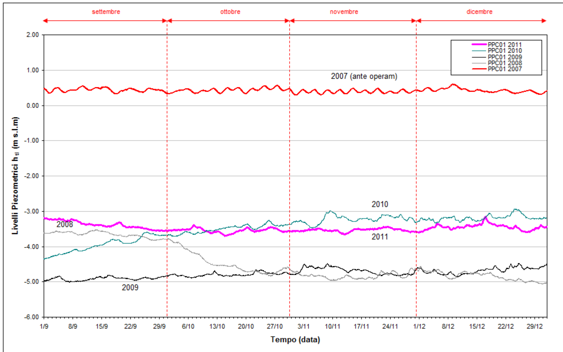
Fig. 9.12 - Confronto tra i livelli piezometrici ( h_u ) nel piezometro PPC01 nel periodo gennaio - aprile degli anni 2007-2011.
