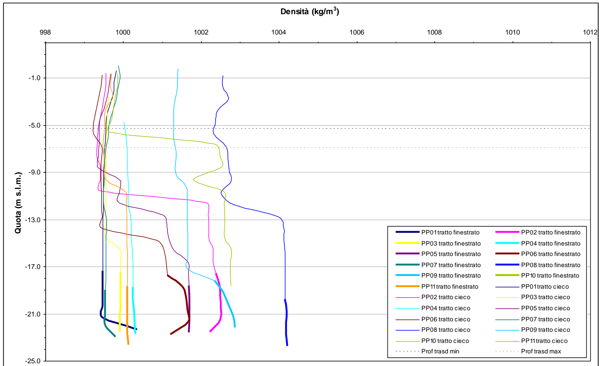
Fig. 4.6- Profili verticali di densità piezometri profondi - 4 marzo 2011.
