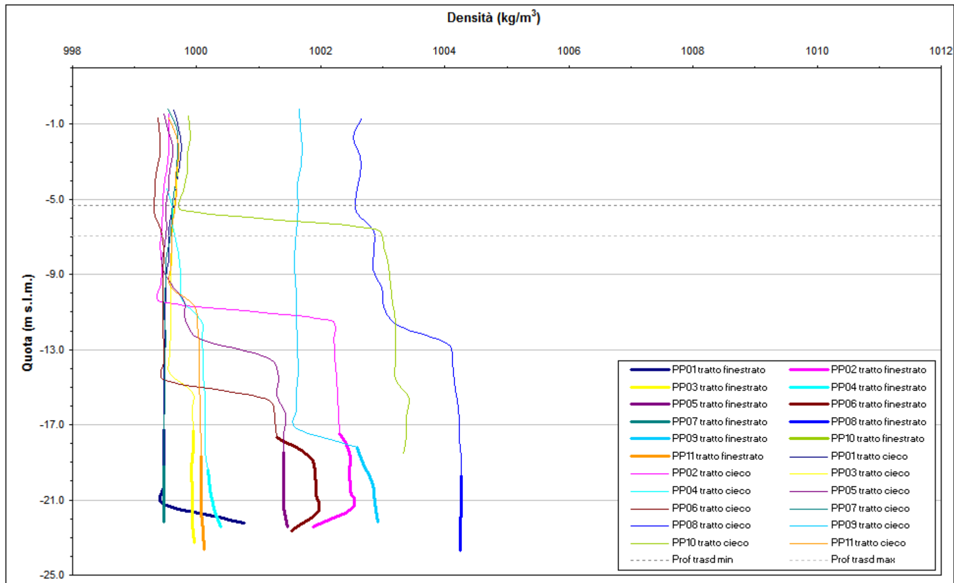
Fig. 4.8 - Profili verticali di densità piezometri profondi - 4 maggio 2011.
