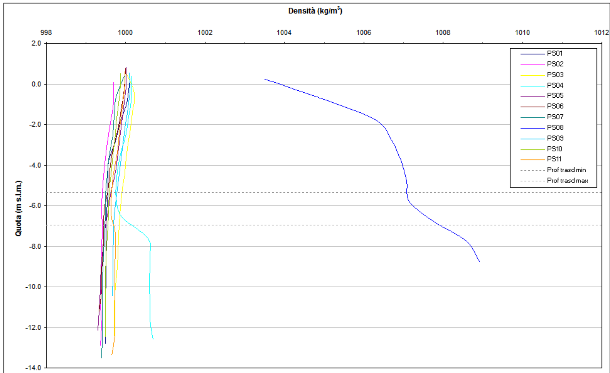
Fig. 4.3 - Profili verticali di densità piezometri superficiali - 5 aprile 2011.
