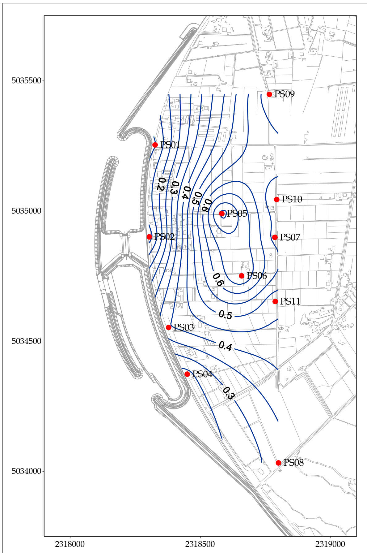
Fig. 5.6 - Piezometria superficiale - marzo 2011 ( h_{tl} - m s.l.m.).
