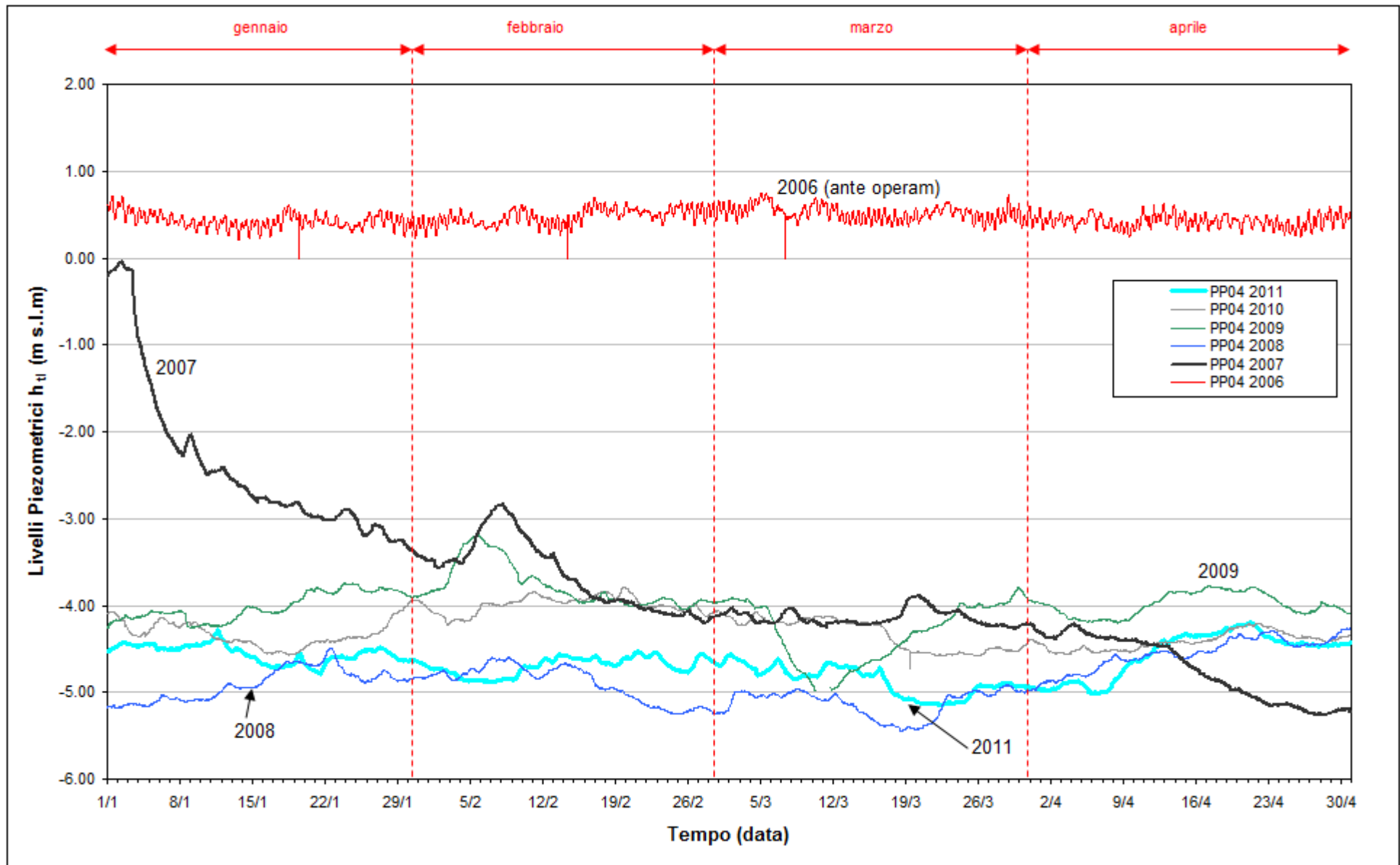
Fig. 2.15 - Confronto tra i livelli piezometrici ( h_u ) nel piezometro PP04 nel periodo gennaio-aprile degli anni 2006÷2011.
