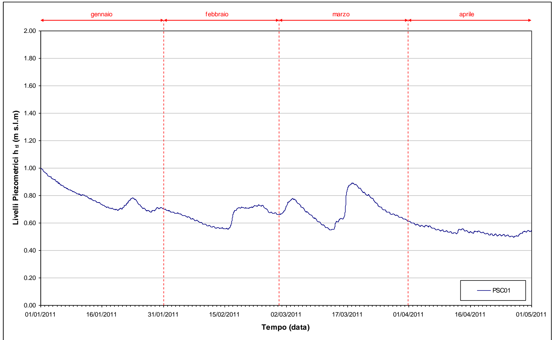
Fig. 9.6- Livelli piezometrici (h u ) relativi al piezometro superficiale nel quadrimestre di monitoraggio.
