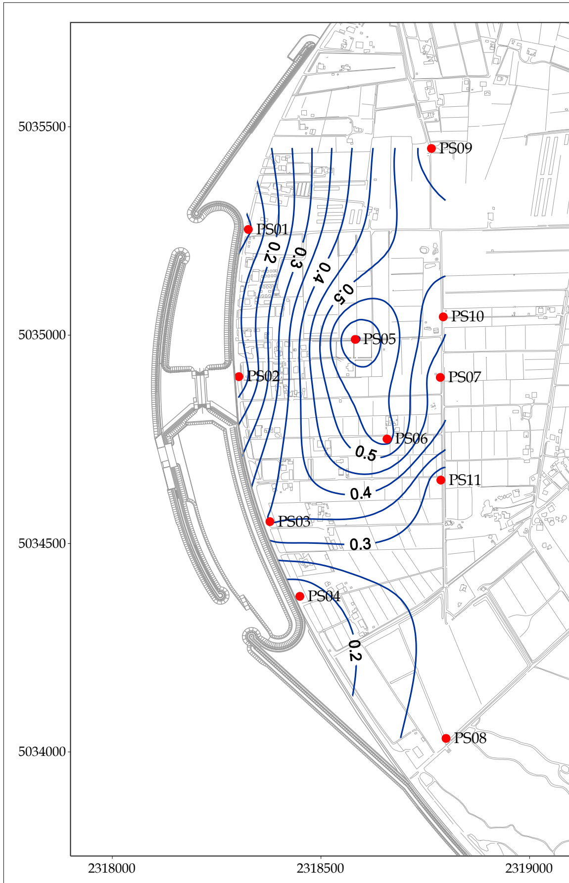
Fig. 5.7 - Piezometria superficiale - aprile 2011 ( h_{hl} - m s.l.m.).
