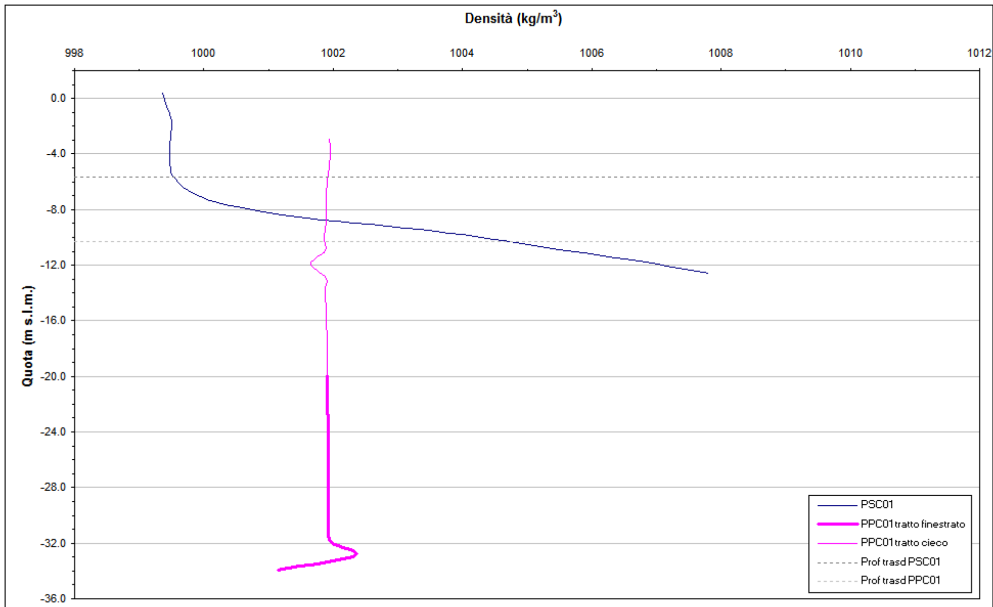
Fig. 11.4.- Profili verticali di densità - 4 maggio 2011.
