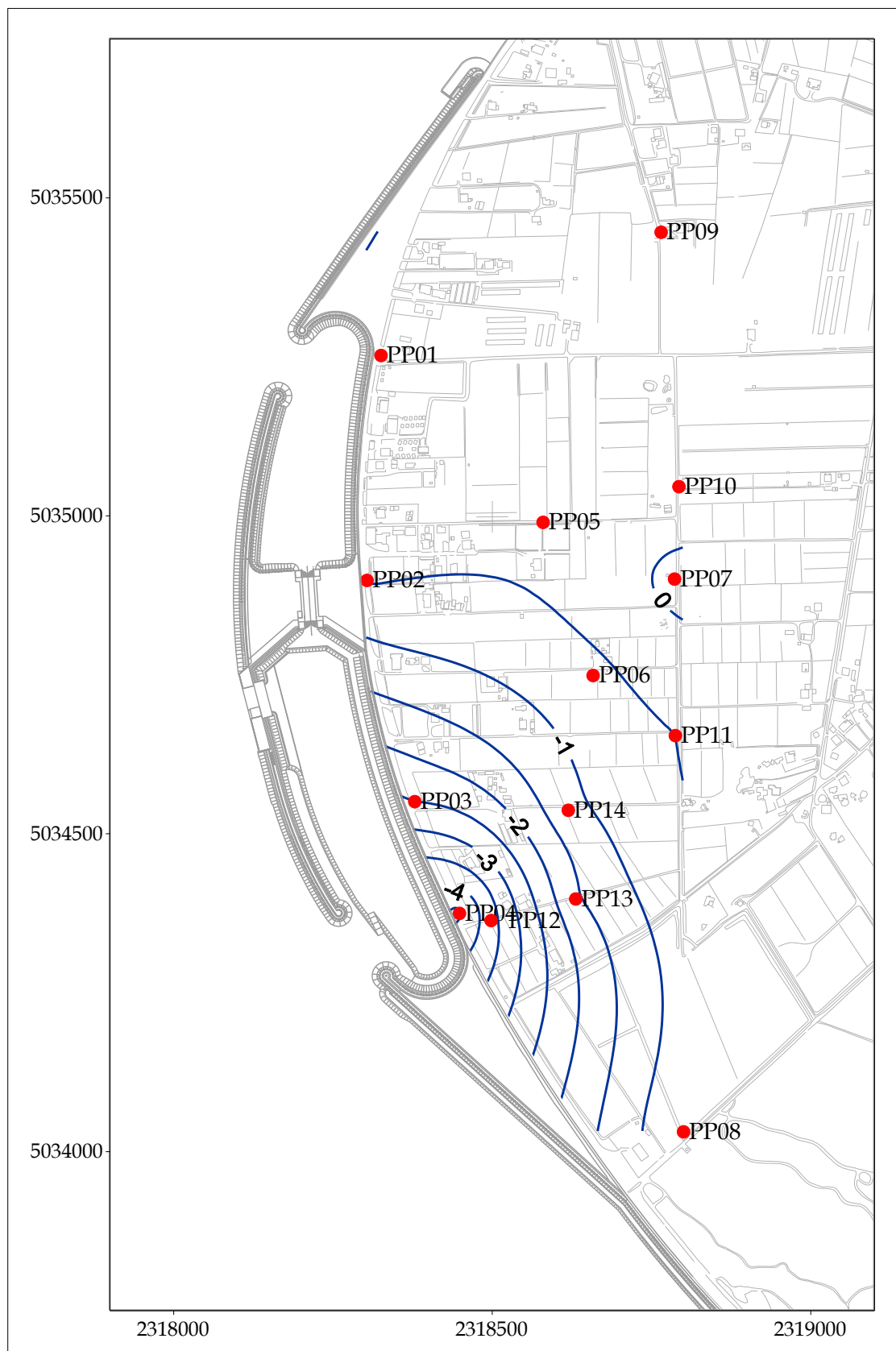
Fig. 5.11 - Piezometria profonda - marzo 2011 ( h_{il} - m s.l.m.).
