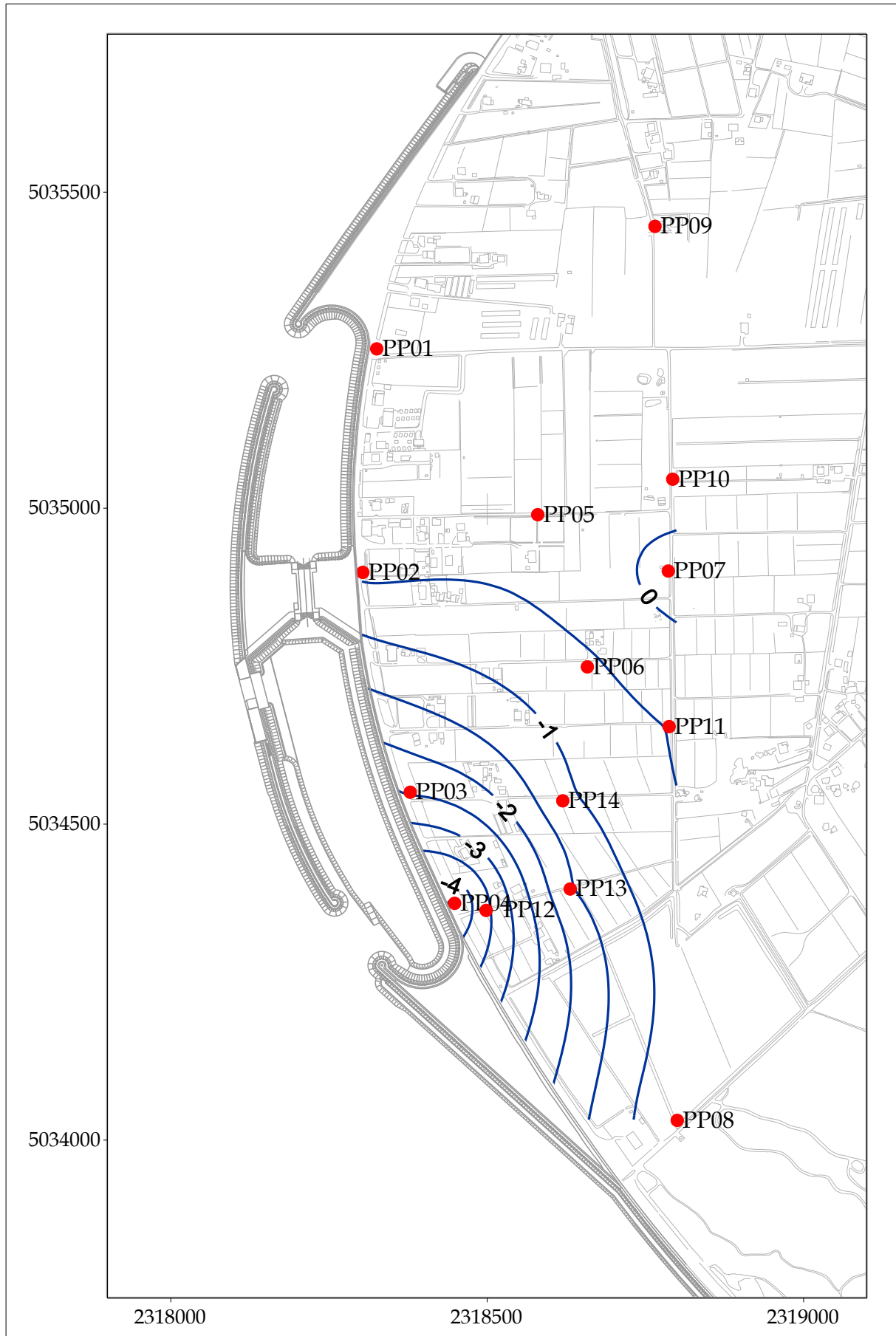
Fig. 5.10 - Piezometria profonda - febbraio 2011 ( h_{PI} - m s.l.m.).
