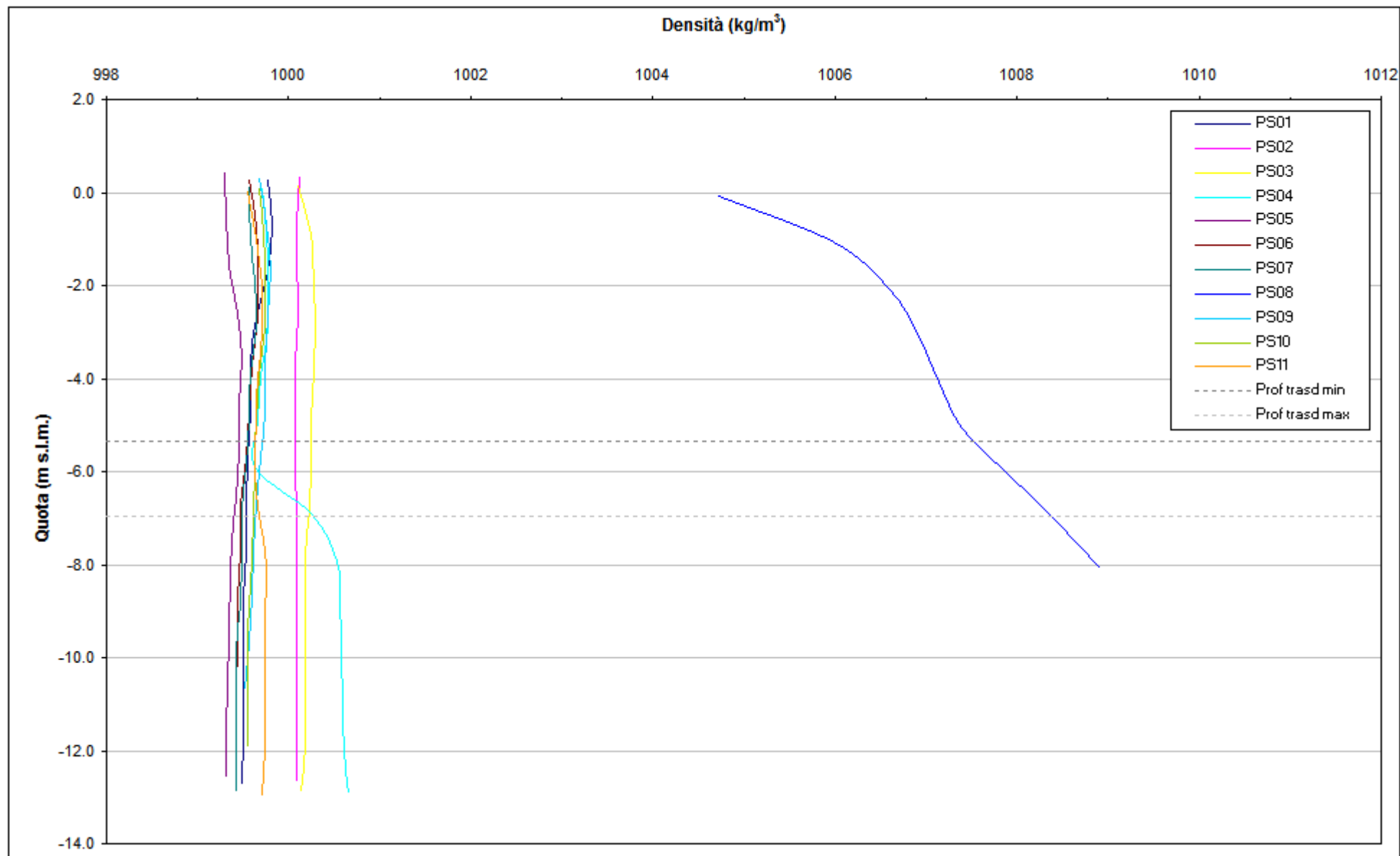
Fig. 4.4 - Profili verticali di densità piezometri superficiali - 4 maggio 2011.
