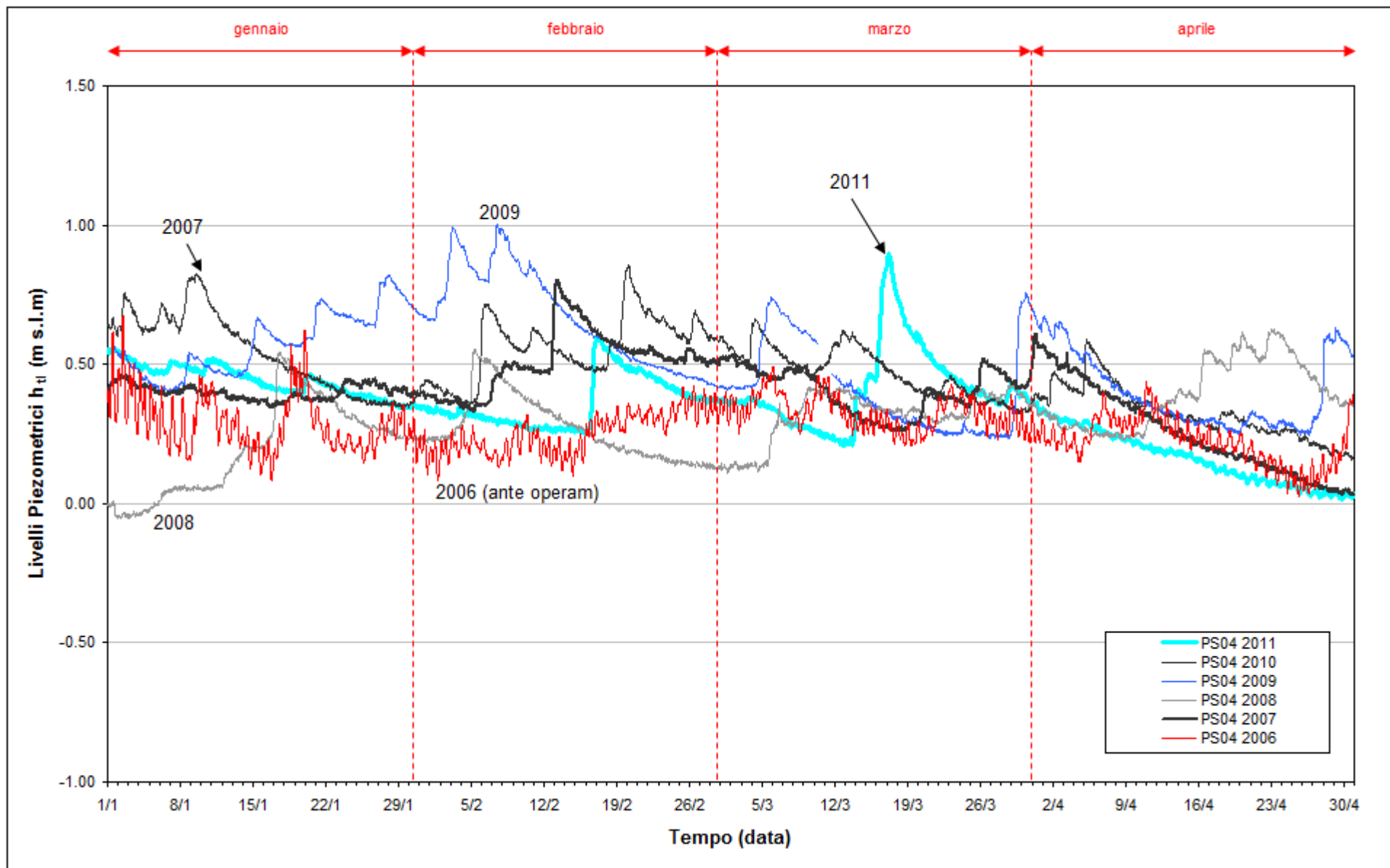
Fig. 2.9 - Confronto tra i livelli piezometrici ( h_t ) nel piezometro PS04 nel periodo gennaio - aprile degli anni 2006÷2011.
