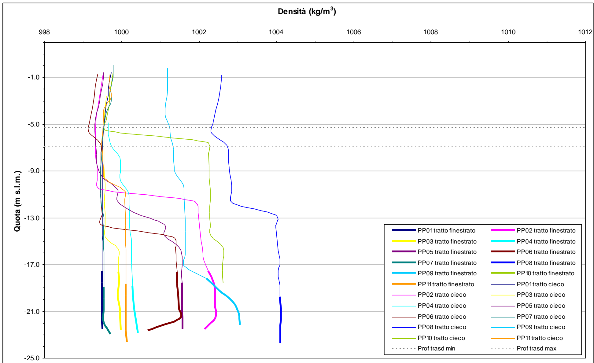
Fig. 4.5 - Profili verticali di densità piezometri profondi - 3-4 febbraio 2011.
