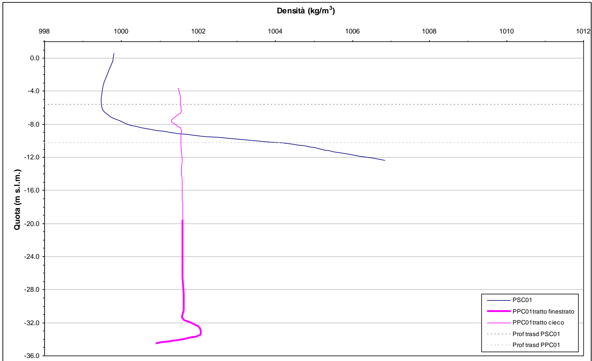
Fig. 11.2.- Profili verticali di densità - 4 marzo 2011.
