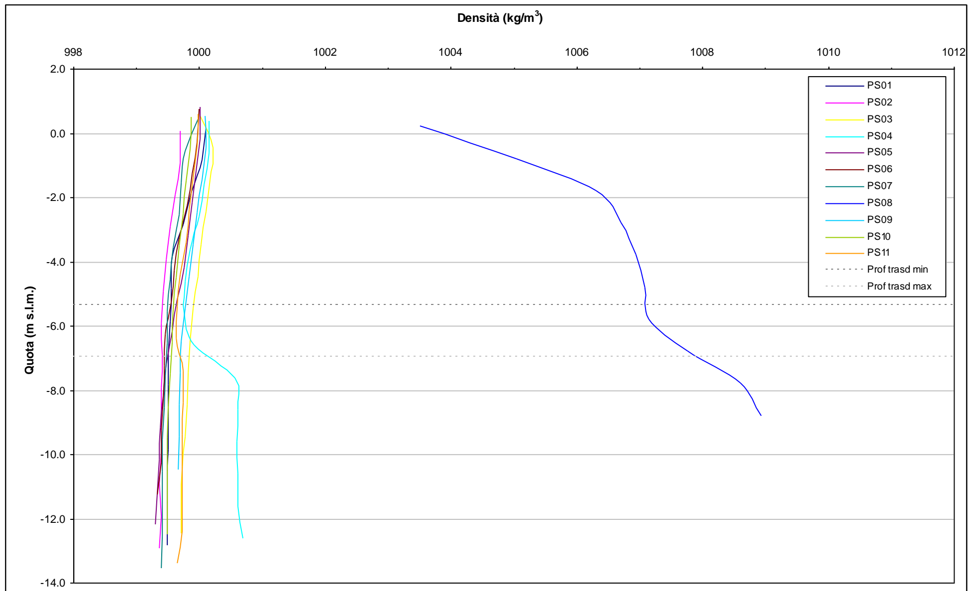
Fig. 4.2- Profili verticali di densità piezometri superficiali - 4 marzo 2011.
