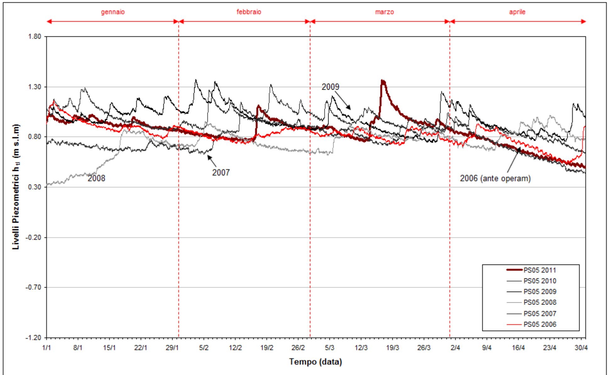
Fig. 2.8 - Confronto tra i livelli piezometrici ( h_t ) nel piezometro PS05 nel periodo gennaio - aprile degli anni 2006÷2011.
