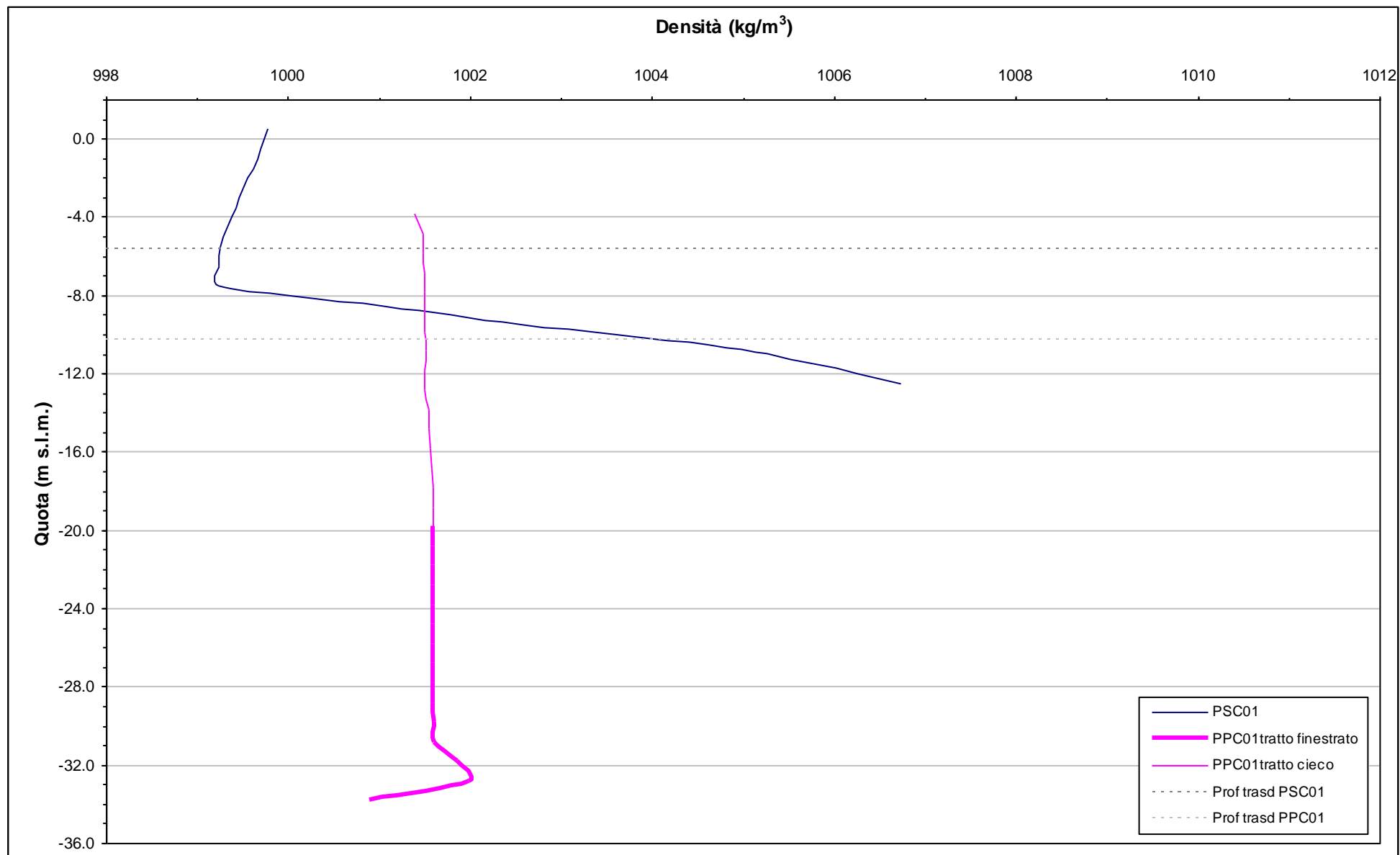
Fig. 11.1 Profili verticali di densità - 4 febbraio 2011.
