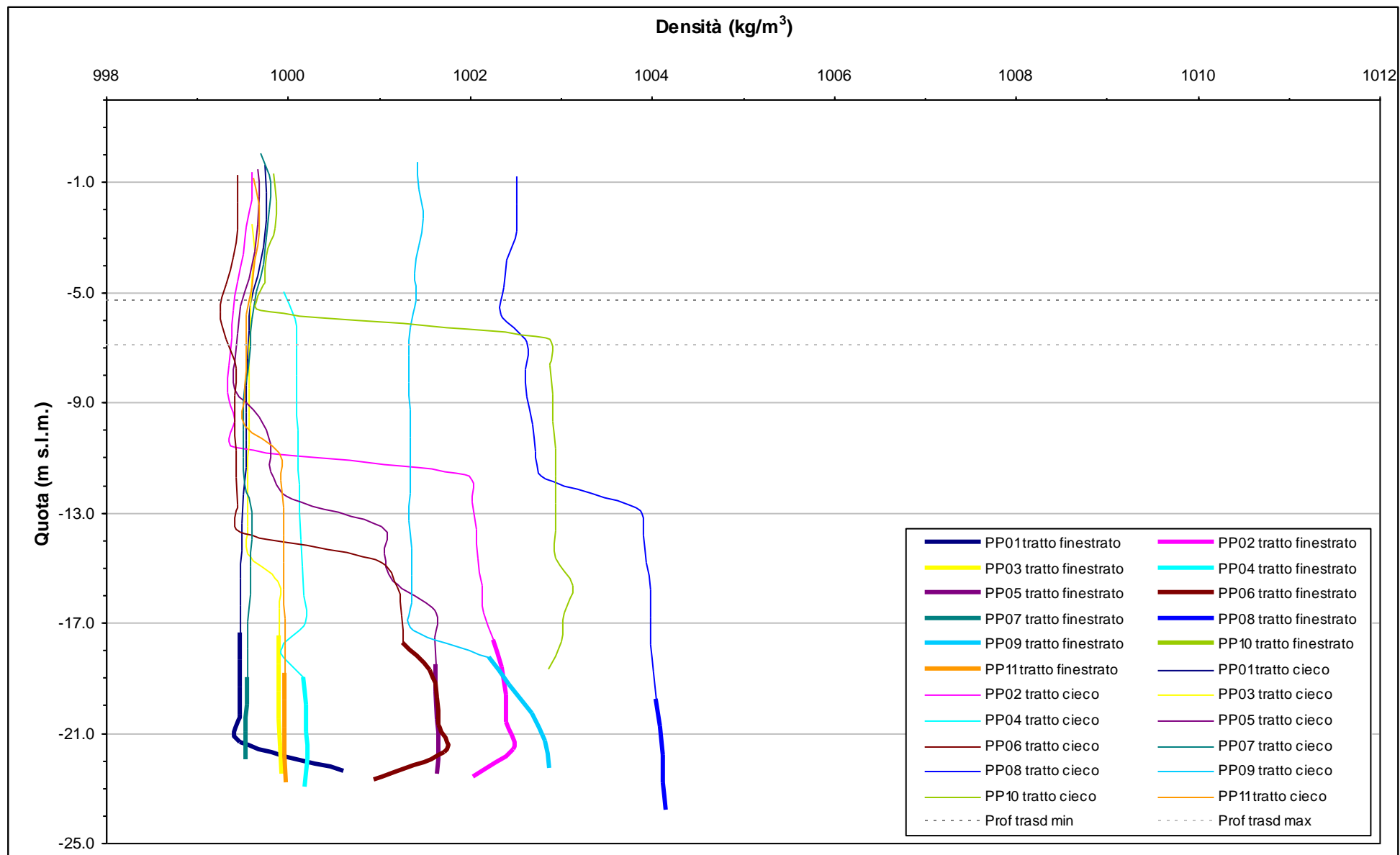
Fig. 4.7 - Profili verticali di densità piezometri profondi - 5 aprile 2011.
