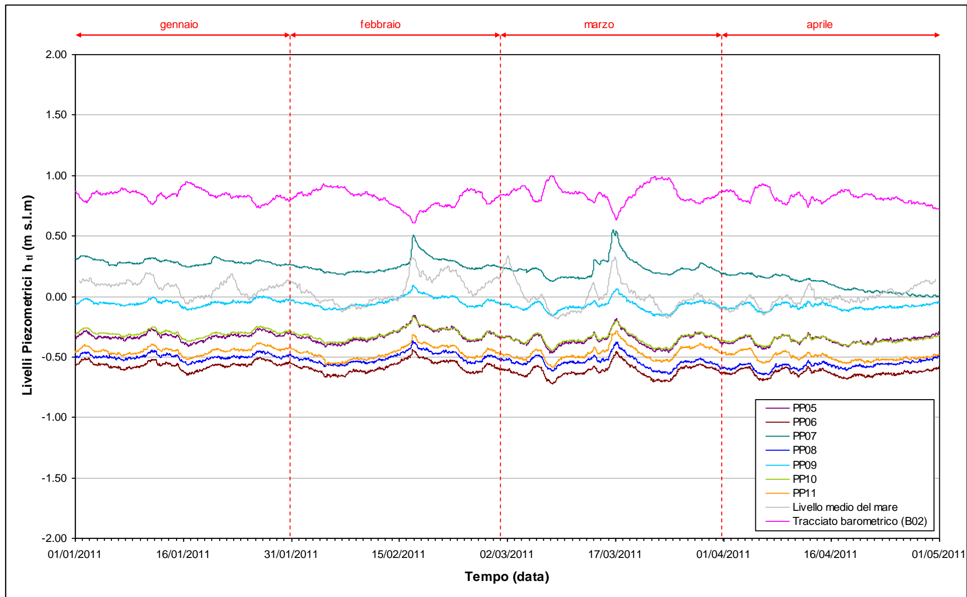
Fig. 2.13 - Livelli piezometrici dei piezometri profondi PP05, PP06, PP07, PP08, PP09, PP10, PP11, livelli medi del mare e tracciati barometrici.
