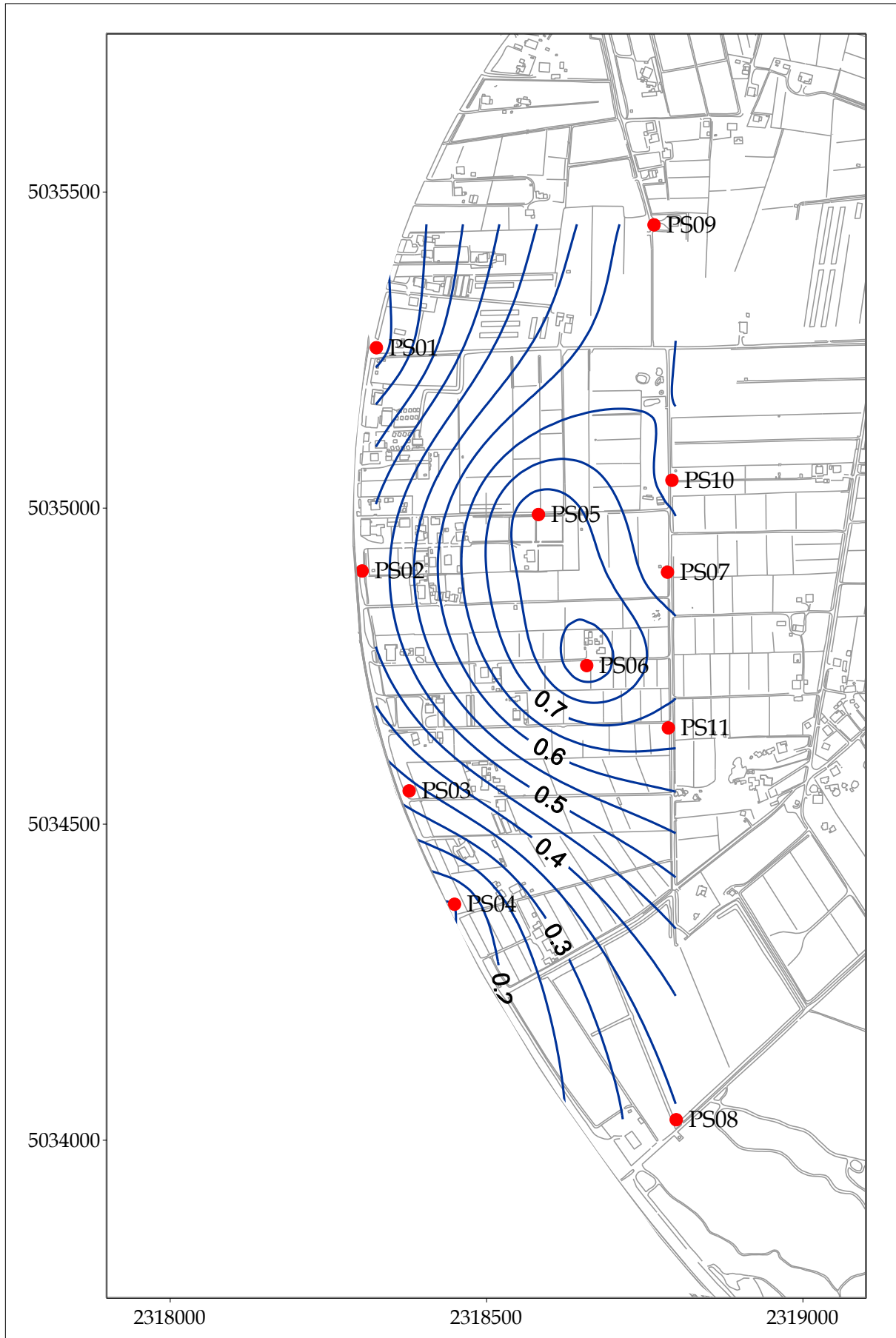
Fig. 5.3 - Piezometri superficiale Fase A - novembre 2005 ( h_d - m s.l.m.).
