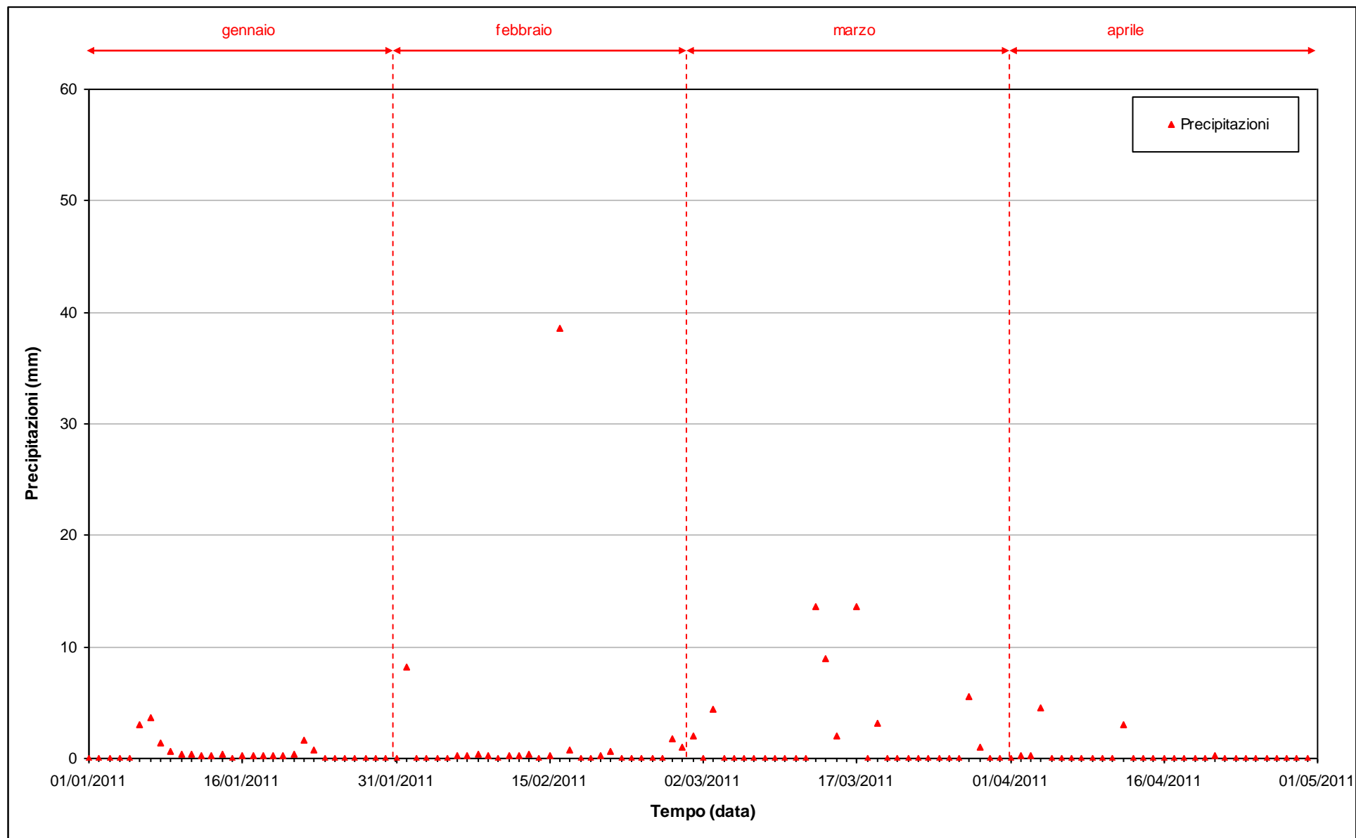
Fig. 2.2 - Precipitazioni registrate nel periodo di monitoraggio 01/01/2011 - 30/04/2011.
