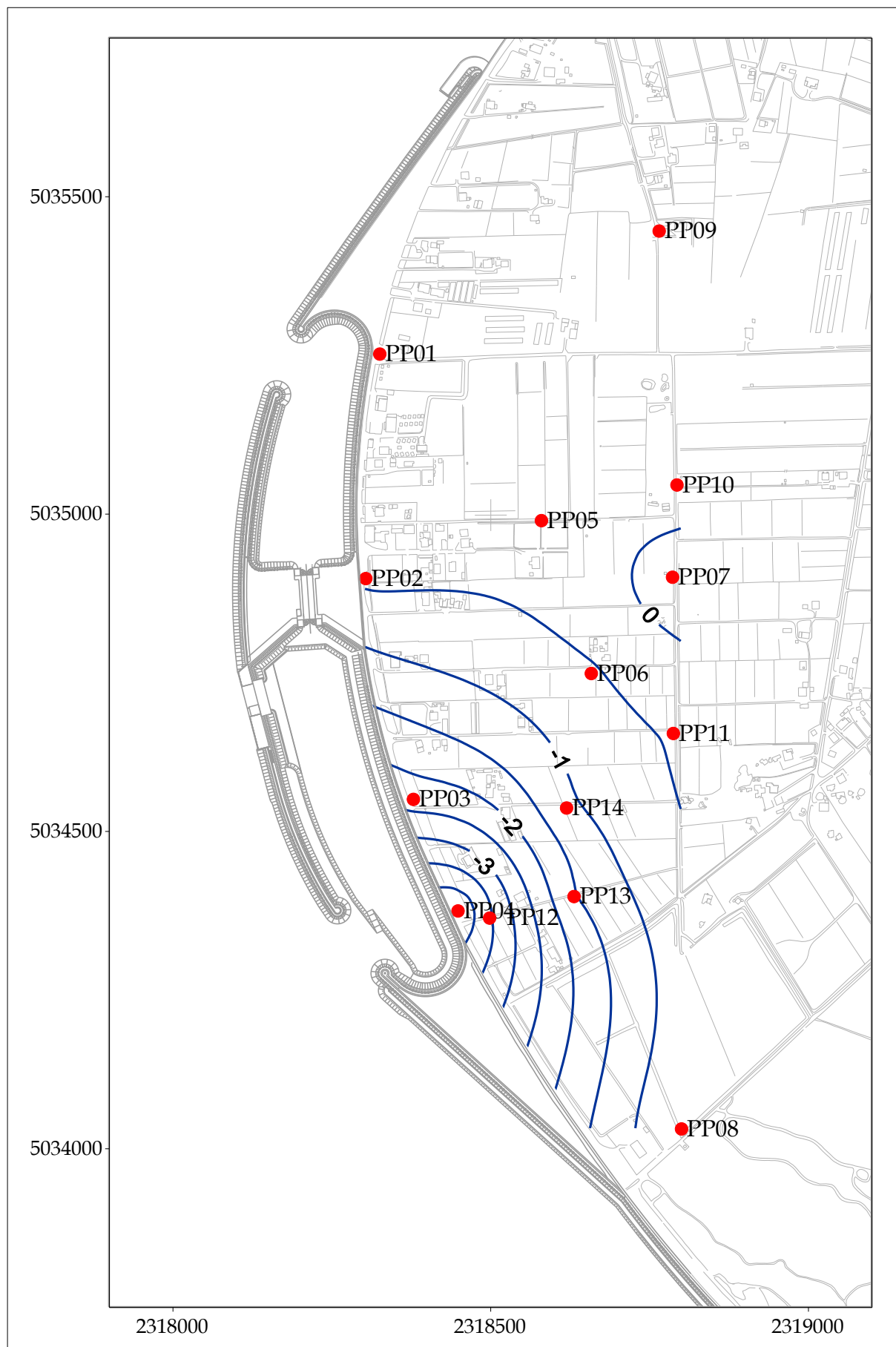
Fig. 5.9 - Piezometria profonda - gennaio 2011 ( h_{PI} - m s.l.m.).
