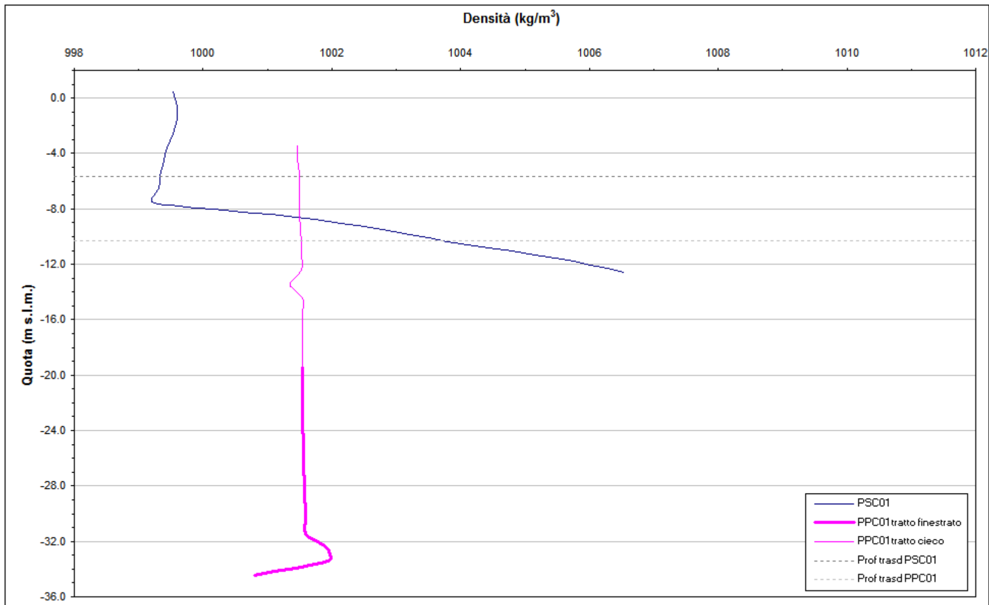
Fig. 11.3.- Profili verticali di densità - 5 aprile 2011.
