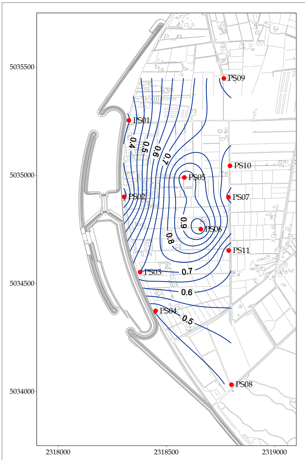
Fig. 5.4 - Piezometria superficiale - gennaio 2011 ( h_{il} - m s.l.m.).
