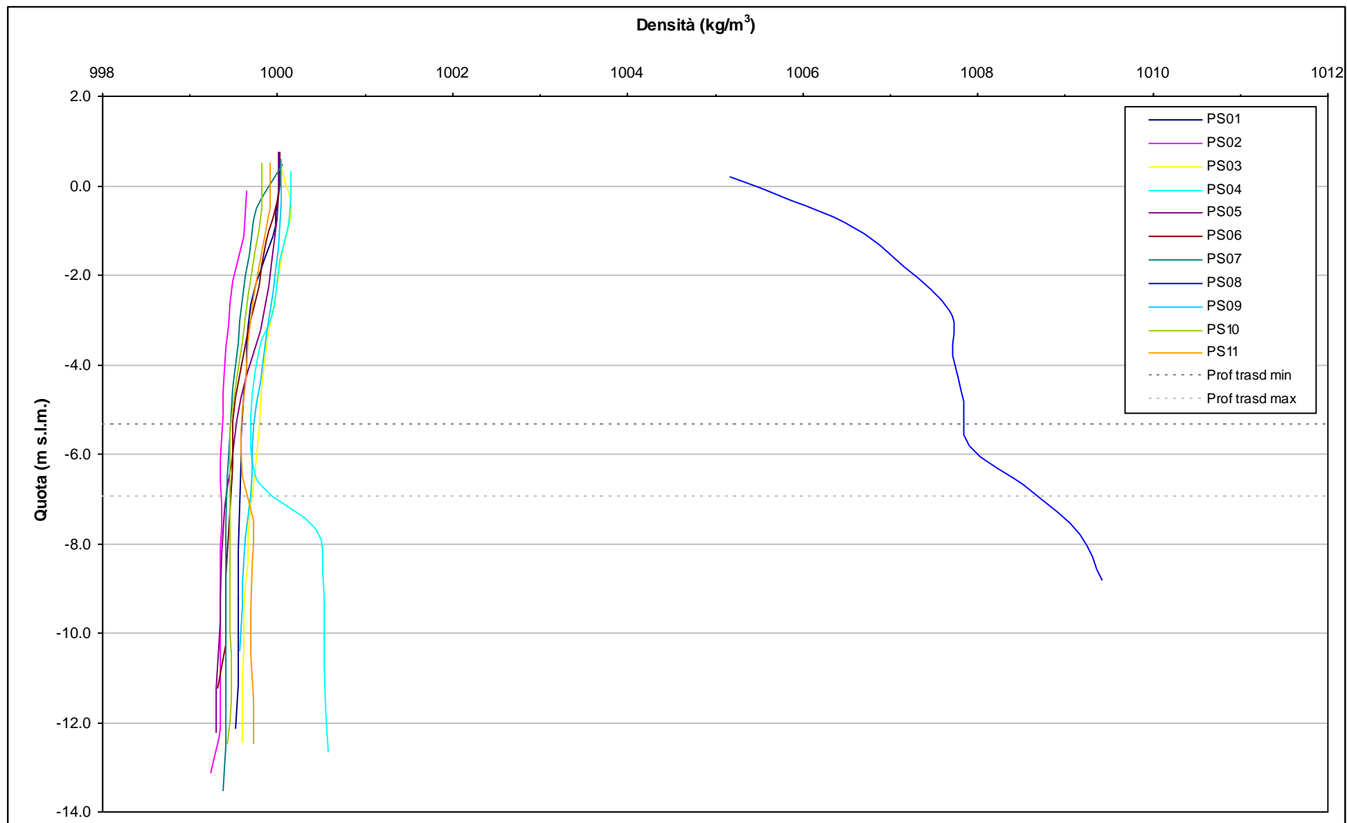
Fig. 4.1- Profili verticali di densità piezometri superficiali - 3-4 febbraio 2011.
