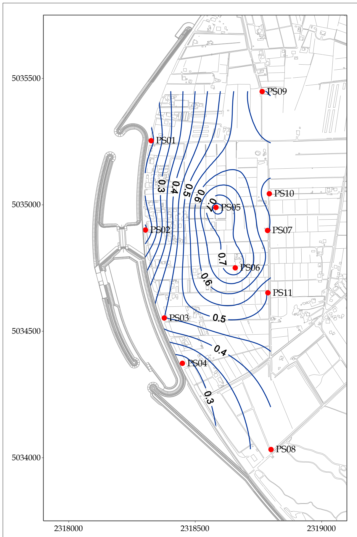
Fig. 5.5- Piezometria superficiale - febbraio 2011 ( h_{el} - m s.l.m.).
