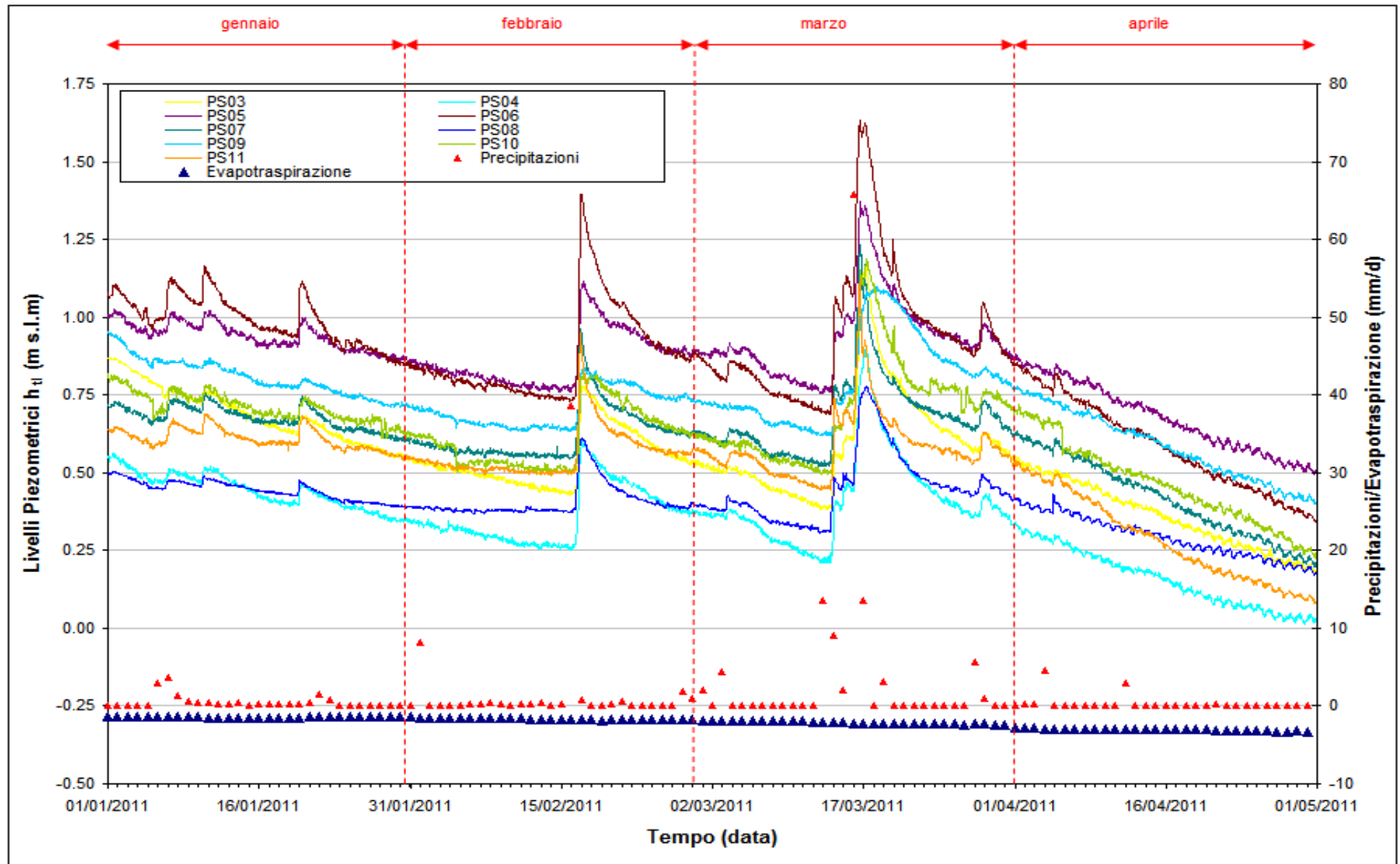
Fig. 2.7 - Livelli piezometrici dei piezometri superficiali maggiormente sensibili alle precipitazioni e all'evapotraspirazione.
