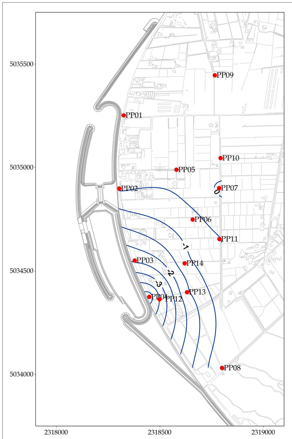
Fig. 5.12 - Piezometria profonda - aprile 2011 ( h_{tl} - m s.l.m.).
