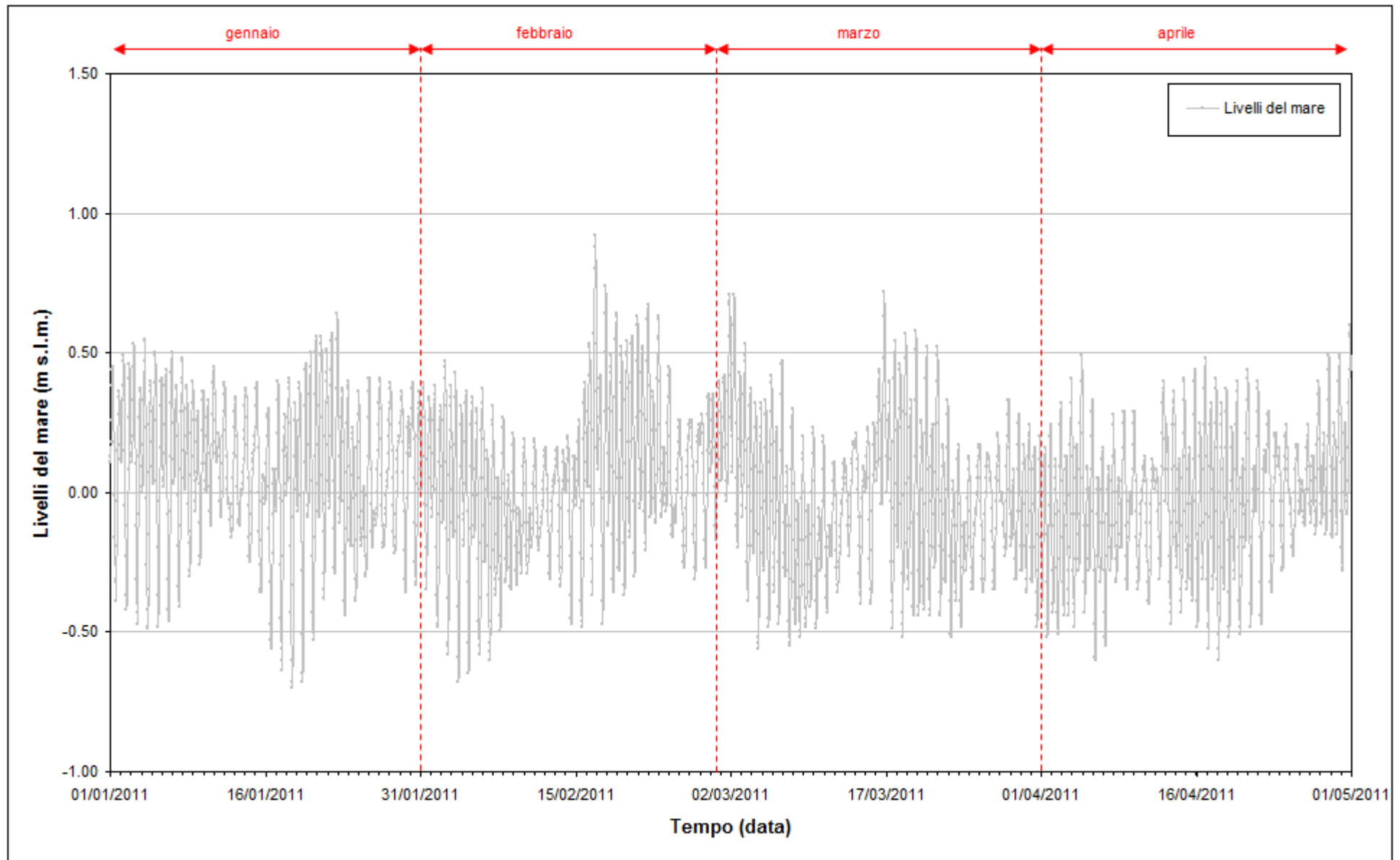
Fig. 9.3 - Livello del mare misurato in corrispondenza del mareografo Chioggia Città. I livelli sono riferiti al sistema IGM - "Genova 1942".
