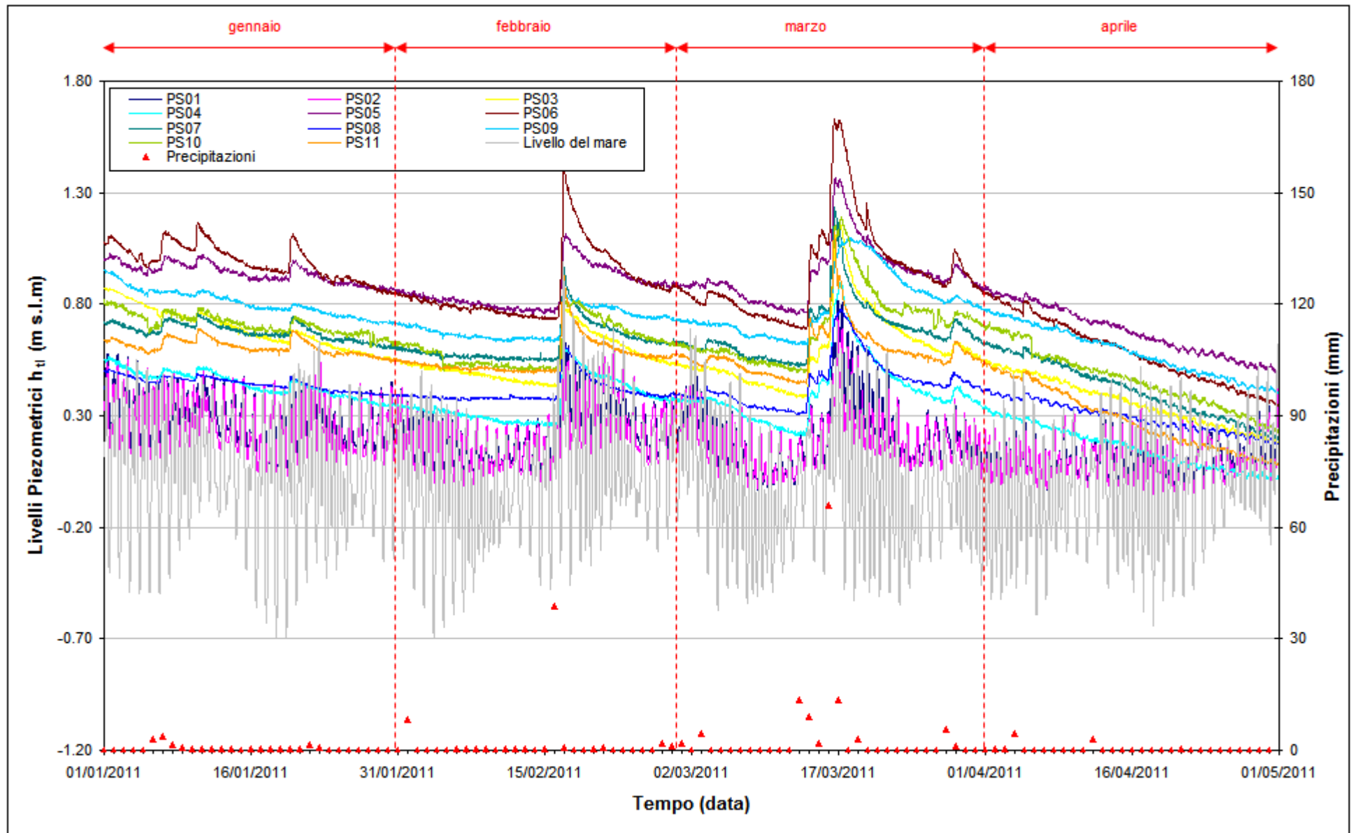
Fig. 2.6 - Livelli piezometrici ( h_u ) relativi ai piezometri superficiali nel periodo di monitoraggio 01/01/2011 - 30/04/2011.
