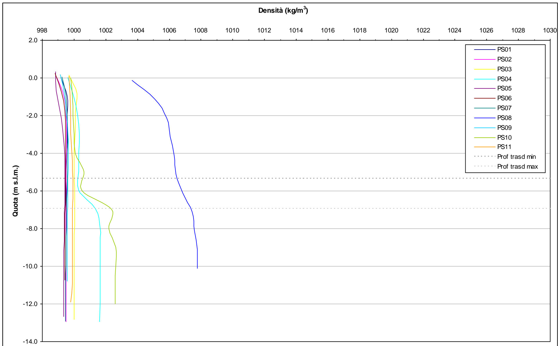
Fig. 4.1- Profili verticali di densità piezometri superficiali - 3-4 giugno 2009.
