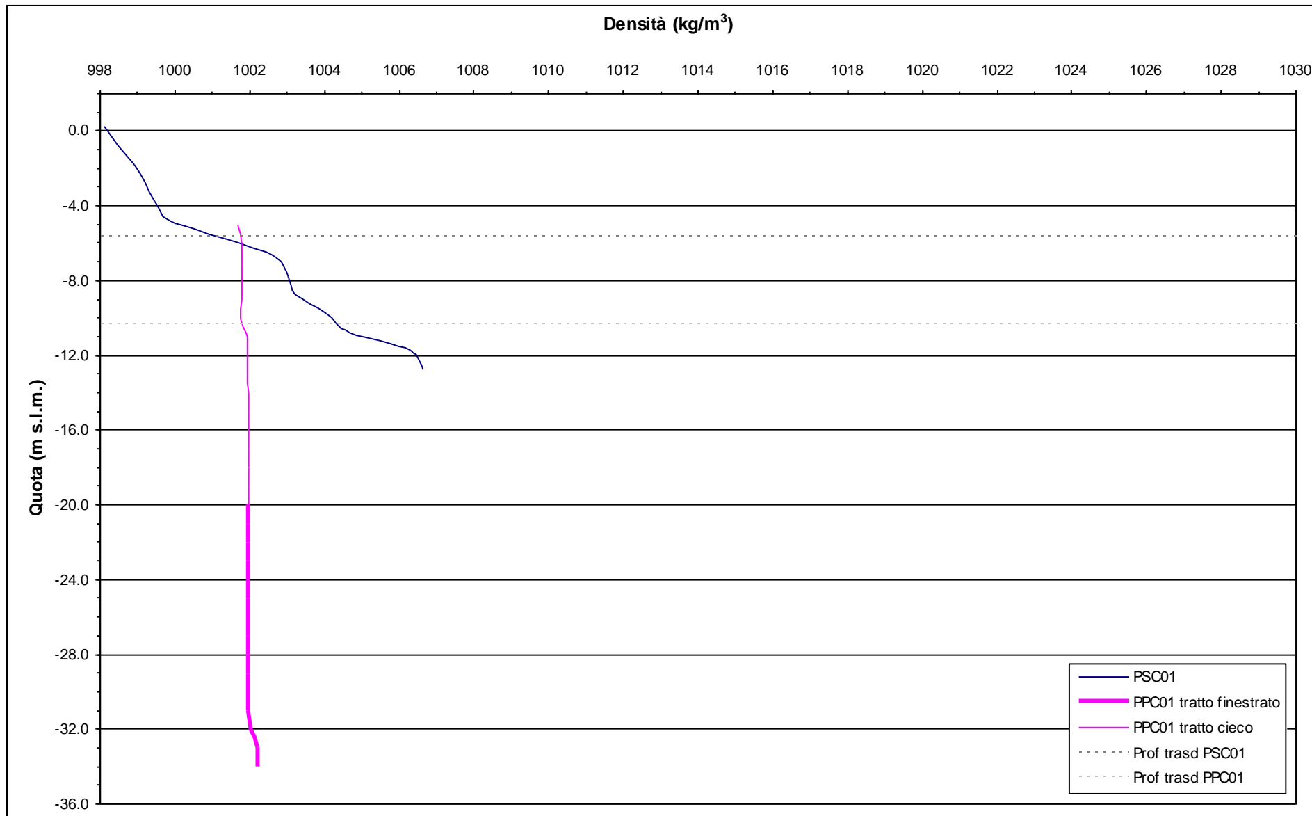
. 11.4.- Profili verticali di densità - 9 settembre 2009.
