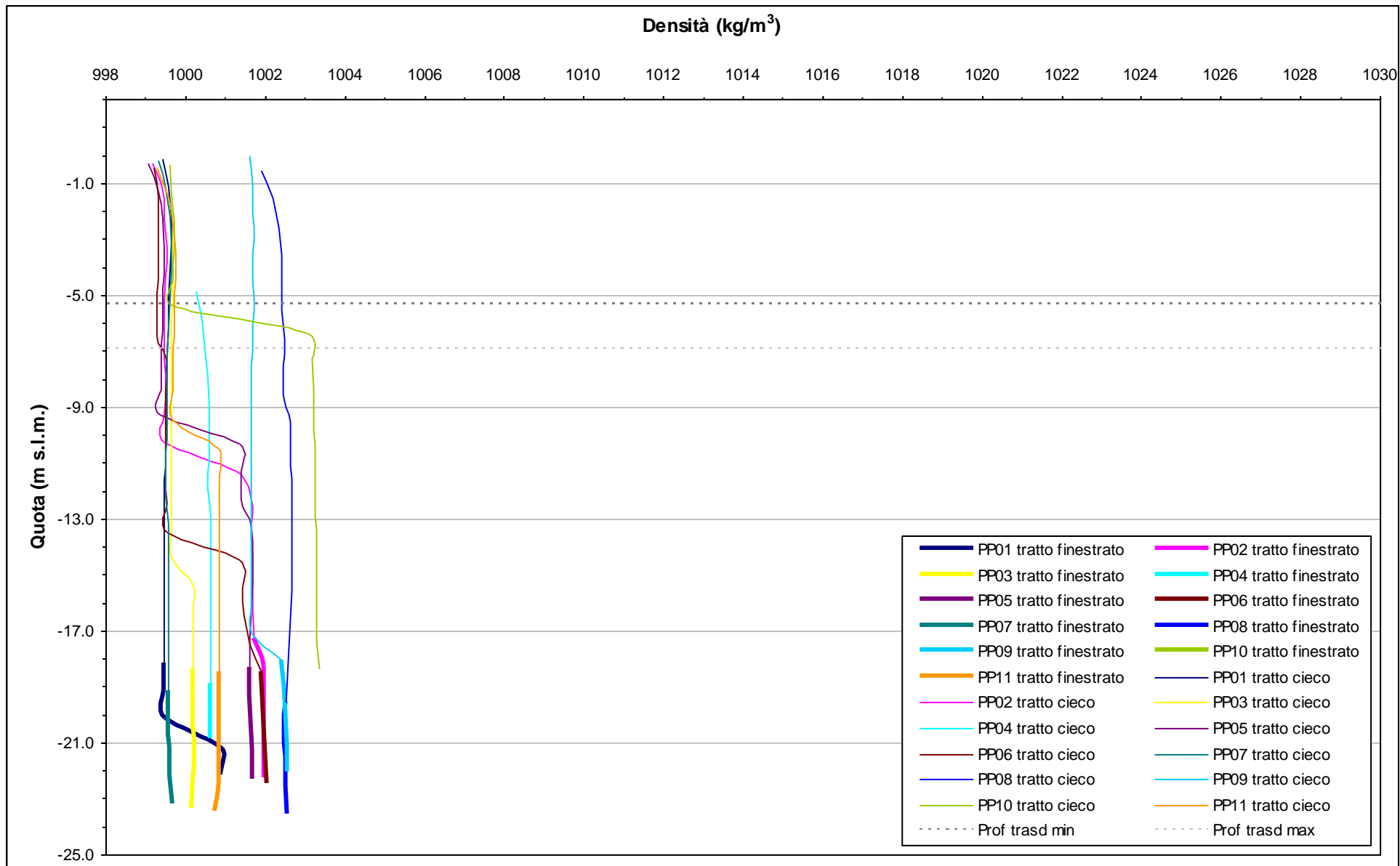
Fig. 4.5 - Profili verticali di densità piezometri profondi - 3-4 giugno 2009.
