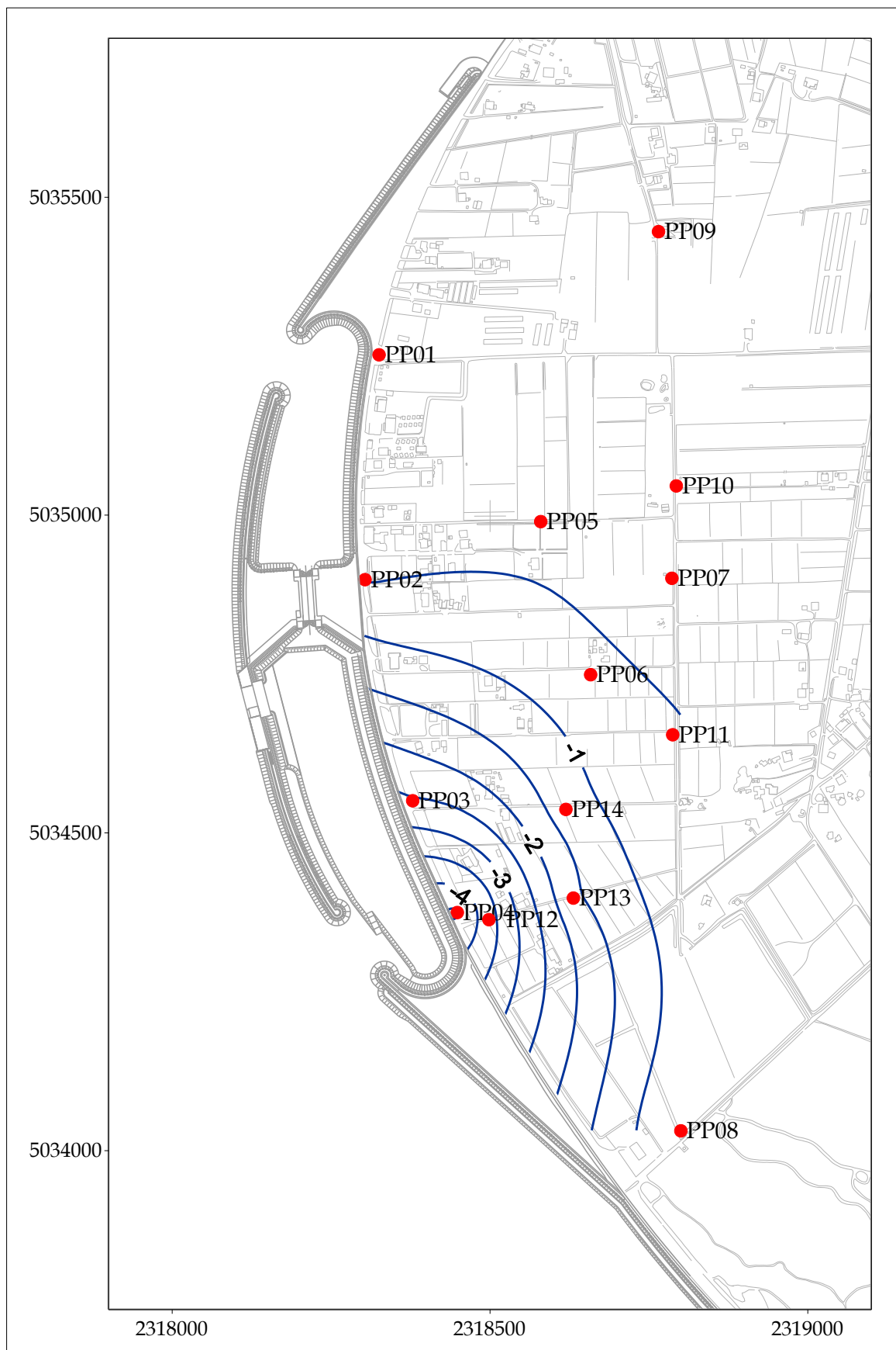
Fig. 5.11 - Piezometria profonda - luglio 2009 ( h_{pi} - m s.l.m.).
