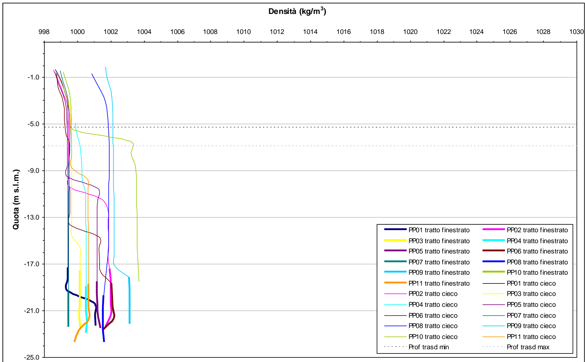
Fig. 4.7 - Profili verticali di densità piezometri profondi - 4 agosto 2009.
