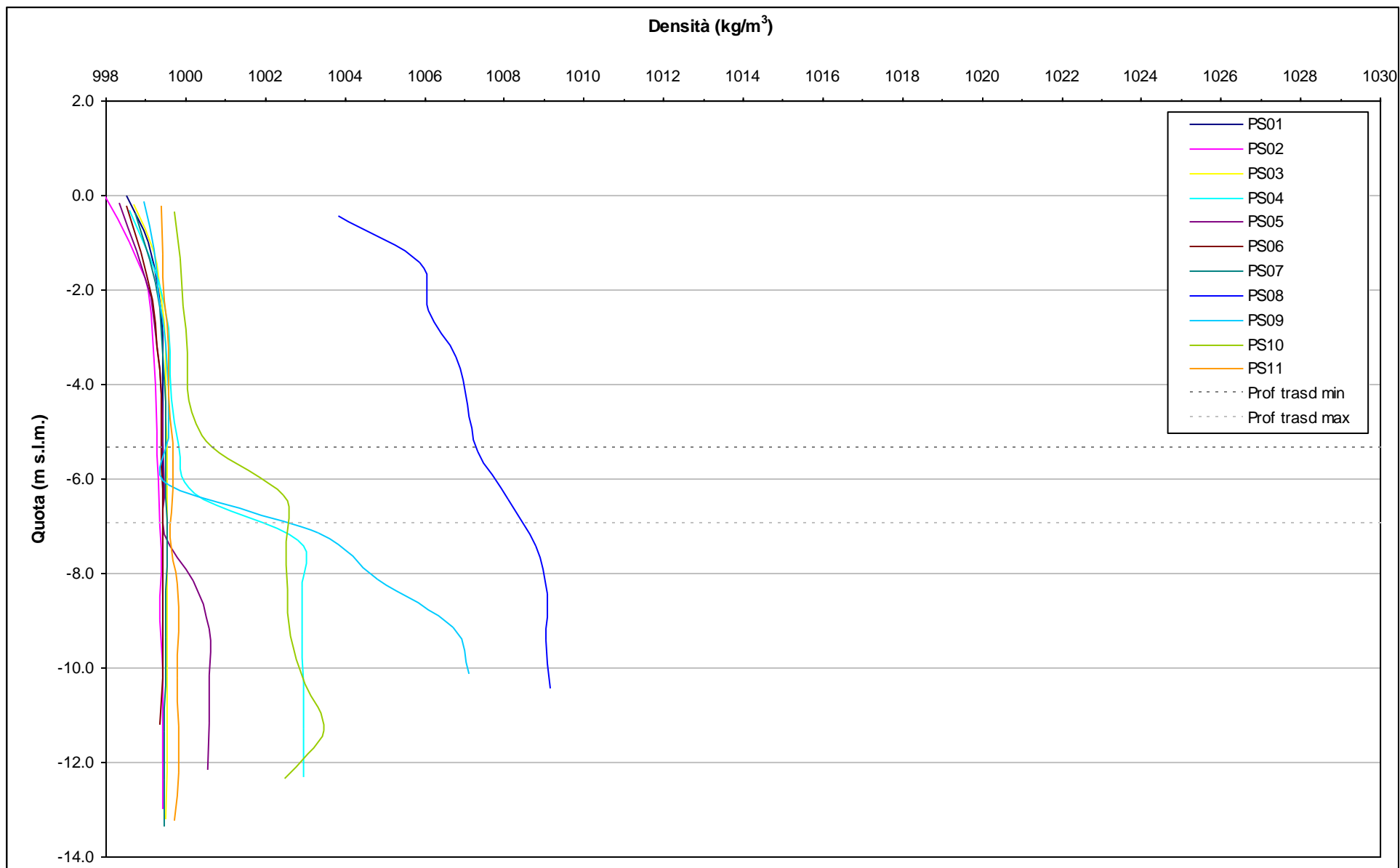
Fig. 4.3 - Profili verticali di densità piezometri superficiali - 4 agosto 2009.
