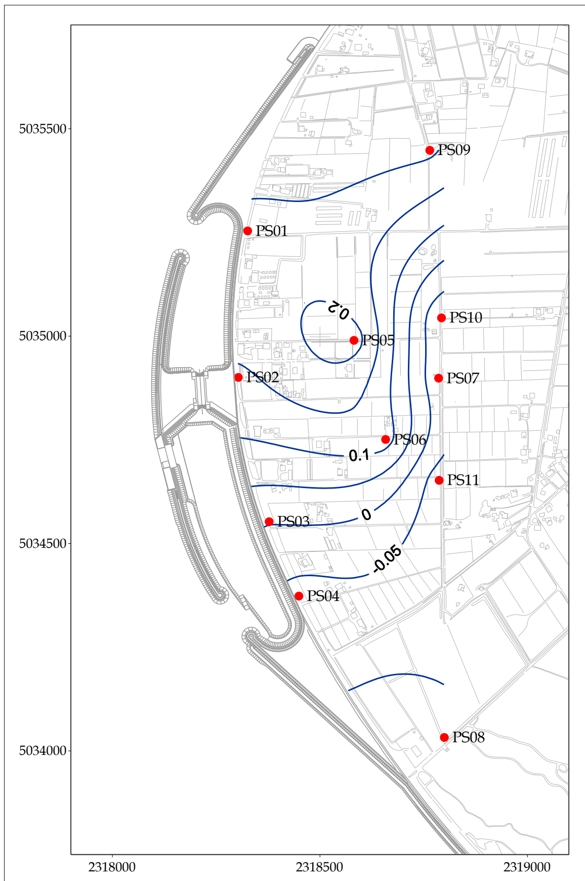
Fig. 5.5- Piezometria superficiale - giugno 2009 (h ti - m s.l.m.).
