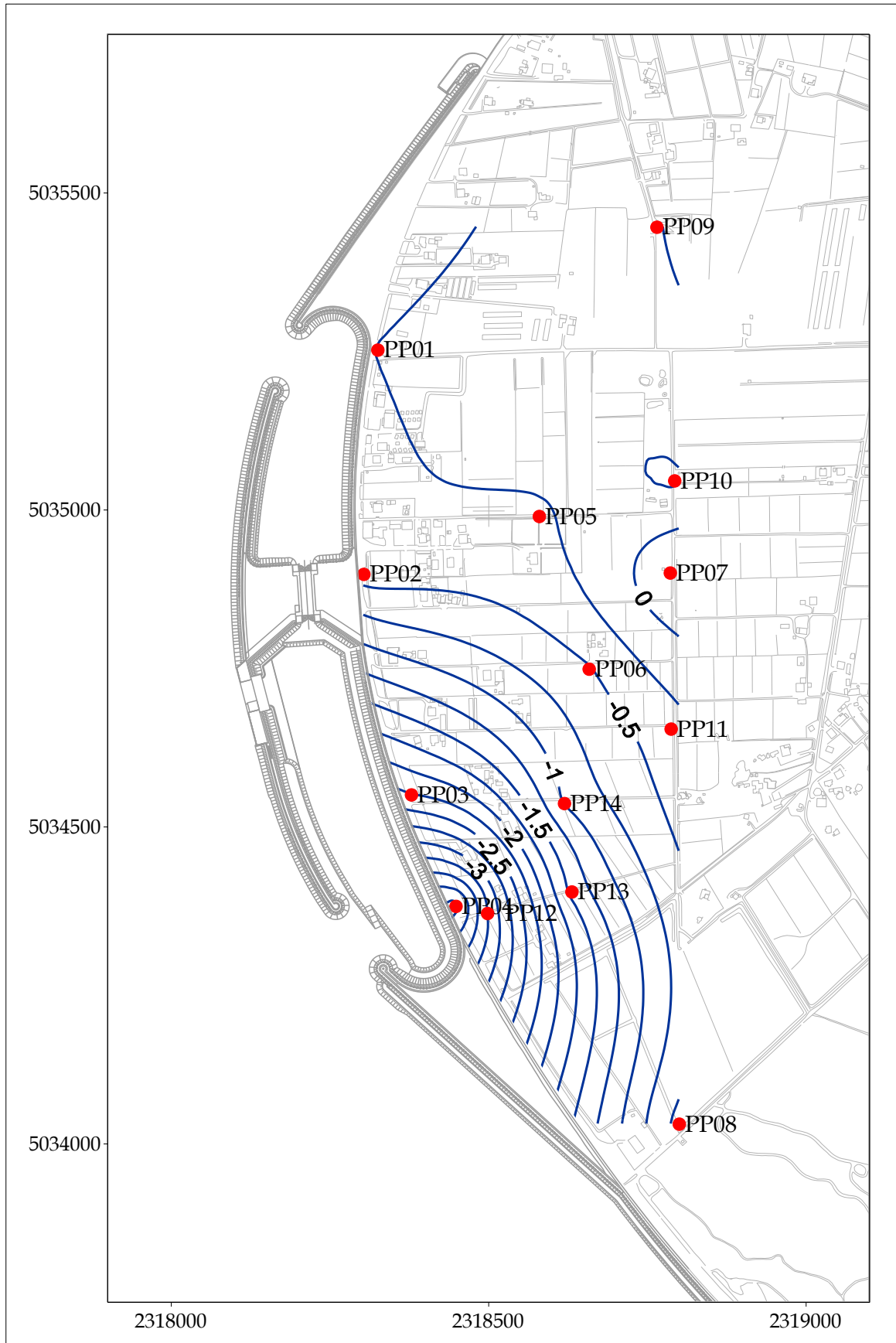
Fig. 5.9 - Piezometria profonda - maggio 2009 ( h_{il} - m s.l.m.).
