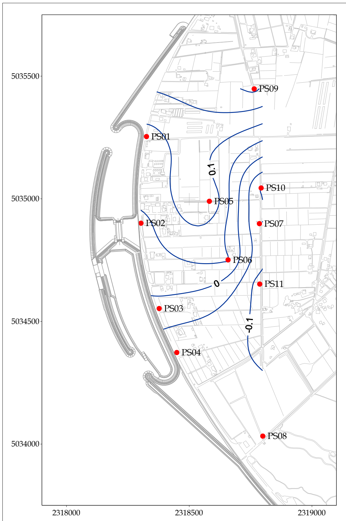
Fig. 5.6 - Piezometria superficiale - luglio 2009 ( h_d - m s.l.m.).
