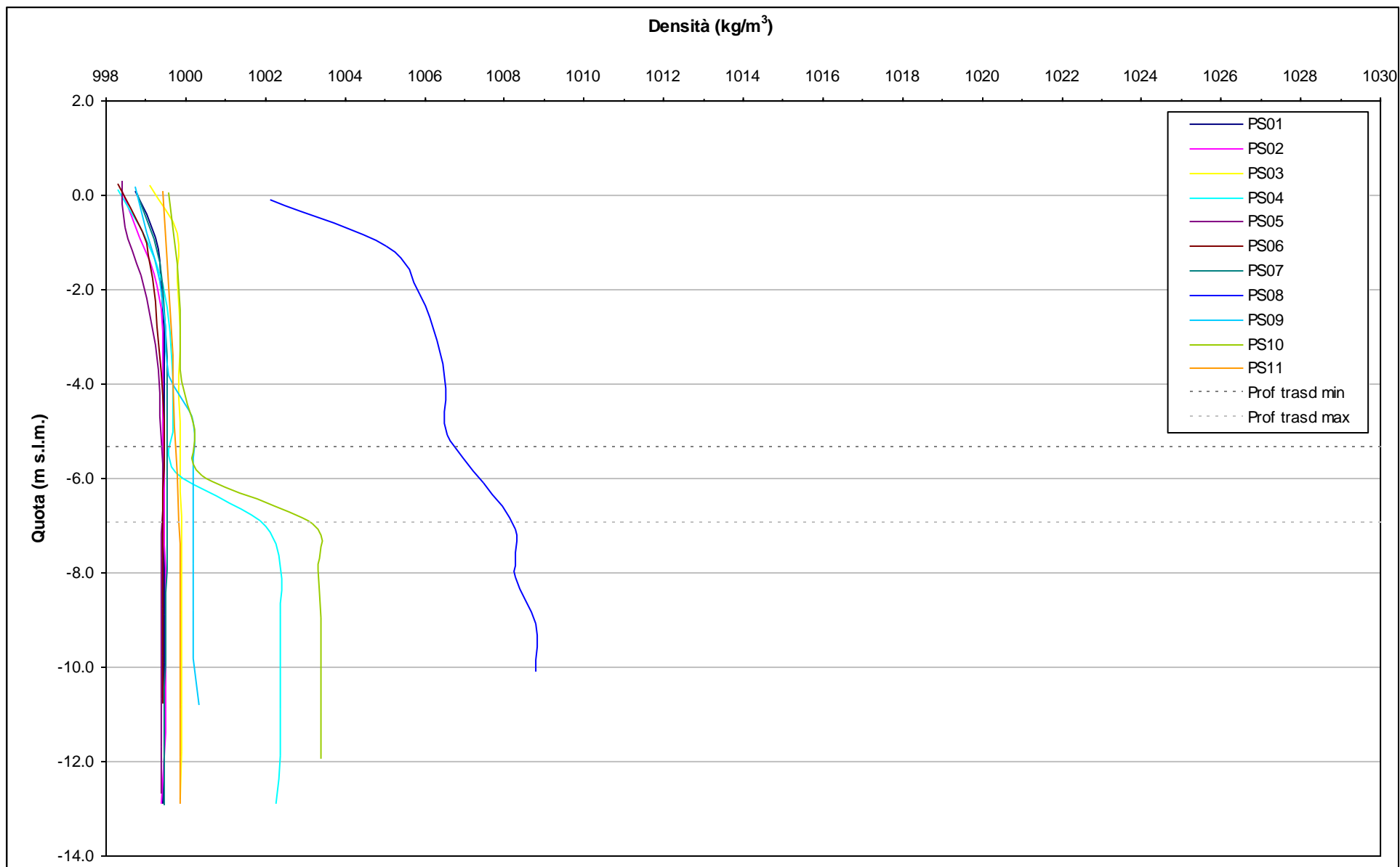
Fig. 4.2- Profili verticali di densità piezometri superficiali - 5 luglio 2009.
