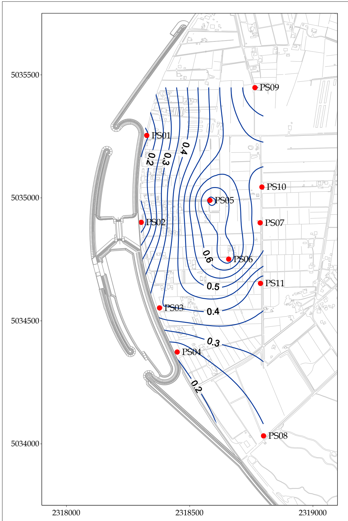
Fig. 5.4 - Piezometria superficiale - maggio 2009 ( h_{II} - m s.l.m.).
