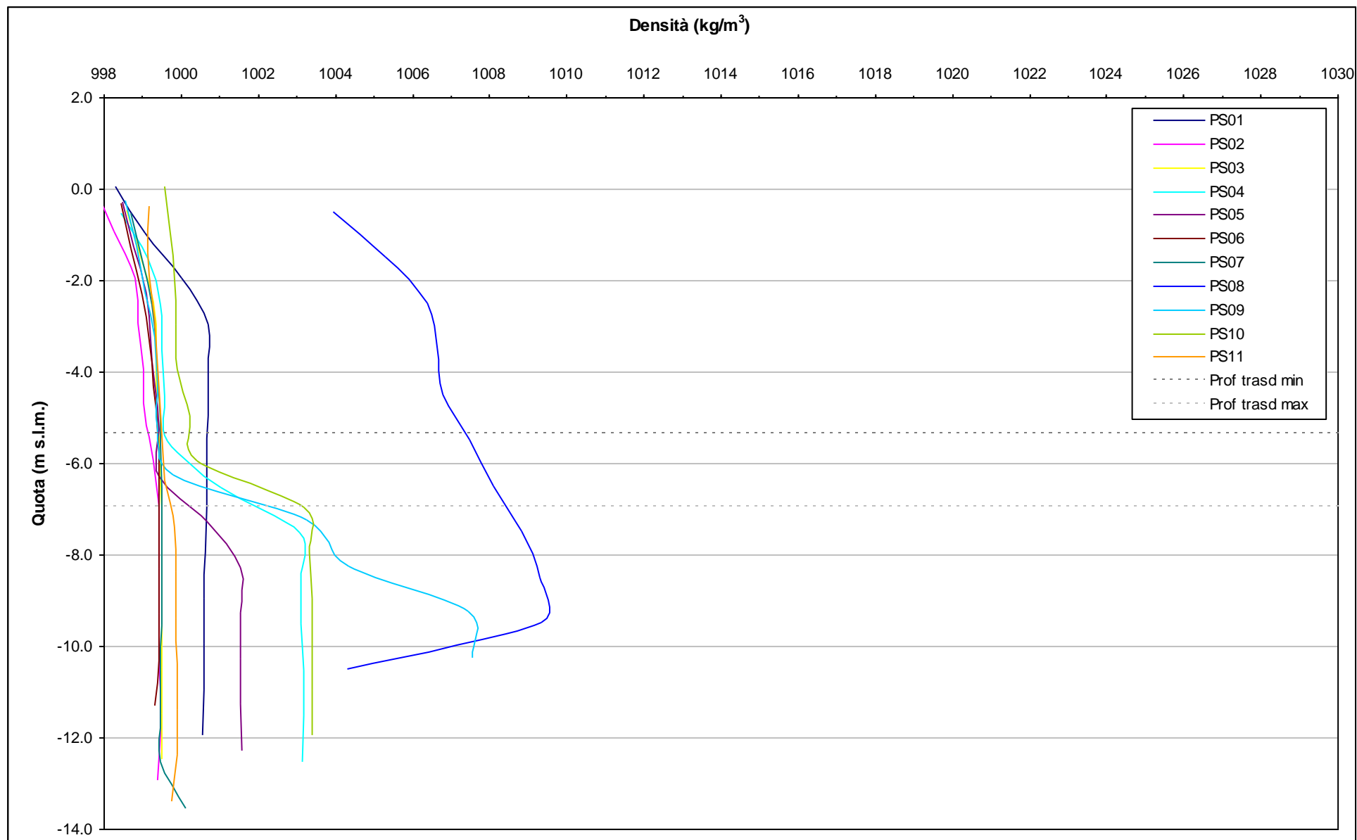
Fig. 4.4 - Profili verticali di densità piezometri superficiali - 9 settembre 2009.
