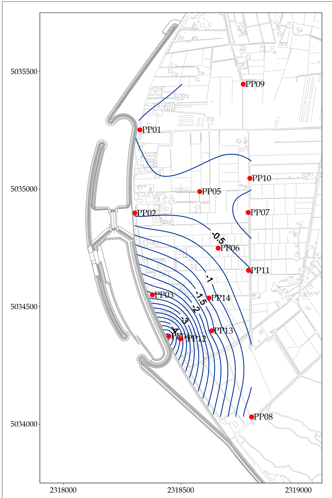
Fig. 5.10 - Piezometria profonda - giugno 2009 ( h_{tl} - m s.l.m.).
