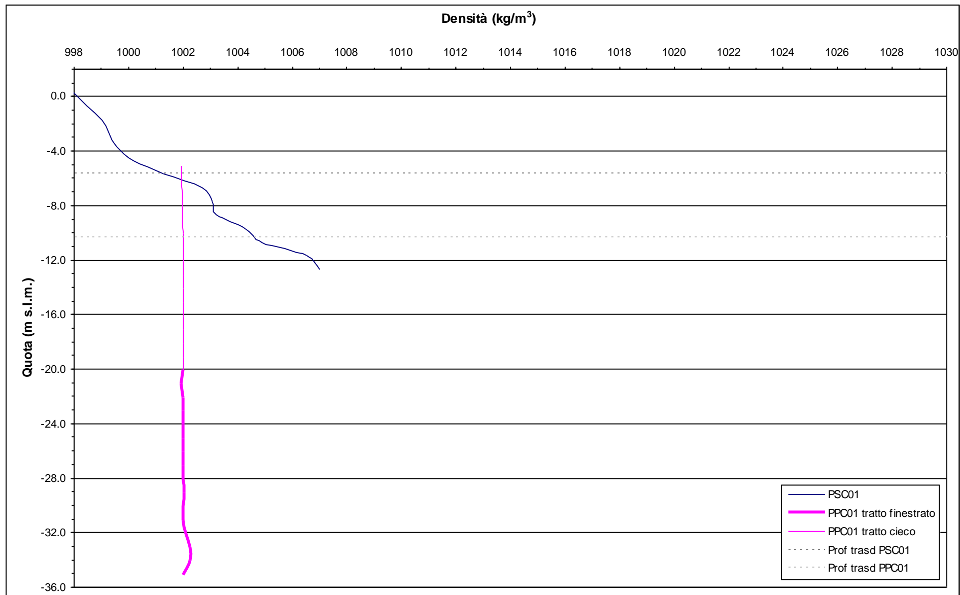
. 11.3.- Profili verticali di densità - 4 agosto 2009.
