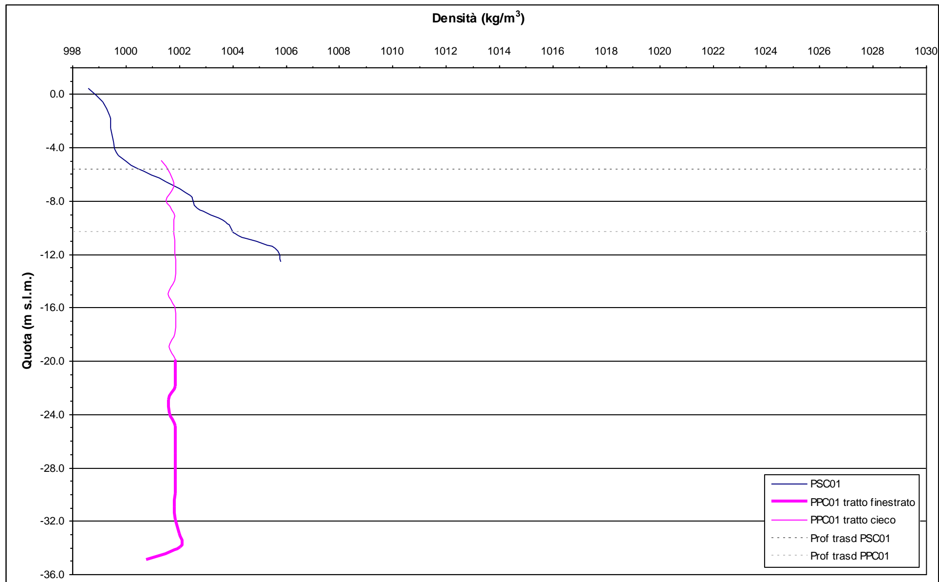
Fig. 11.1 Profili verticali di densità - 3 giugno 2009.
