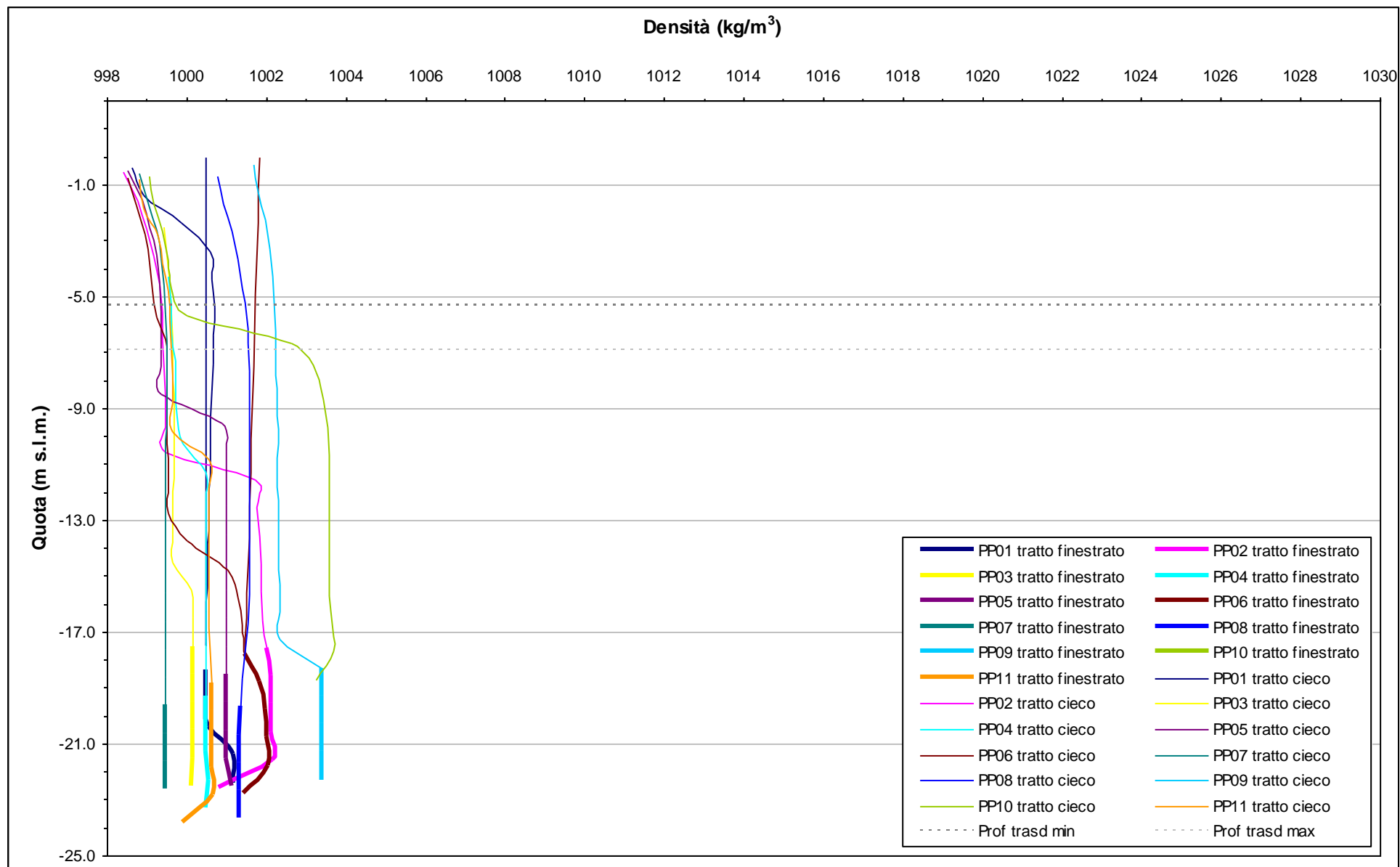
Fig. 4.8 - Profili verticali di densità piezometri profondi - 9 settembre 2009.
