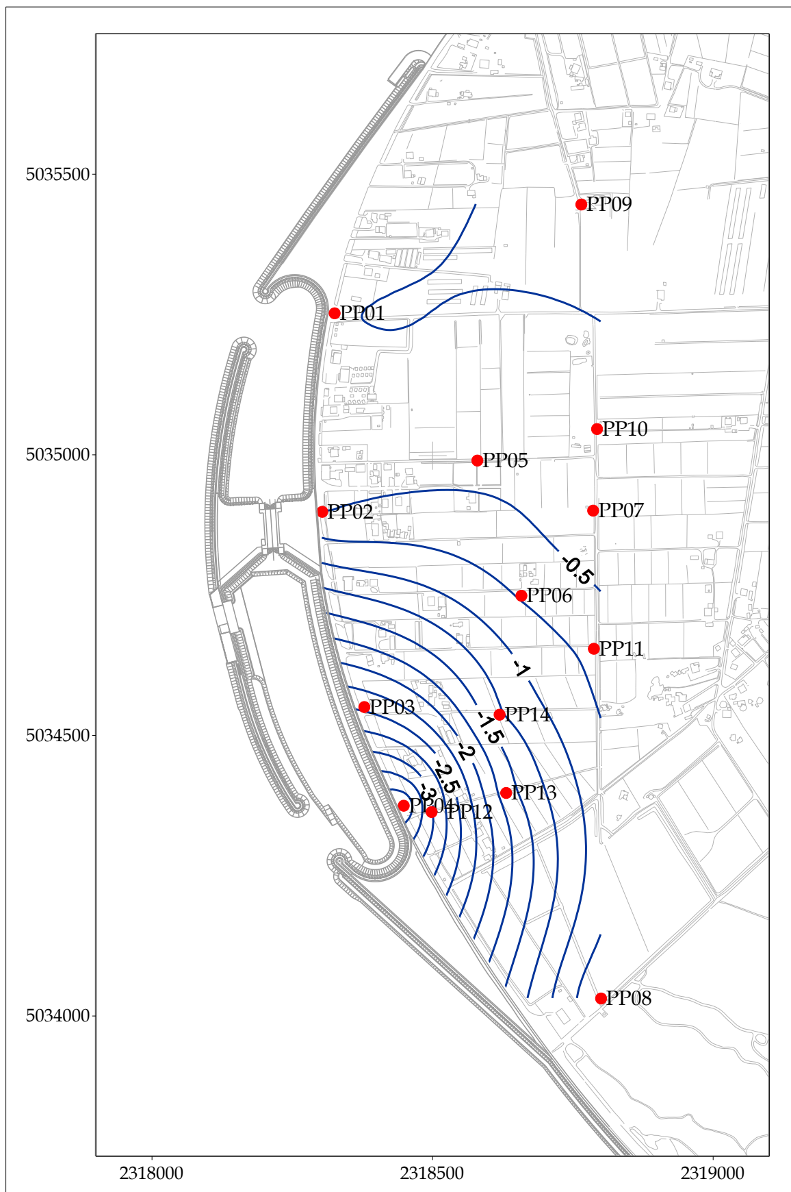
Fig. 5.12 - Piezometria profonda - agosto 2009 (h d - m s.l.m.).
