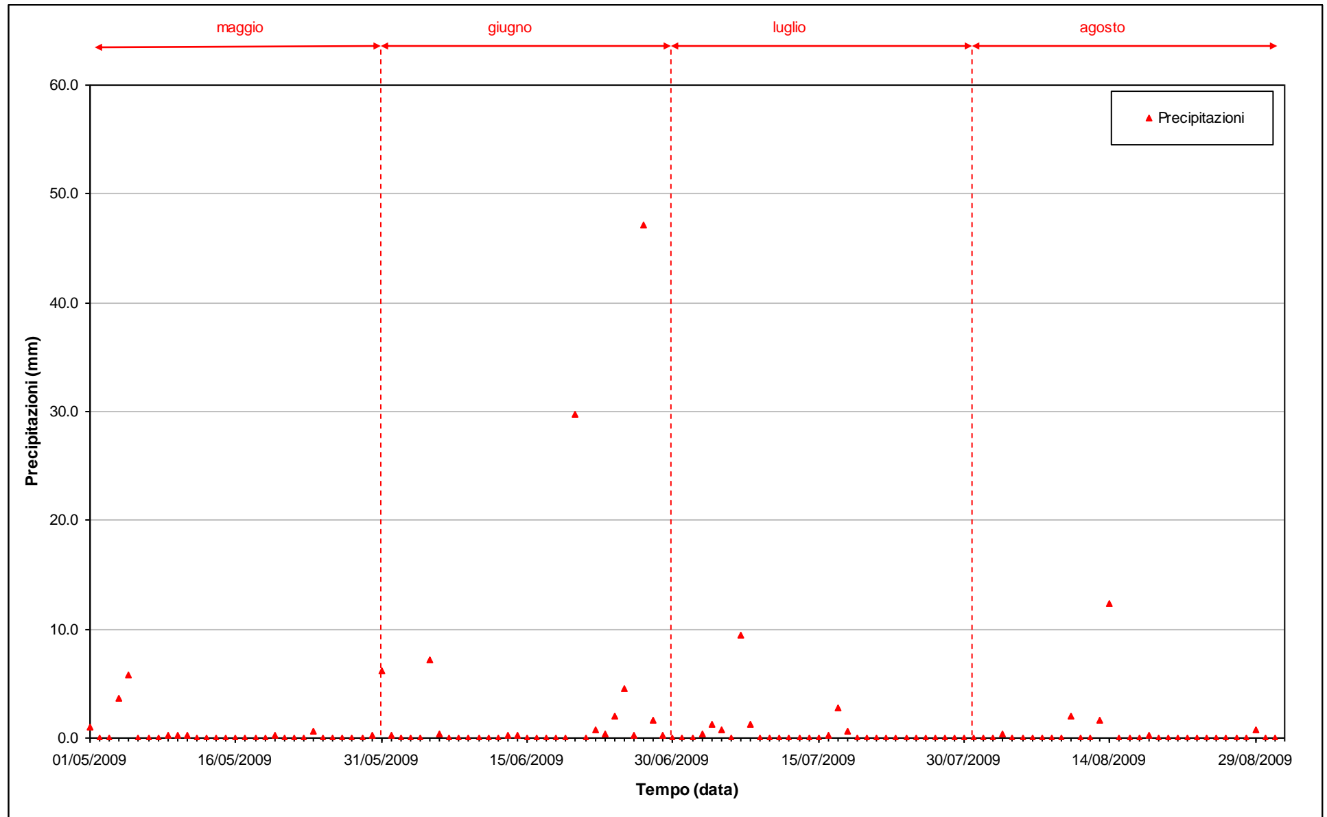
Fig. 2.2 - Precipitazioni registrate nel periodo di monitoraggio 01/05/2009 - 31/08/2009.
