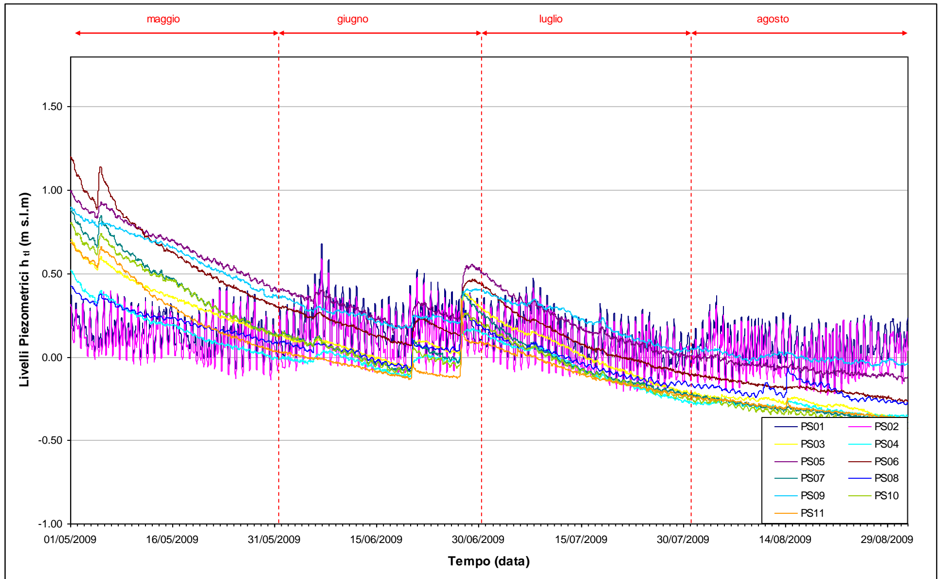
Fig. 2.6 - Livelli piezometrici ( h_u ) relativi ai piezometri superficiali nel periodo di monitoraggio 01/05/2009 - 31/08/2009.
