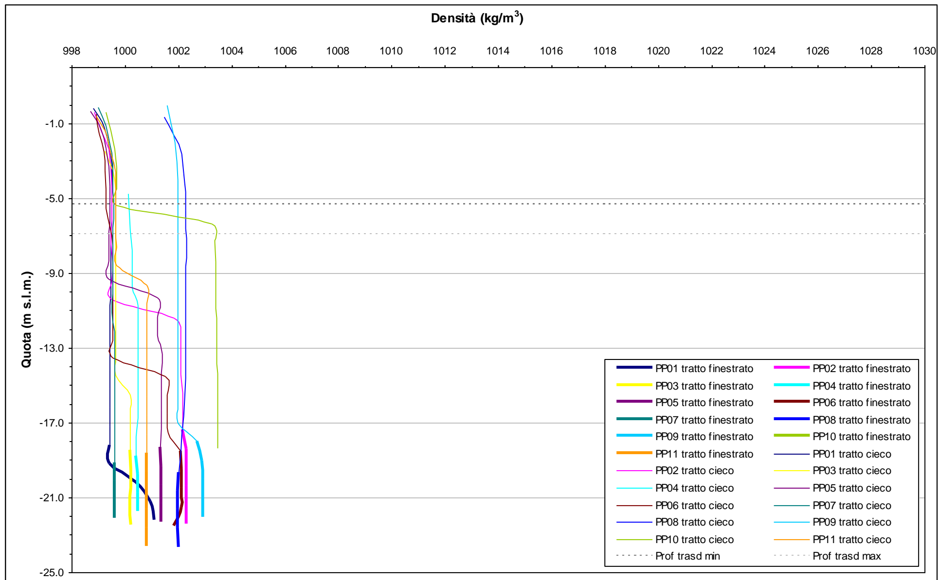
Fig. 4.6- Profili verticali di densità piezometri profondi - 5 luglio 2009.
