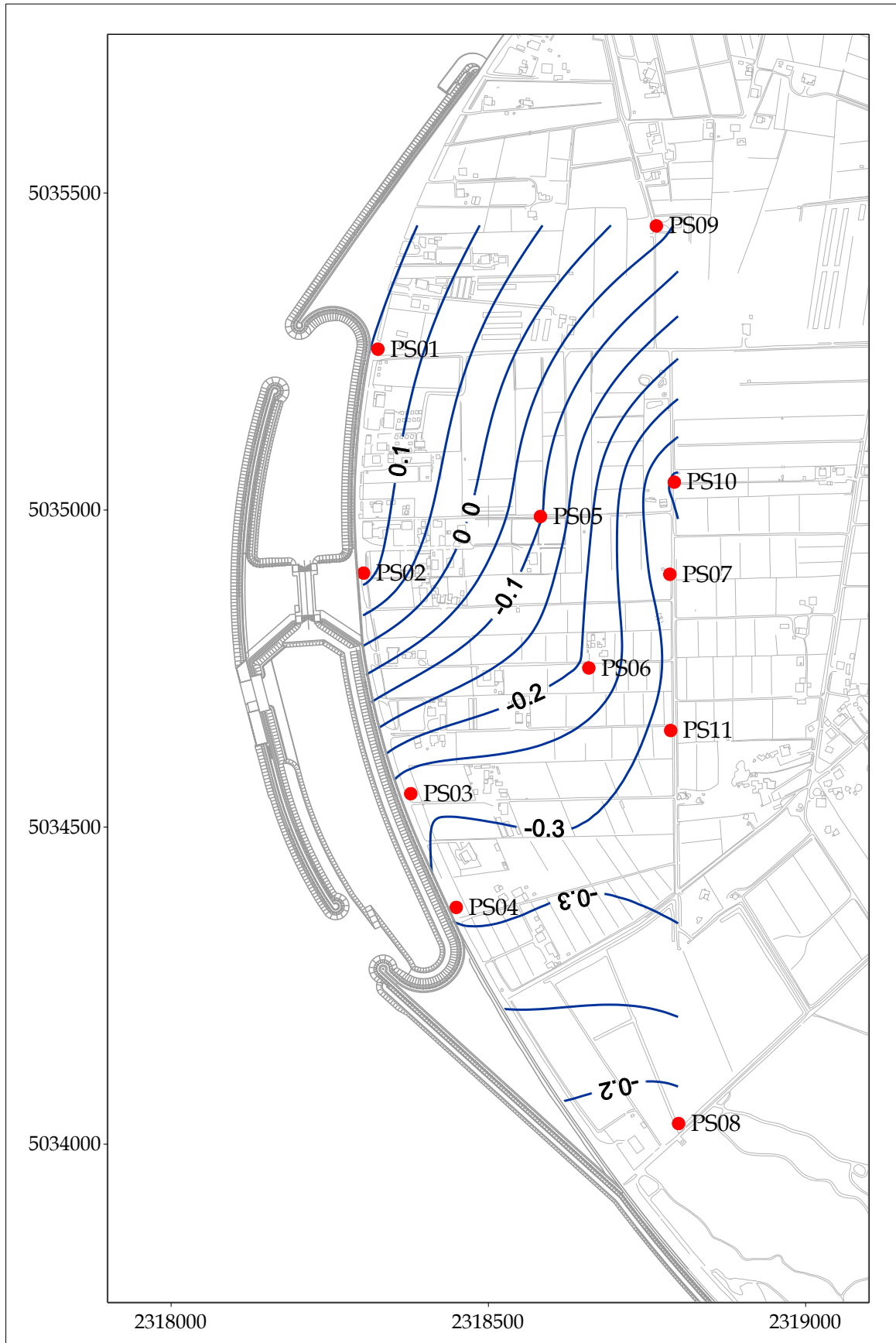
Fig. 5.7 - Piezometria superficiale - agosto 2009 ( h_{tl} - m s.l.m.).
