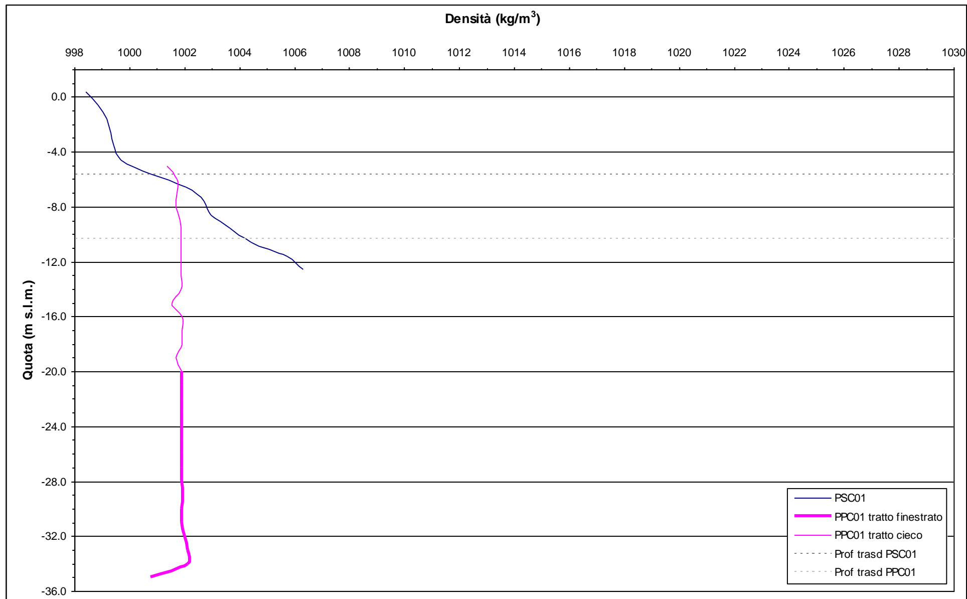
Fig. 11.2.- Profili verticali di densità - 5 luglio 2009.
