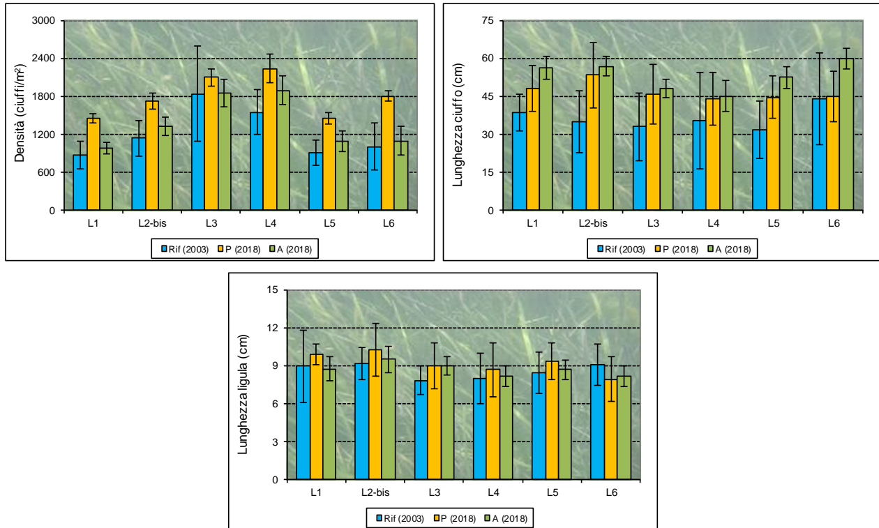
Figura 3.1. Rappresentazione grafica dei valori medi (e delle deviazioni standard) di alcuni indicatori strutturali (densità ciuffi/m 2 , lunghezza del ciuffo e della ligula in cm) dello studio di riferimento del 2003 (primavera-estate-autunno) e della primavera (P) e dell'autunno (A) (2018).
