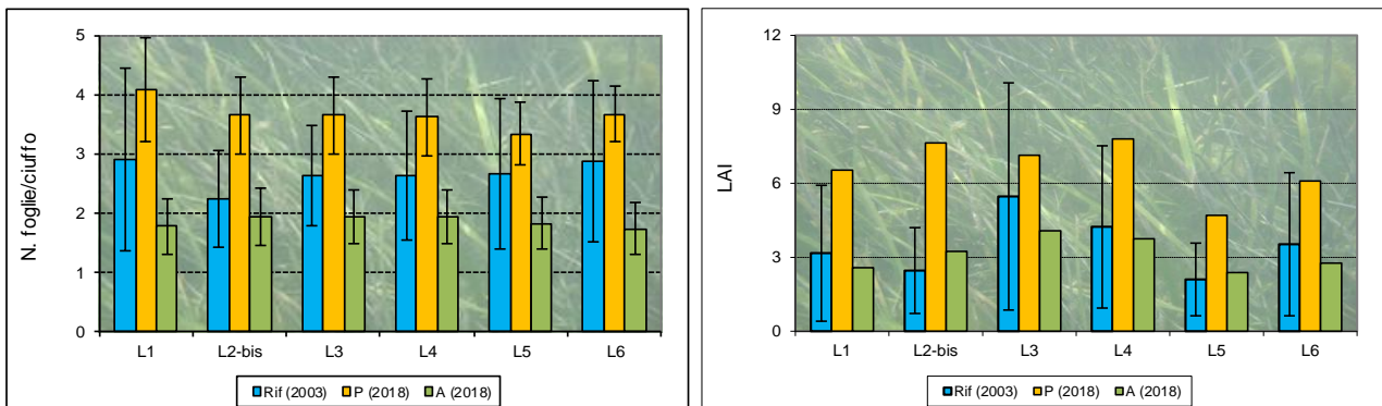
Figura 3.2. Rappresentazione grafica dei valori medi (e delle deviazioni standard) di alcuni indicatori strutturali (numero foglie/ciuffo e LAI) dello studio di riferimento del 2003 (primavera-estate-autunno) e della primavera (P) e dell'autunno (A) (2018).
