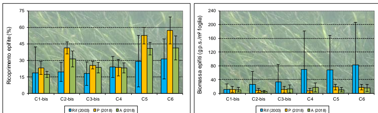
Figura 3.16. Rappresentazione grafica dei valori medi (e delle deviazioni standard) di alcuni indicatori strutturali (ricoprimento % e biomassa g p.s.) dello studio di riferimento del 2003(primavera-estate-autunno) e della primavera (P) e dell'autunno (A) (2018).
