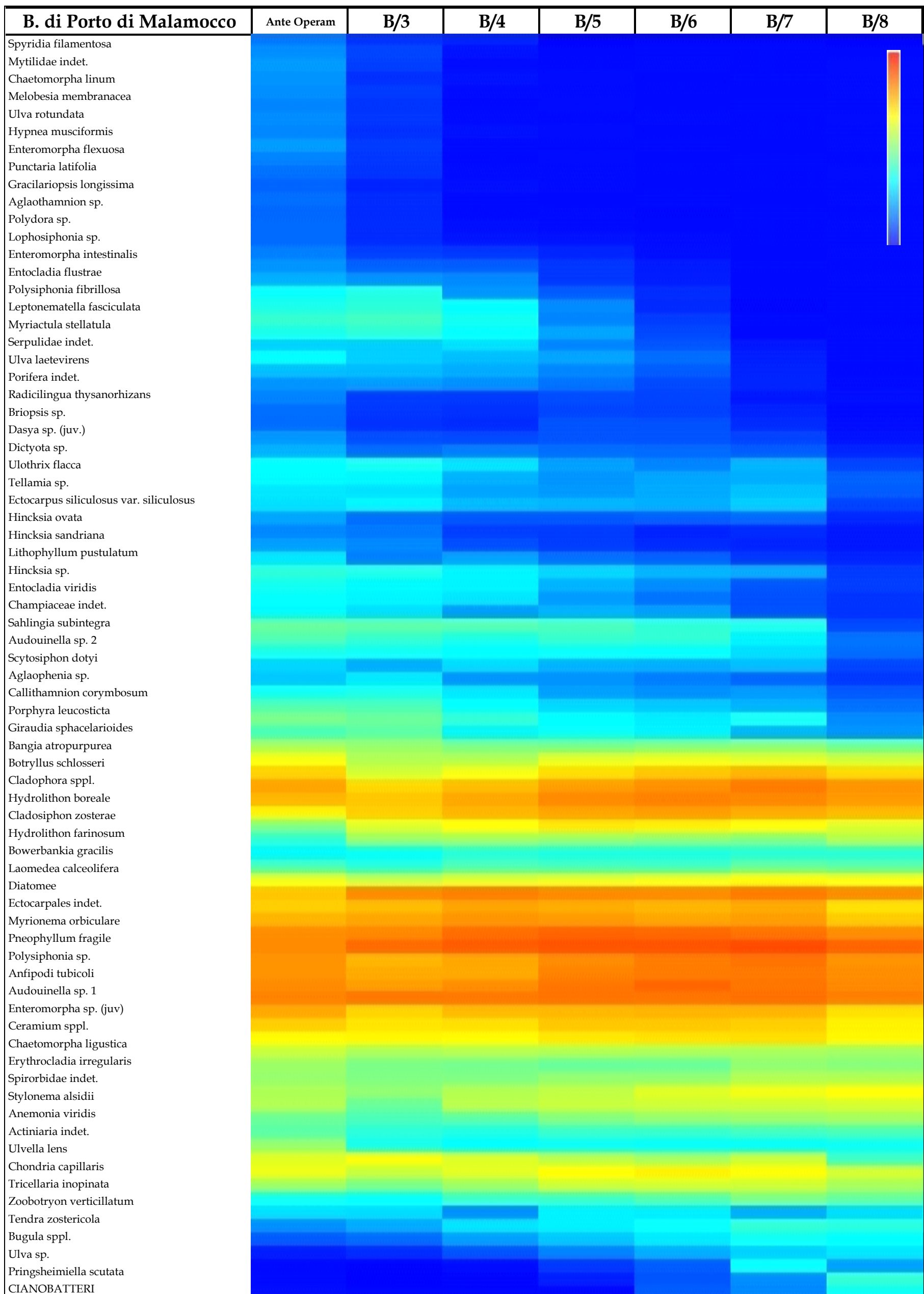
Figura A.11 - Bocca di porto di Malamocco: Matrix Plot dei valori di frequenza di rinvenimento dei taxa per i 6 anni di monitoraggio ( Ante operam = Studio B.6.78/I; B/1-B/8 = Studi B.6.72 B/1-B/8, 2005-2012). Valori (log+1) trasformati ( rosso = massima frequenza; blu = assenza di rilevamenti).
