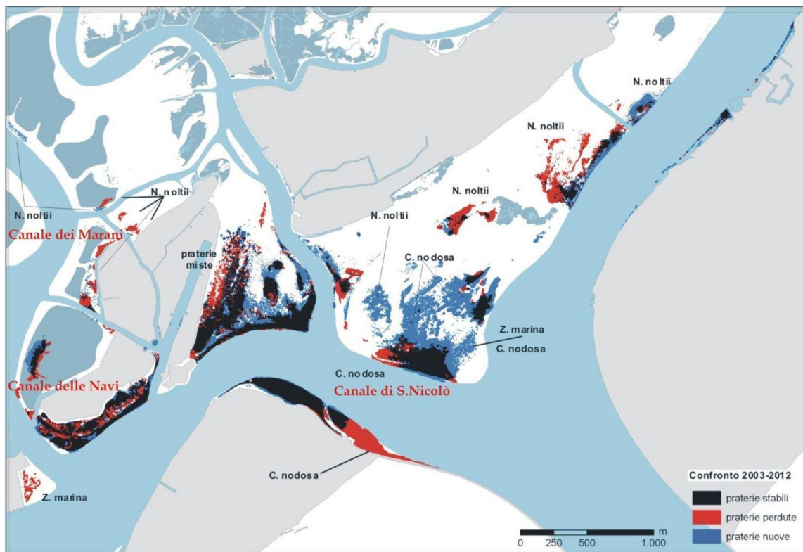
Figura 3.6 – Porto di Lido: variazioni delle coperture a fanerogame marine tra il 2003 e il 2012.
