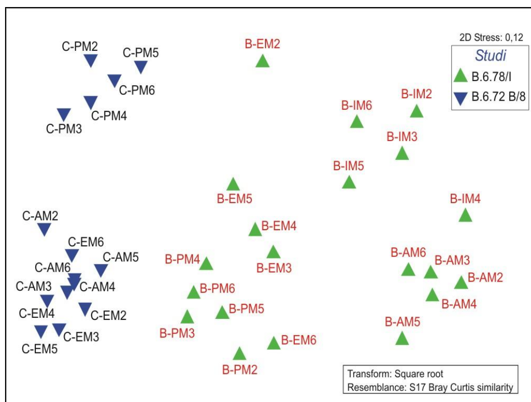
Figura A.4 - MultiDimensional Scaling (MDS) dell'ordinamento in base alla similarità della comunità epifitica nelle stazioni a Cymodocea nodosa (dati di ricoprimento trasformati con radice quadrata). [B=B.6.78/I; C=B.6.72 B/8; I=inverno; P=primavera; E=estate; A=autunno]
