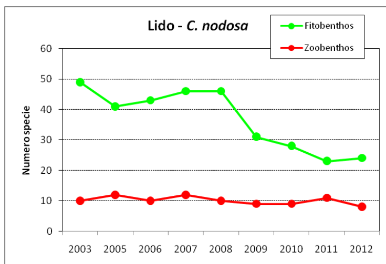
Figura 3.1 – Numero totale di specie (elenco floristico-faunistico) per le 6 stazioni della bocca di porto di Lido a Cymodocea nodosa , tra lo Studio B.6.78/I del 2003 e quello attuale B.6.72 B/8 (2012).
