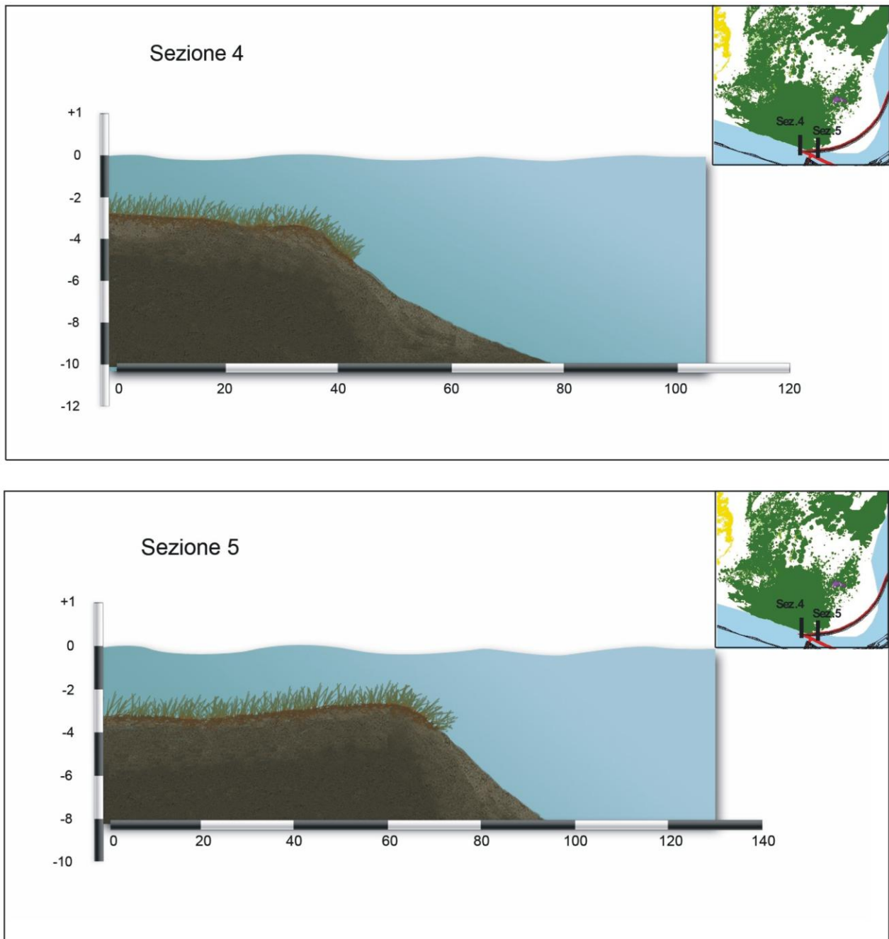
Figura 3.22 – Schema semplificato della tipologia del limite delle praterie lungo due transetti. Per la realizzazione del profilo si è fatto riferimento ai più recenti dati batimetrici multibeam del 2001 e rilievi in campo con profondimetro del 2012.
