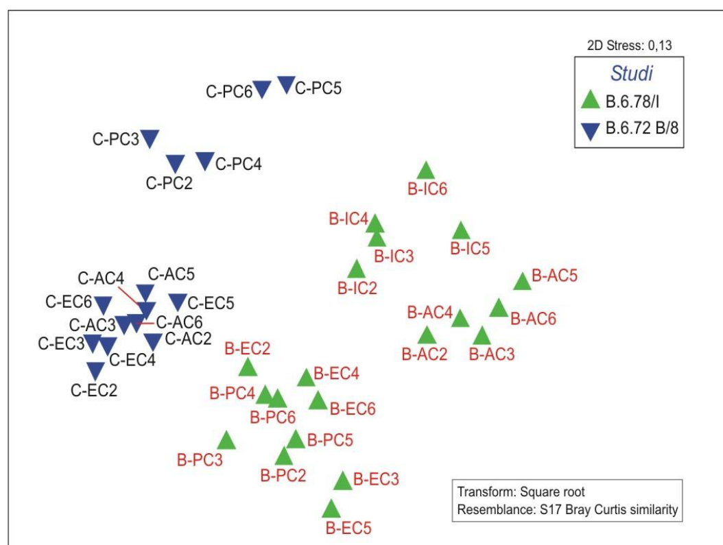
Figura A.8 - MultiDimensional Scaling (MDS) dell'ordinamento in base alla similarità della comunità epifitica nelle stazioni a Cymodocea nodosa (dati di ricoprimento trasformati con radice quadrata). [B=B.6.78/I; C=B.6.72 B/8; I=inverno; P=primavera; E=estate; A=autunno].
