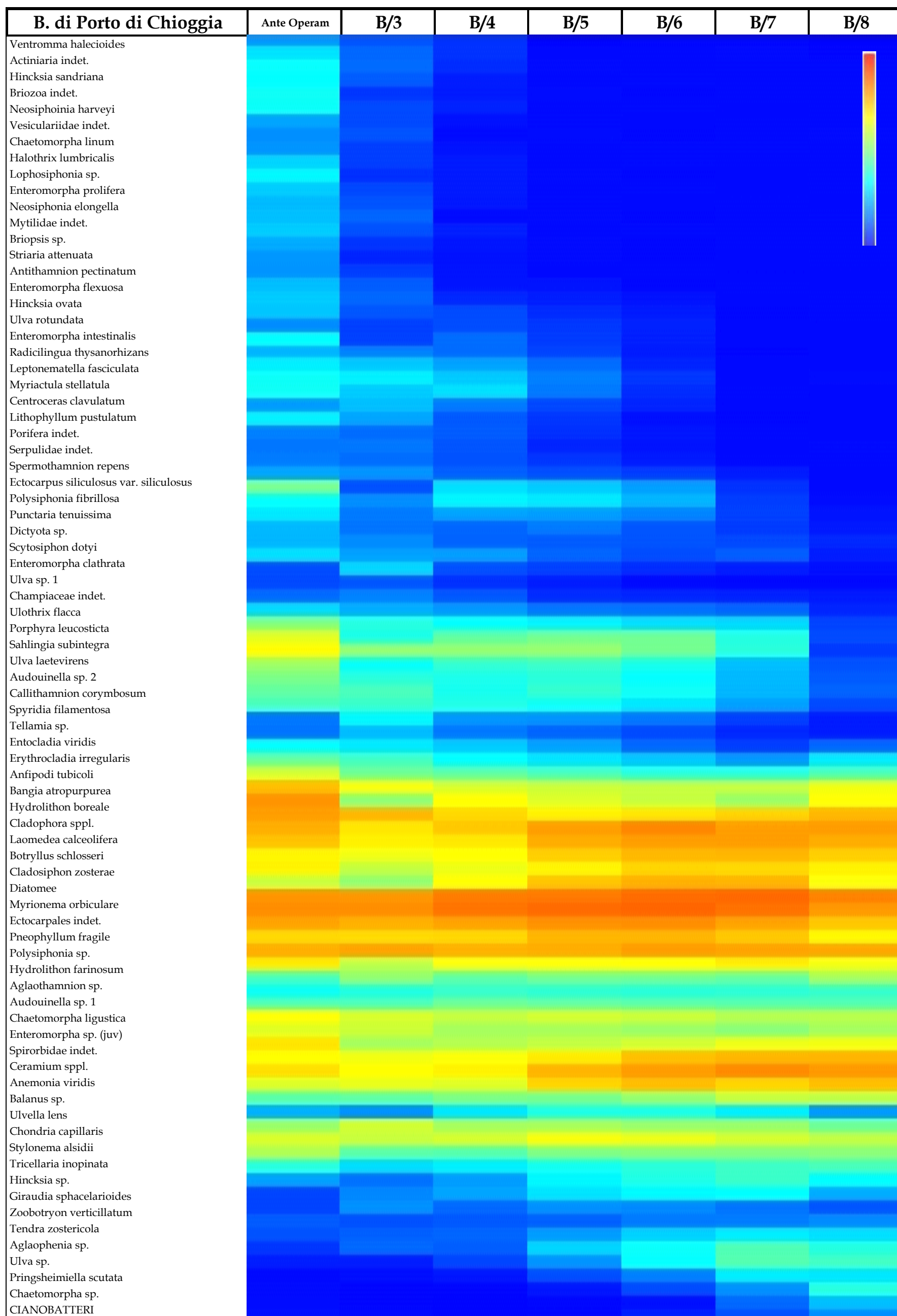
Figura A.12 - Bocca di porto di Chioggia: Matrix Plot dei valori di frequenza di rinvenimento dei taxa per i 6 anni di monitoraggio ( Ante operam = Studio B.6.78/I; B/1-B/8 = Studi B.6.72 B/1-B/8, 2005-2012). Valori (log+1) trasformati ( rosso = massima frequenza; blu = assenza di rilevamenti).
