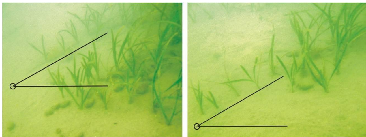
Figura 3.24 – Esempi di rizomi che si protendono verso il margine inclinato del canale.
