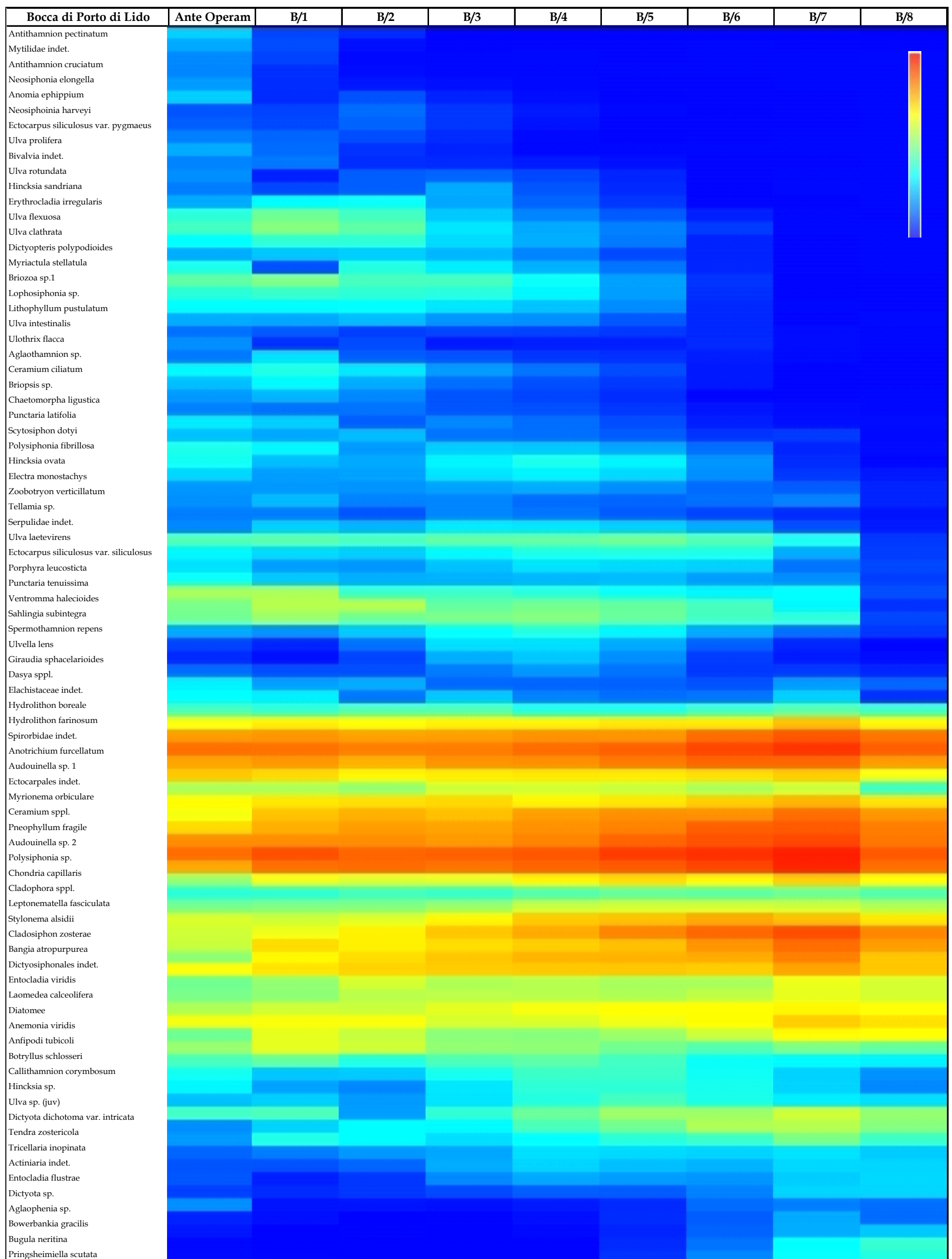
Figura A.10 - Bocca di porto di Lido: Matrix Plot dei valori di frequenza di rinvenimento dei taxa per gli 8 anni di monitoraggio ( Ante operam = Studio B.6.78/I; B/1-B/8 = Studi B.6.72 B/1-B/8, 2005-2012). Valori (log+1) trasformati ( rosso = massima frequenza; blu = assenza di rilevamenti).
