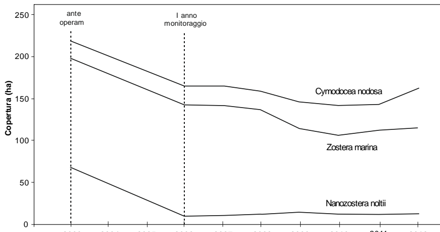
Figura 3.10 – Bocca di porto di Chioggia: variazione delle coperture avvenute tra il 2003 e il 2012 per le diverse tipologie di praterie. Nessun rilievo è stato eseguito nel 2004 e nel 2005 per questa bocca di porto.
