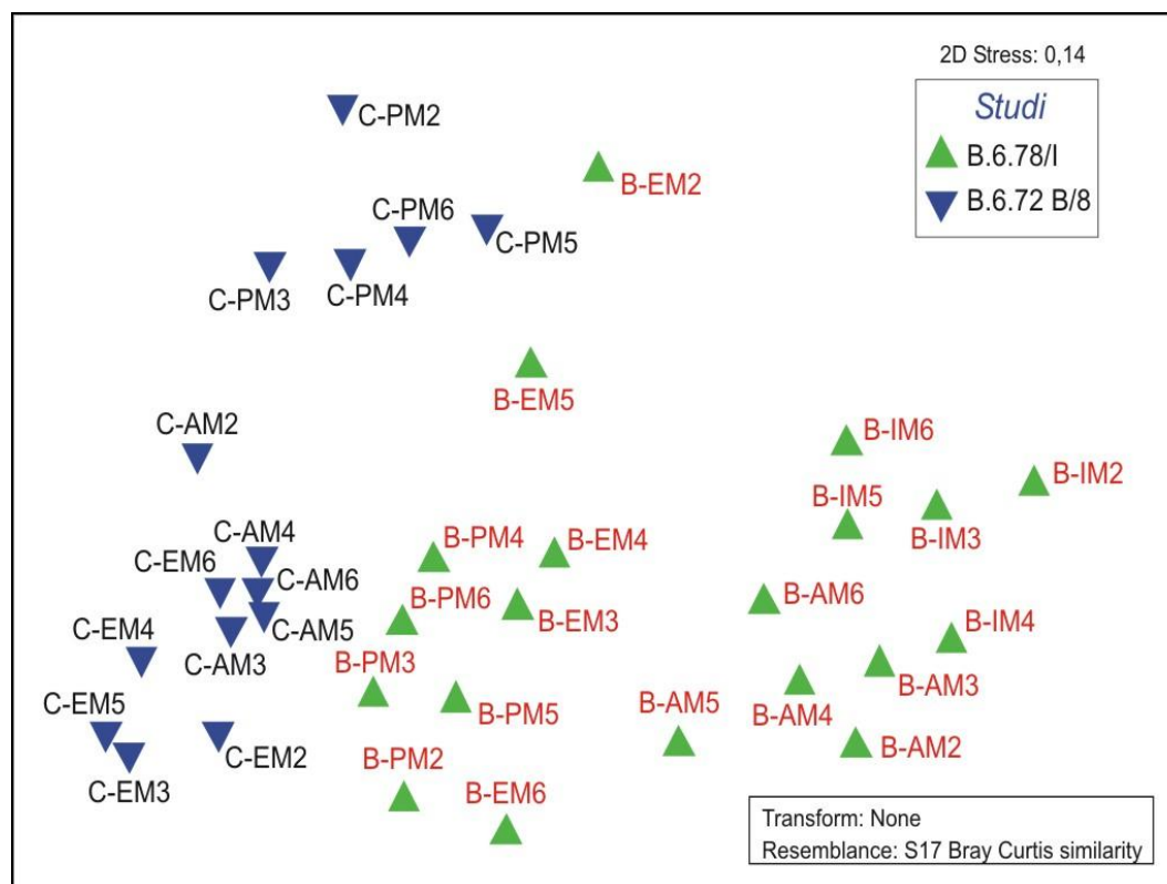
Figura A.3 - MultiDimensional Scaling (MDS) dell'ordinamento in base alla similarità della comunità epifitica nelle stazioni a Cymodocea nodosa (dati di ricoprimento senza trasformazione). [B=B.6.78/I; C=B.6.72 B/8; I=inverno; P=primavera; E=estate; A=autunno].
