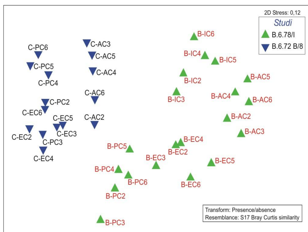
Figura A.9 - MultiDimensional Scaling (MDS) dell'ordinamento in base alla similarità della comunità epifitica nelle stazioni a Cymodocea nodosa (presenza-assenza). [B=B.6.78/I; C=B.6.72 B/8; I=inverno; P=primavera; E=estate; A=autunno].
