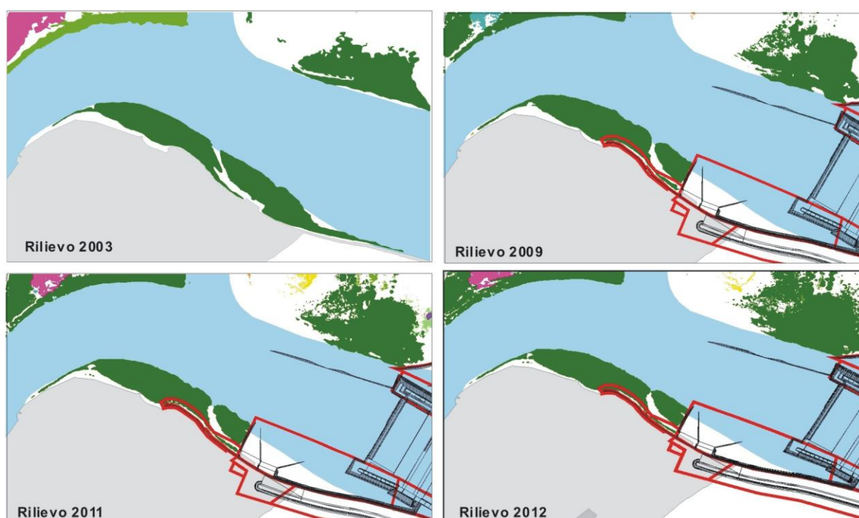
Figura 3.28 - Estensione della prateria negli anni 2003 e 2012. Dal 2008 è riportata l'impronta delle opere (in nero) e le aree in consegna alle ditte (in rosso) per la realizzazione dei lavori e movimentazione dei mezzi.
