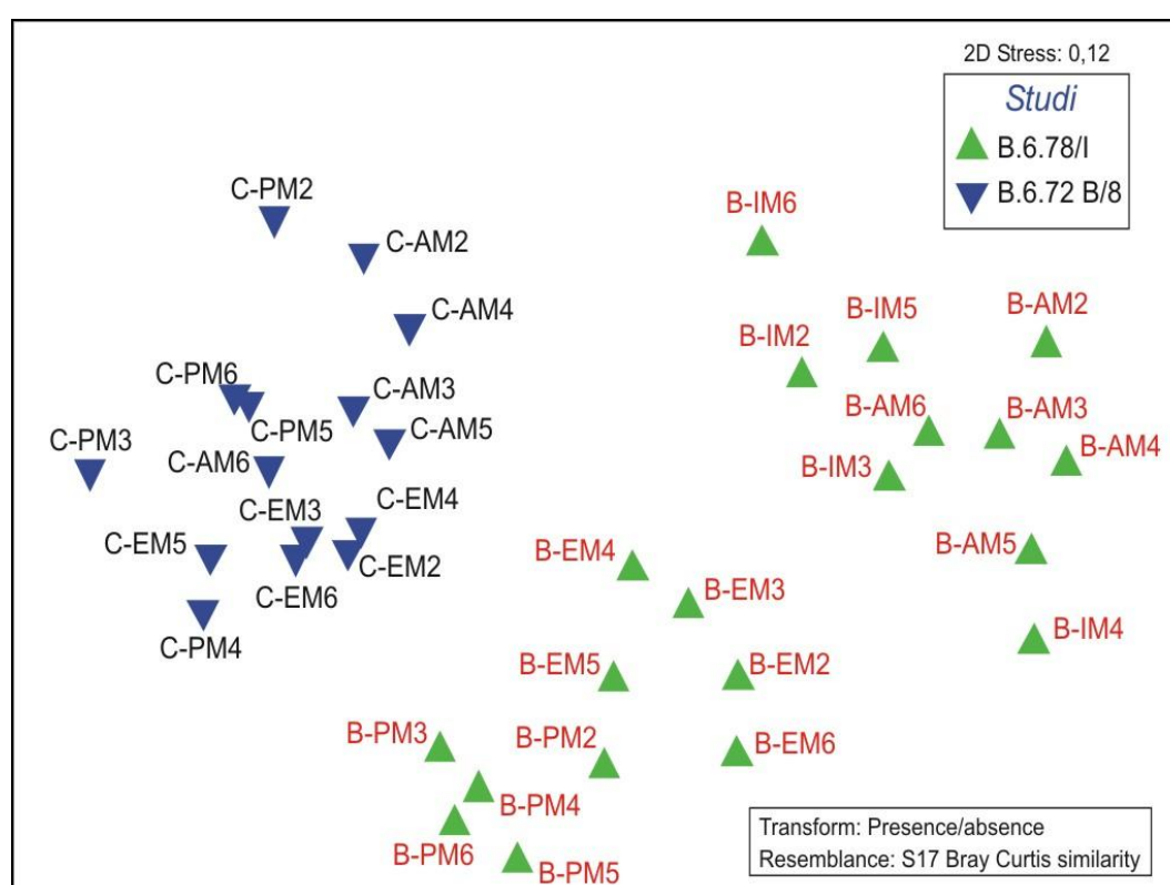
Figura A.5 - MultiDimensional Scaling (MDS) dell'ordinamento in base alla similarità della comunità epifitica nelle stazioni a Cymodocea nodosa (presenza-assenza). [B=B.6.78/I; C=B.6.72 B/8; I=inverno; P=primavera; E=estate; A=autunno].
