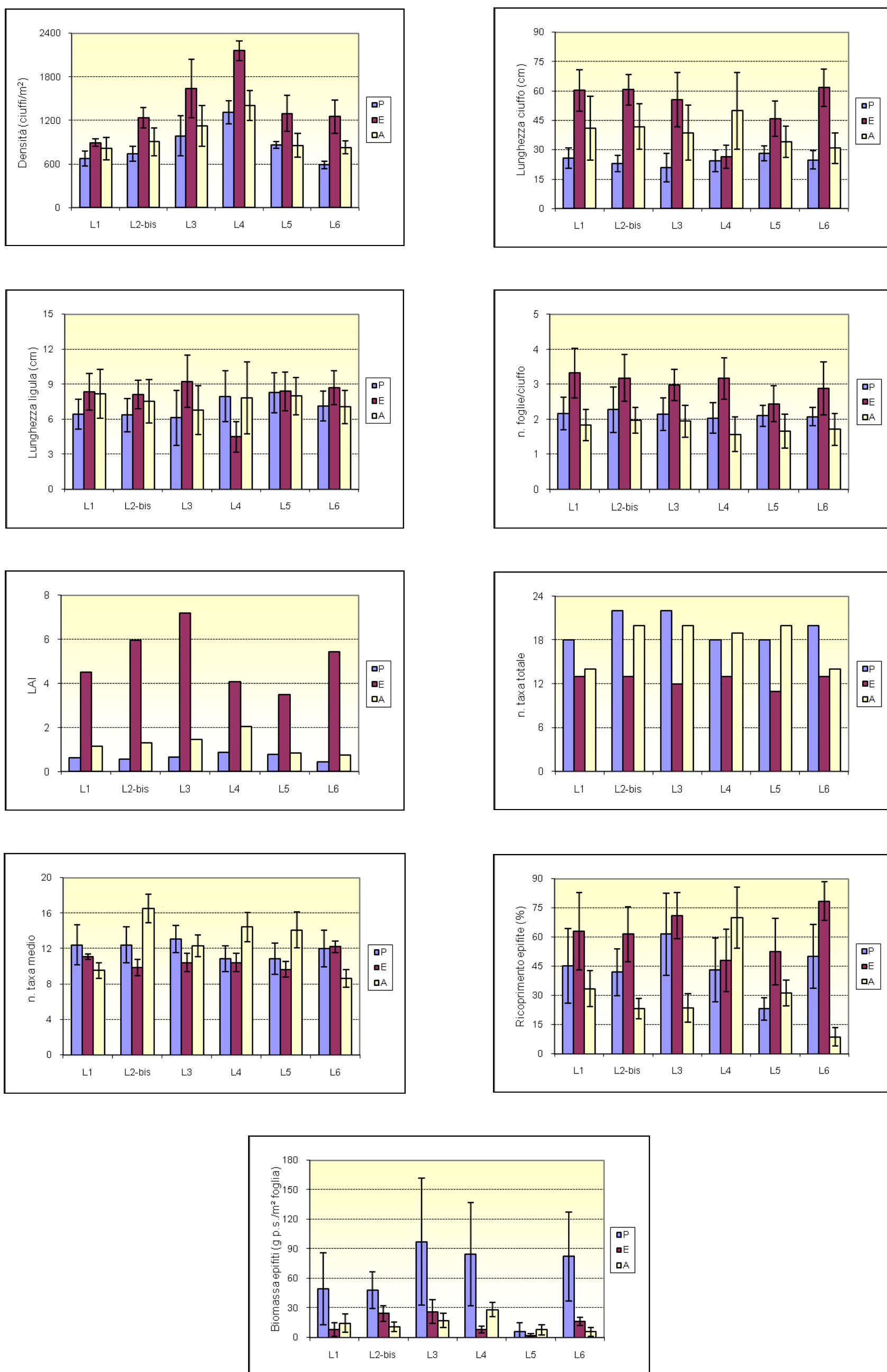
Figura A.1 - Bocca di porto di Lido: rappresentazione grafica e confronto di alcuni indicatori strutturali della Primavera (P), dell'Estate (E) e dell'Autunno (A) 2012.
