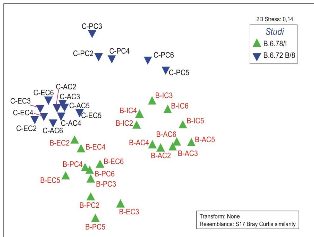
Figura A.7 - MultiDimensional Scaling (MDS) dell'ordinamento in base alla similarità della comunità epifitica nelle stazioni a Cymodocea nodosa (dati di ricoprimento senza trasformazione). [B=B.6.78/I; C=B.6.72 B/8; I=inverno; P=primavera; E=estate; A=autunno].
