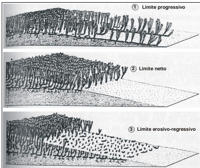
Figura 3.23 – Schema semplificato delle tipologie del limite delle praterie mutuato da Pergent et al. [1995] per Posidonia oceanica .
