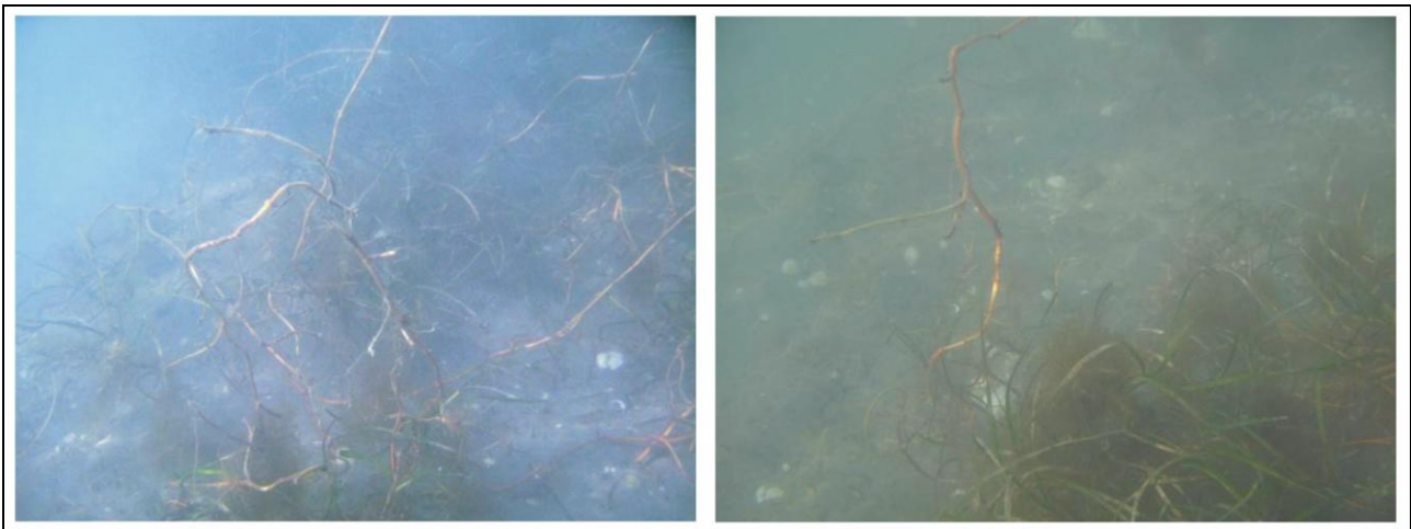
Figura 3.26 – Esempi di fenomeni erosivi al margine della prateria con rizomi esterni al sedimento.
