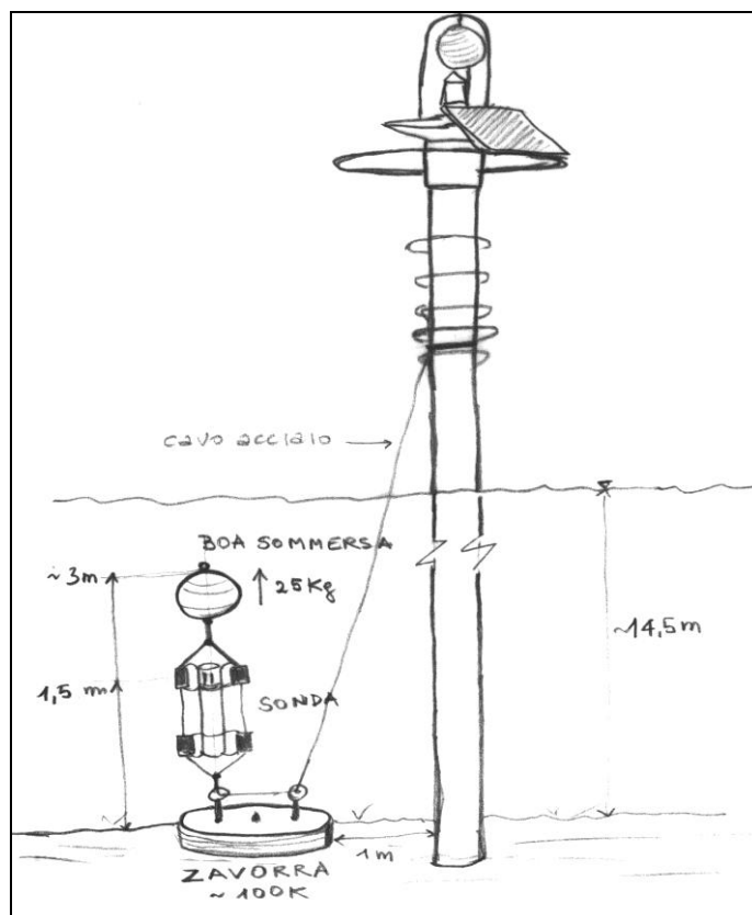
Figura 1.8. Schema del sistema di posizionamento e ancoraggio utilizzato nelle stazioni a mare.
