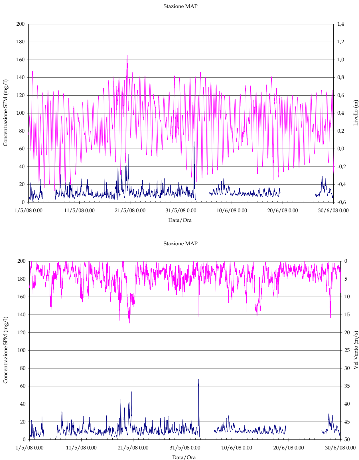
Figura 2.10 (a). Serie temporale della concentrazione di SPM e del livello idrico (in alto) e della velocità del vento (in basso) alla stazione MAP nel periodo Maggio-Giugno 2008.
