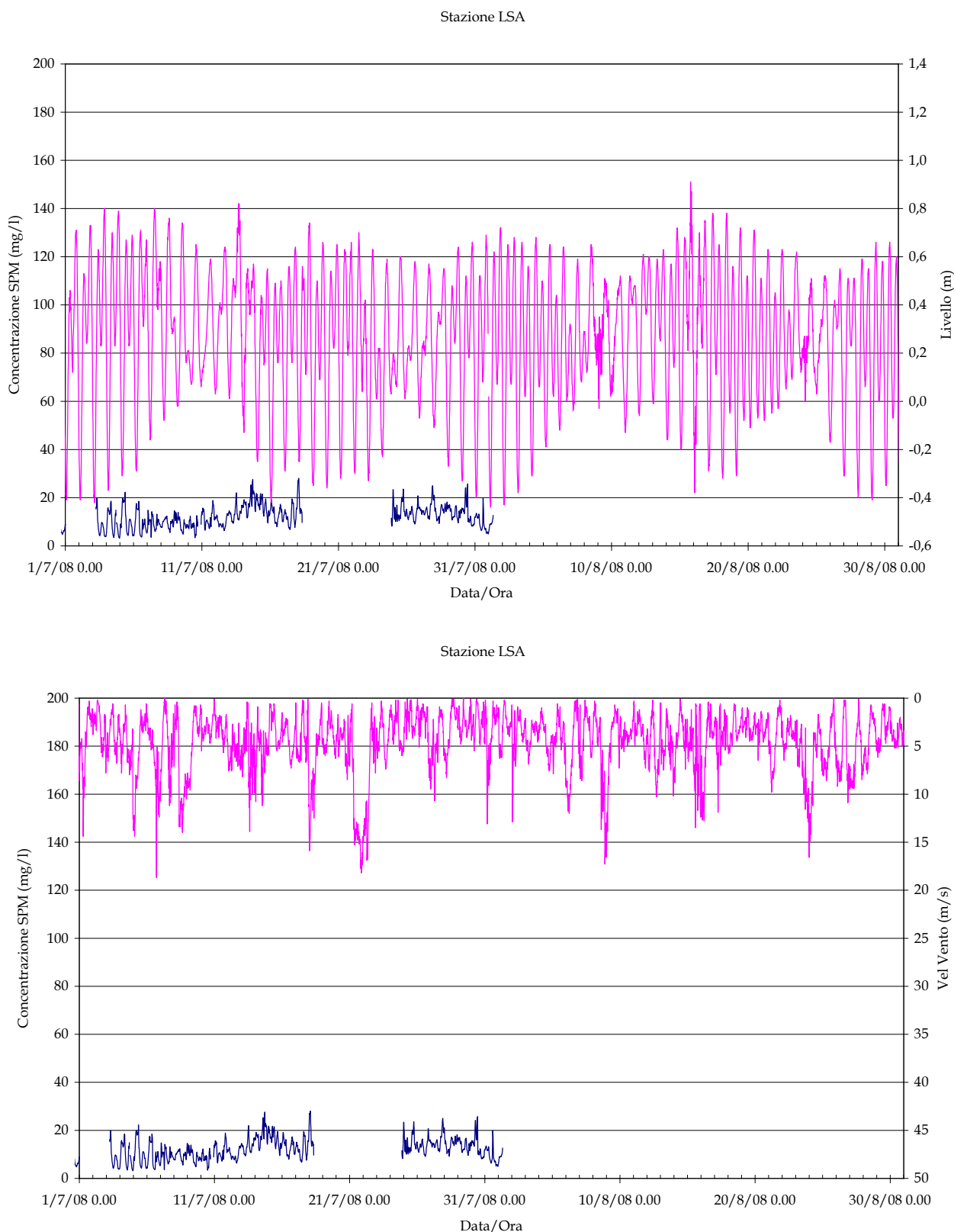
Figura 2.7 (b). Serie temporale della concentrazione di SPM e del livello idrico (in alto) e della velocità del vento (in basso) alla stazione LSA nel periodo Luglio-Agosto 2008.
