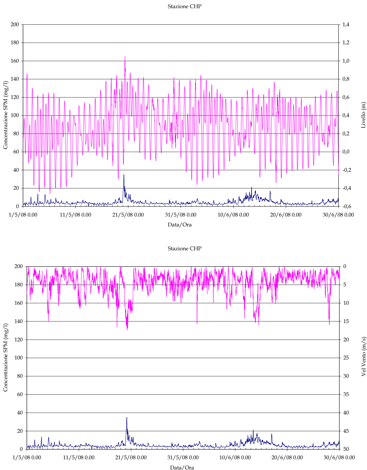
Figura 2.3 (a). Serie temporale della concentrazione di SPM e del livello idrico (in alto) e della velocità del vento (in basso) alla stazione CHP nel periodo Maggio-Giugno 2008.
