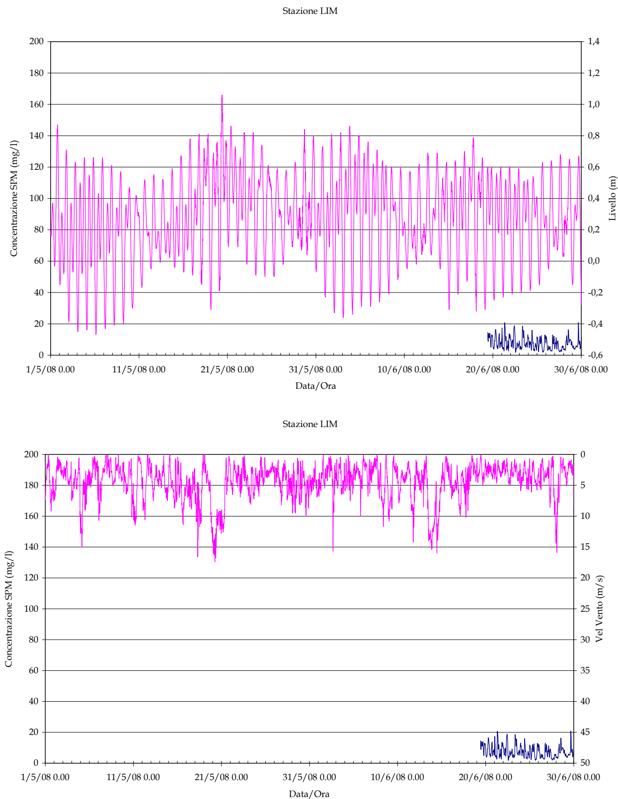
Figura 2.4 (a). Serie temporale della concentrazione di SPM e del livello idrico (in alto) e della velocità del vento (in basso) alla stazione LIM nel periodo Maggio-Giugno 2008.
