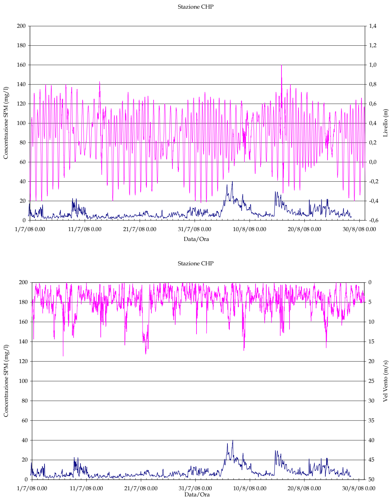
Figura 2.3 (b). Serie temporale della concentrazione di SPM e del livello idrico (in alto) e della velocità del vento (in basso) alla stazione CHP nel periodo Luglio-Agosto 2008.
