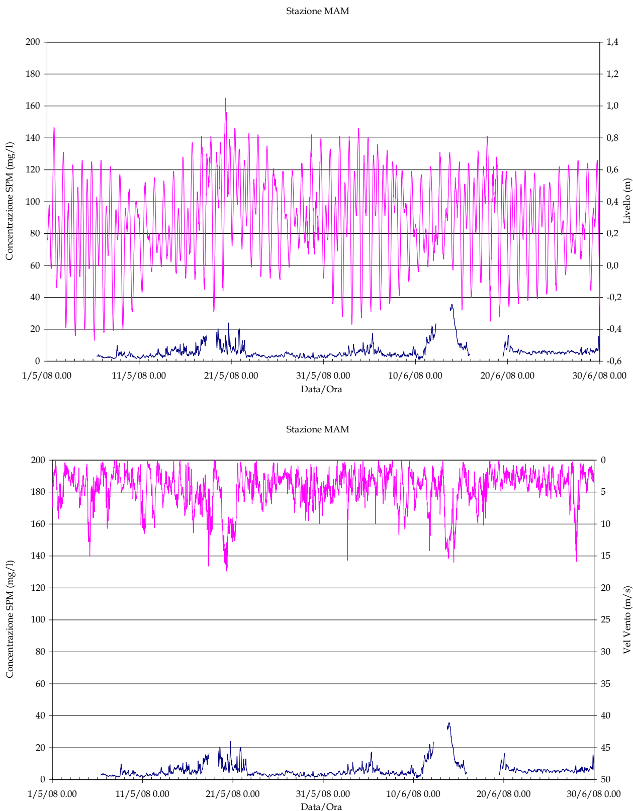
Figura 2.9 (a). Serie temporale della concentrazione di SPM e del livello idrico (in alto) e della velocità del vento (in basso) alla stazione MAM nel periodo Maggio-Giugno 2008.
