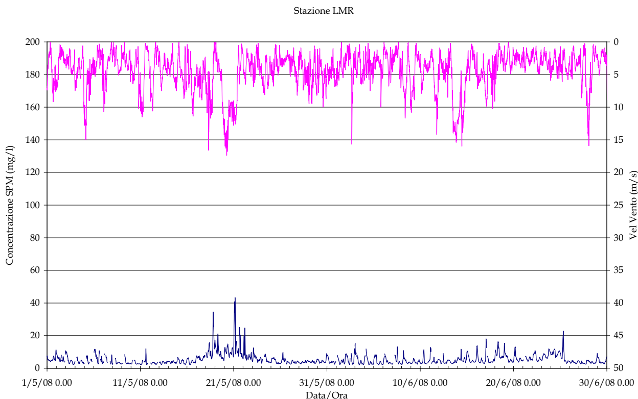
Figura 2.5 (a). Serie temporale della concentrazione di SPM e del livello idrico (in alto) e della velocità del vento (in basso) alla stazione LMR nel periodo Maggio-Giugno 2008.
