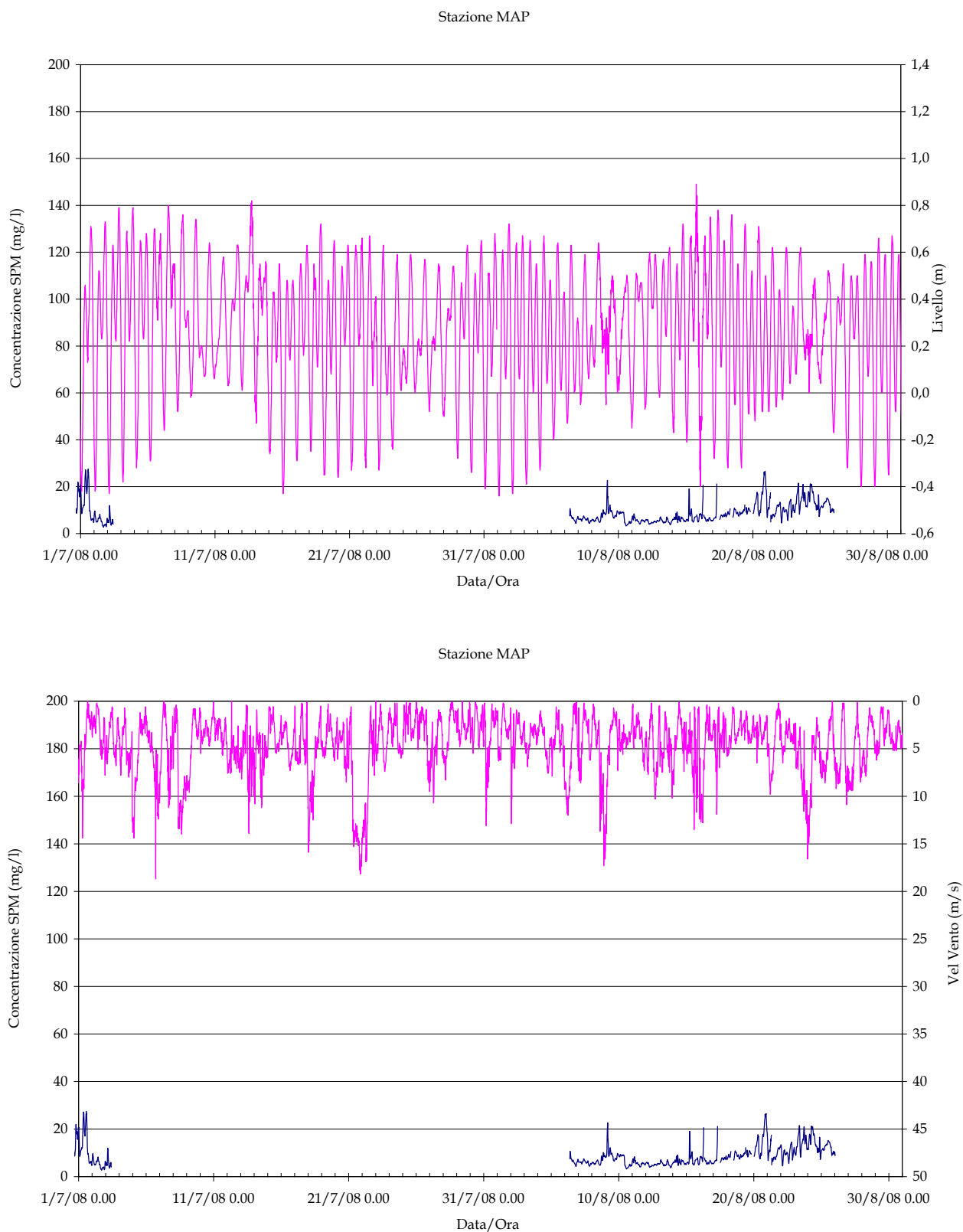
Figura 2.10 (b). Serie temporale della concentrazione di SPM e del livello idrico (in alto) e della velocità del vento (in basso) alla stazione MAP nel periodo Luglio-Agosto 2008.
