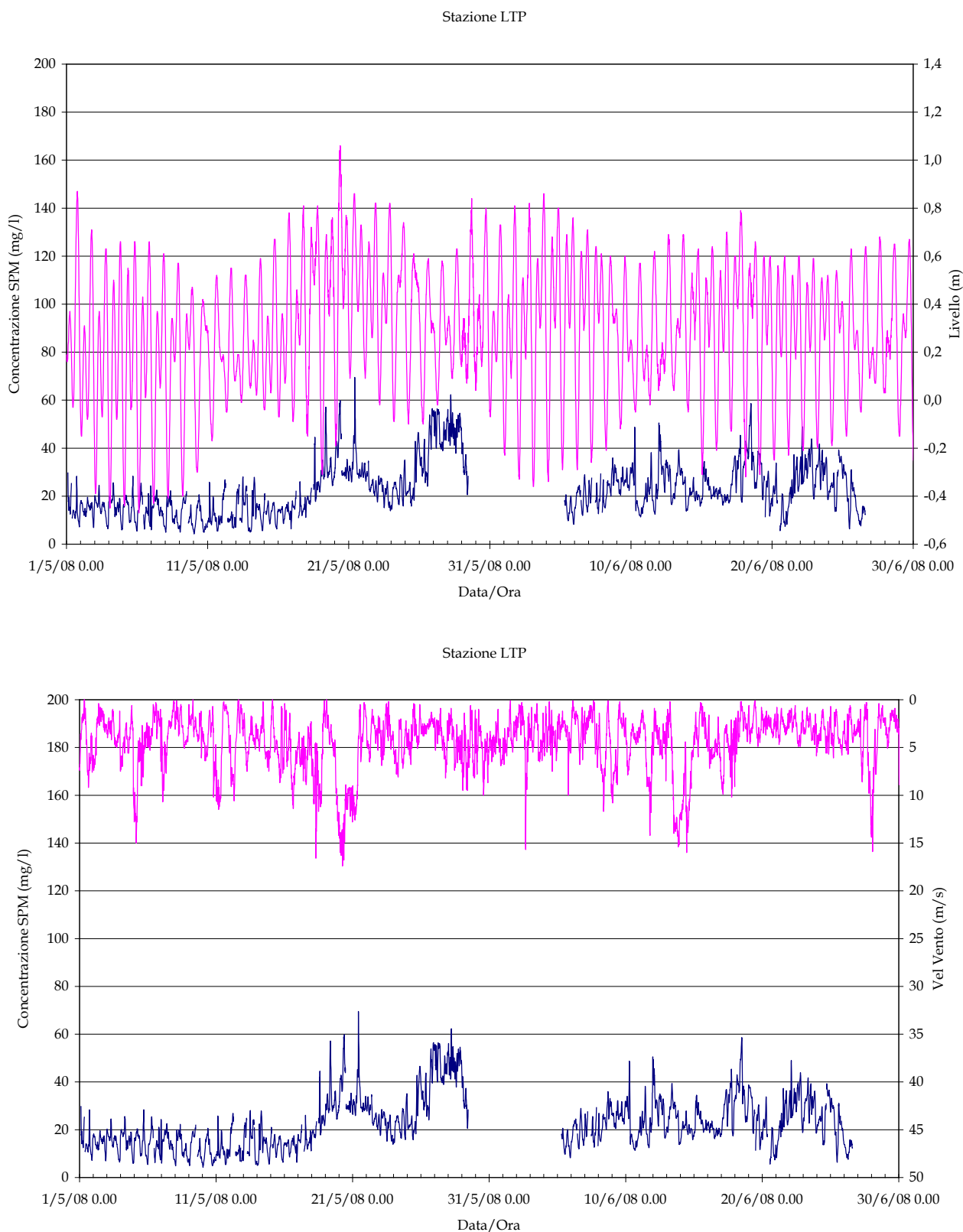
Figura 2.8 (a). Serie temporale della concentrazione di SPM e del livello idrico (in alto) e della velocità del vento (in basso) alla stazione LTP nel periodo Maggio-Giugno 2008.
