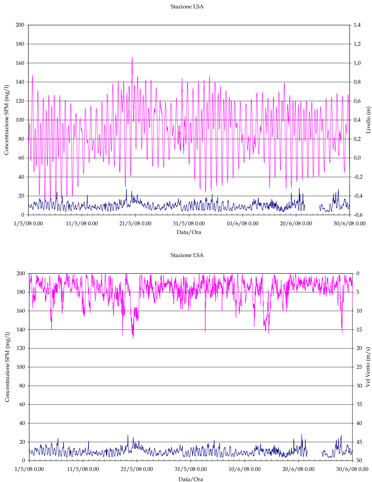
Figura 2.7 (a). Serie temporale della concentrazione di SPM e del livello idrico (in alto) e della velocità del vento (in basso) alla stazione LSA nel periodo Maggio-Giugno 2008
