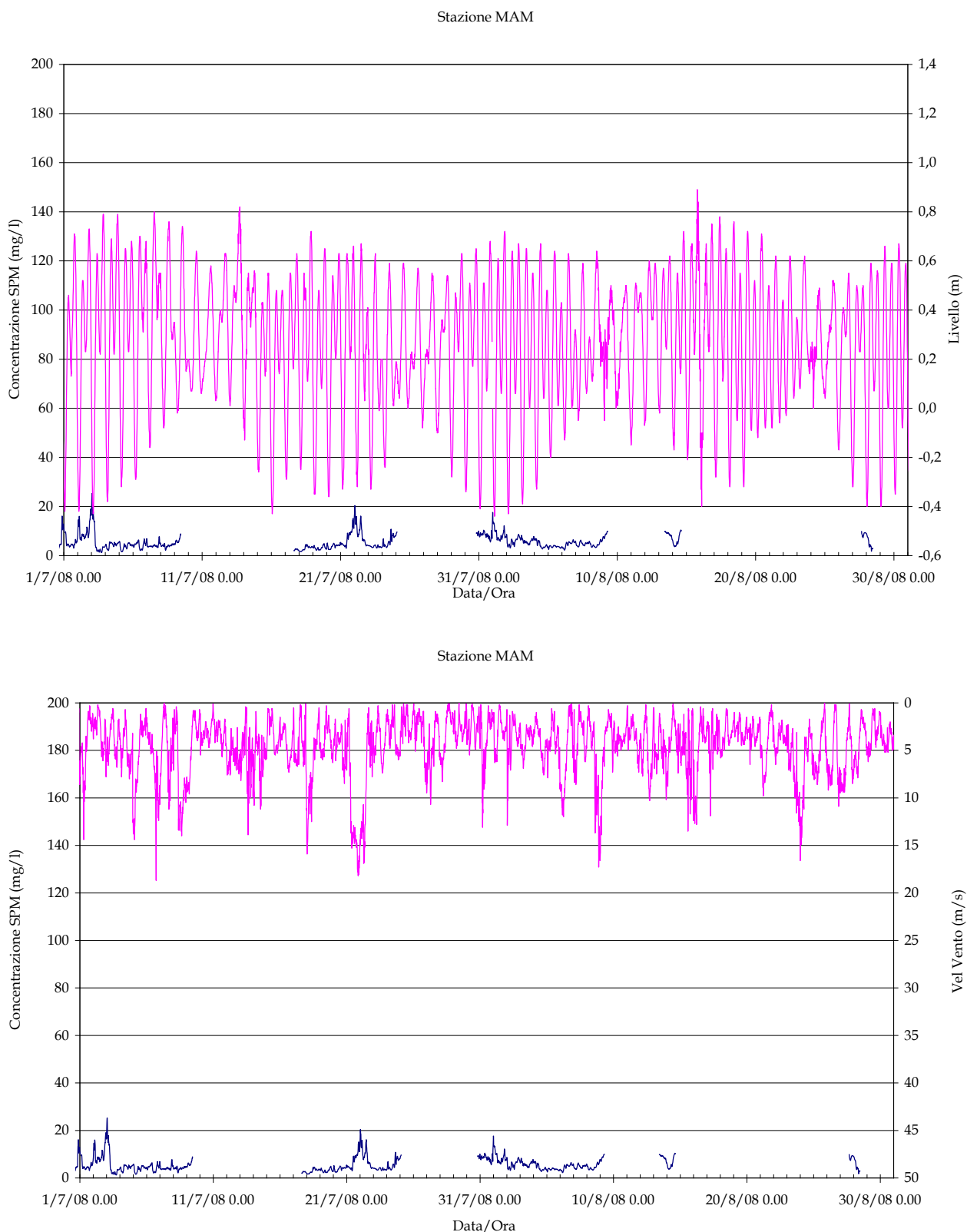
Figura 2.9 (b). Serie temporale della concentrazione di SPM e del livello idrico (in alto) e della velocità del vento (in basso) alla stazione MAM nel periodo Luglio-Agosto 2008.
