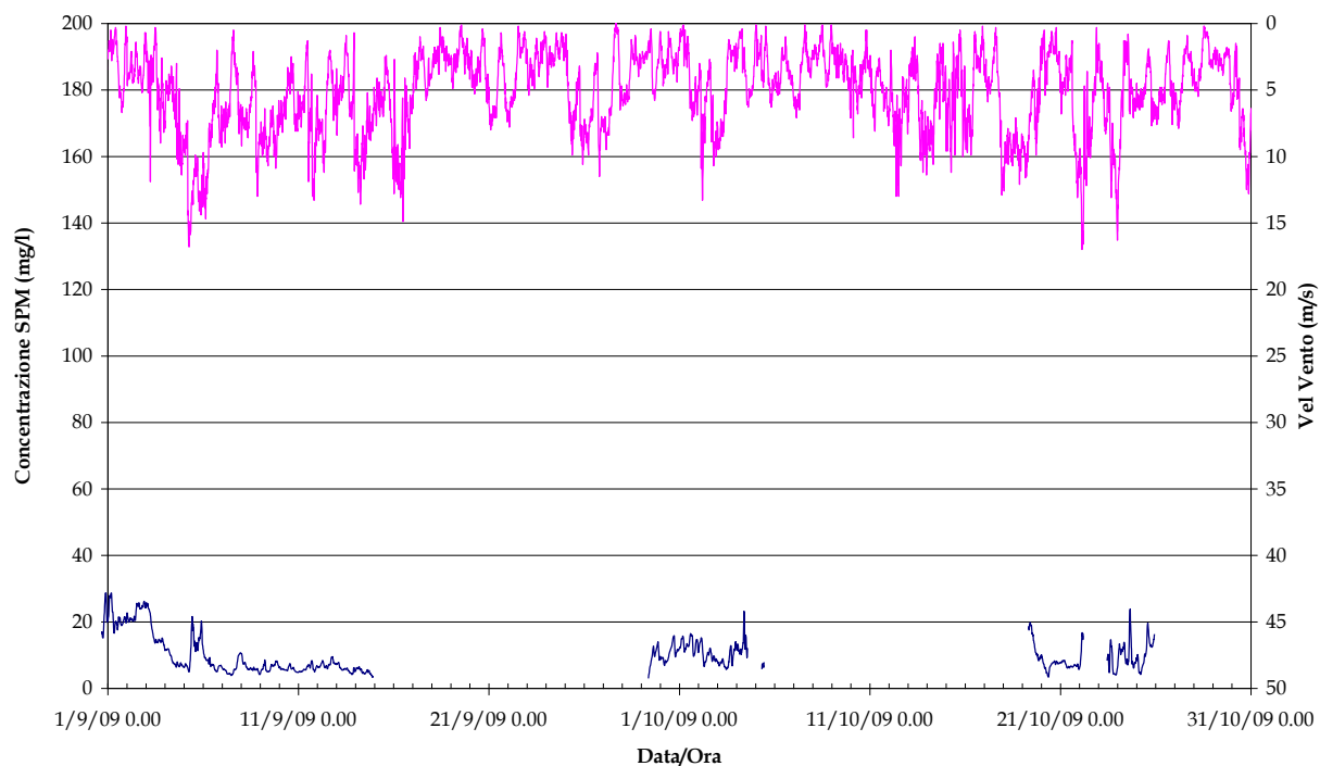
Figura 2.4 (a). Serie temporale della concentrazione di SPM e del livello idrico (in alto) e della velocità del vento (in basso) alla stazione MAM nel periodo Settembre-Ottobre 2009.
