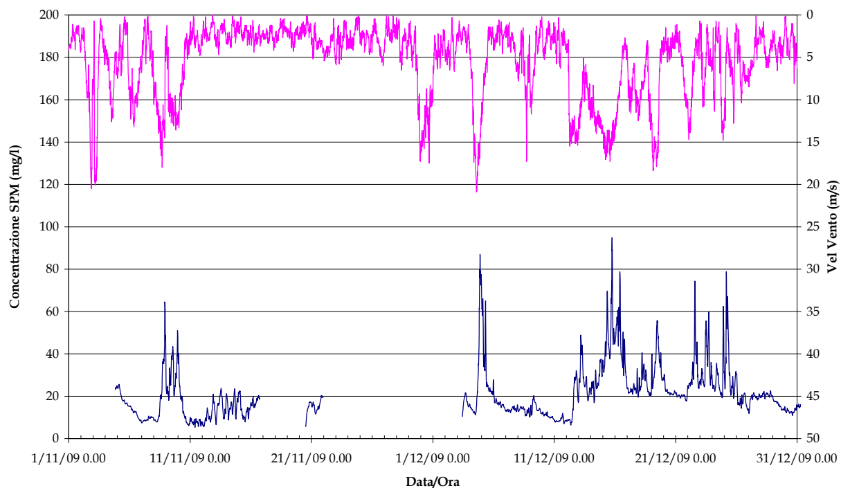
Figura 2.4 (b). Serie temporale della concentrazione di SPM e del livello idrico (in alto) e della velocità del vento (in basso) alla stazione MAM nel periodo Novembre-Dicembre2009.
