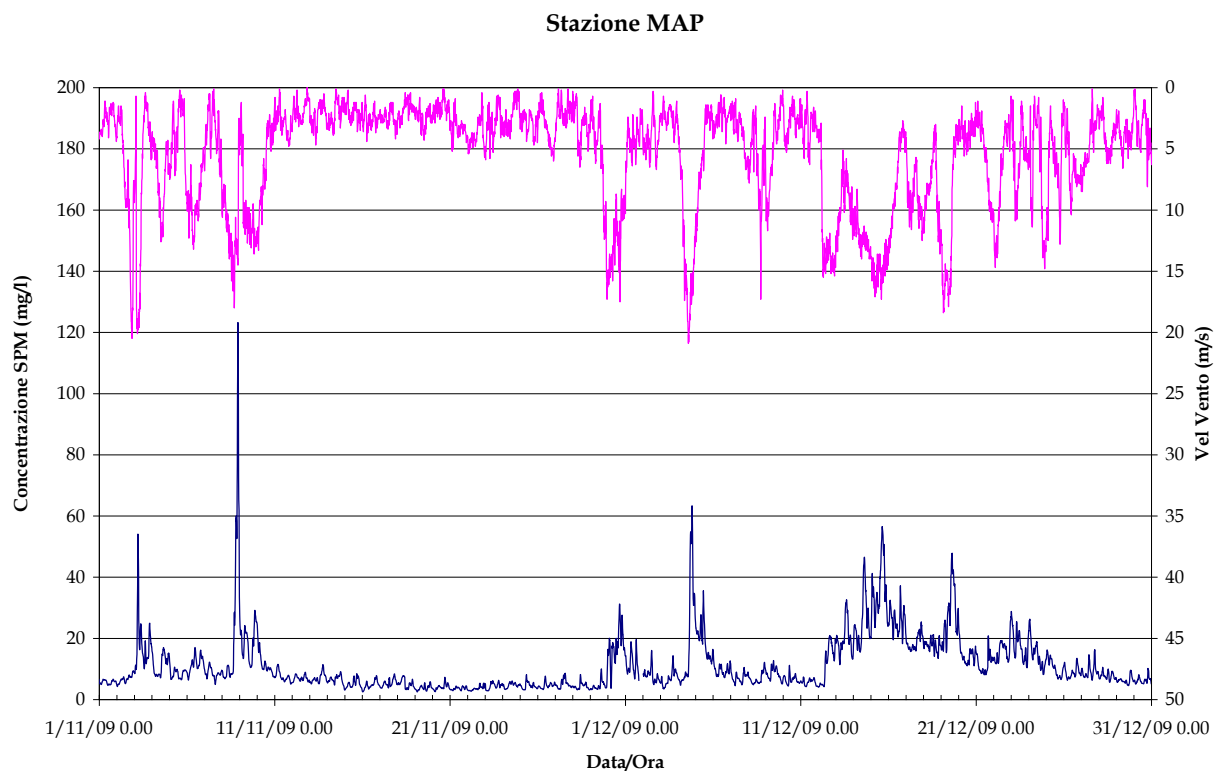
Figura 2.5 (b). Serie temporale della concentrazione di SPM e del livello idrico (in alto) e della velocità del vento (in basso) alla stazione MAP nel periodo Novembre-Dicembre2009.
