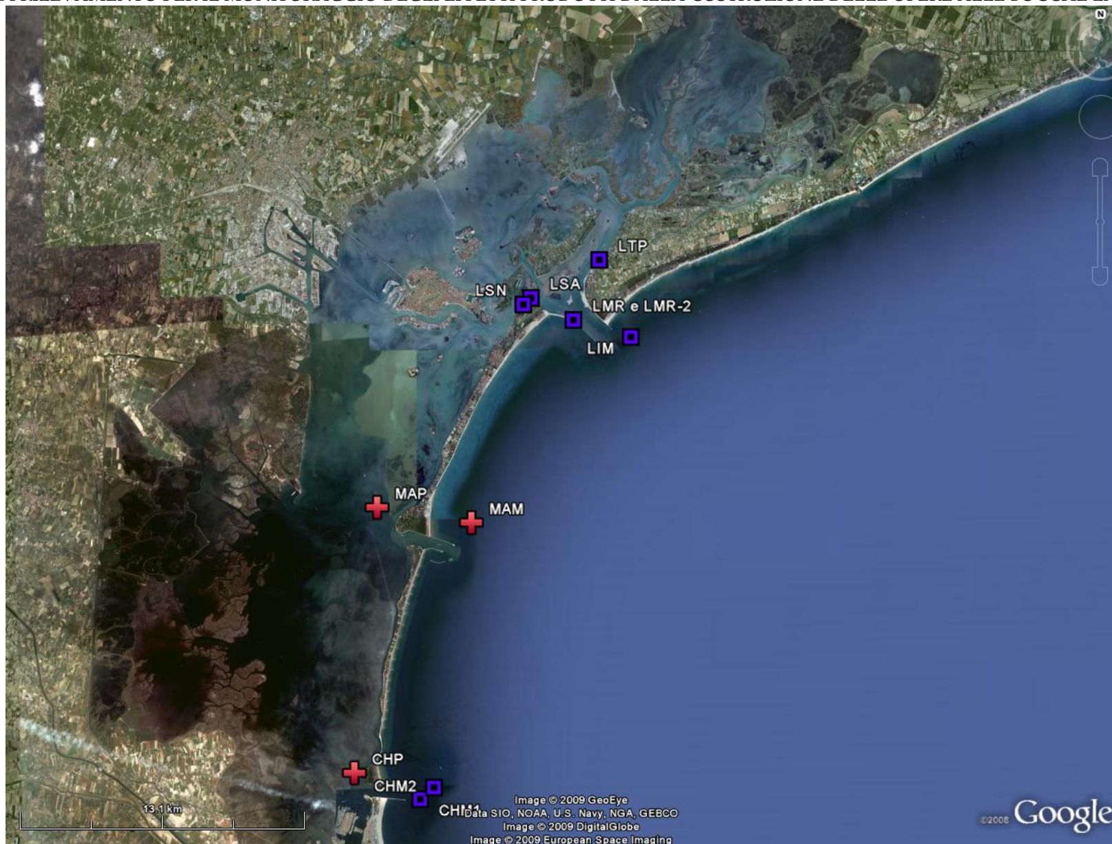
Figura 1.1. La rete delle stazioni fisse per la misura della torbidità in continuo. In rosso le stazioni attive nel periodo 2009-2010.
