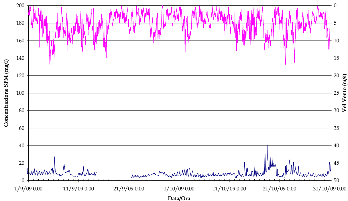
Figura 2.3 (a). Serie temporale della concentrazione di SPM e del livello idrico (in alto) e della velocità del vento (in basso) alla stazione CHP nel periodo Settembre-Ottobre 2009.
