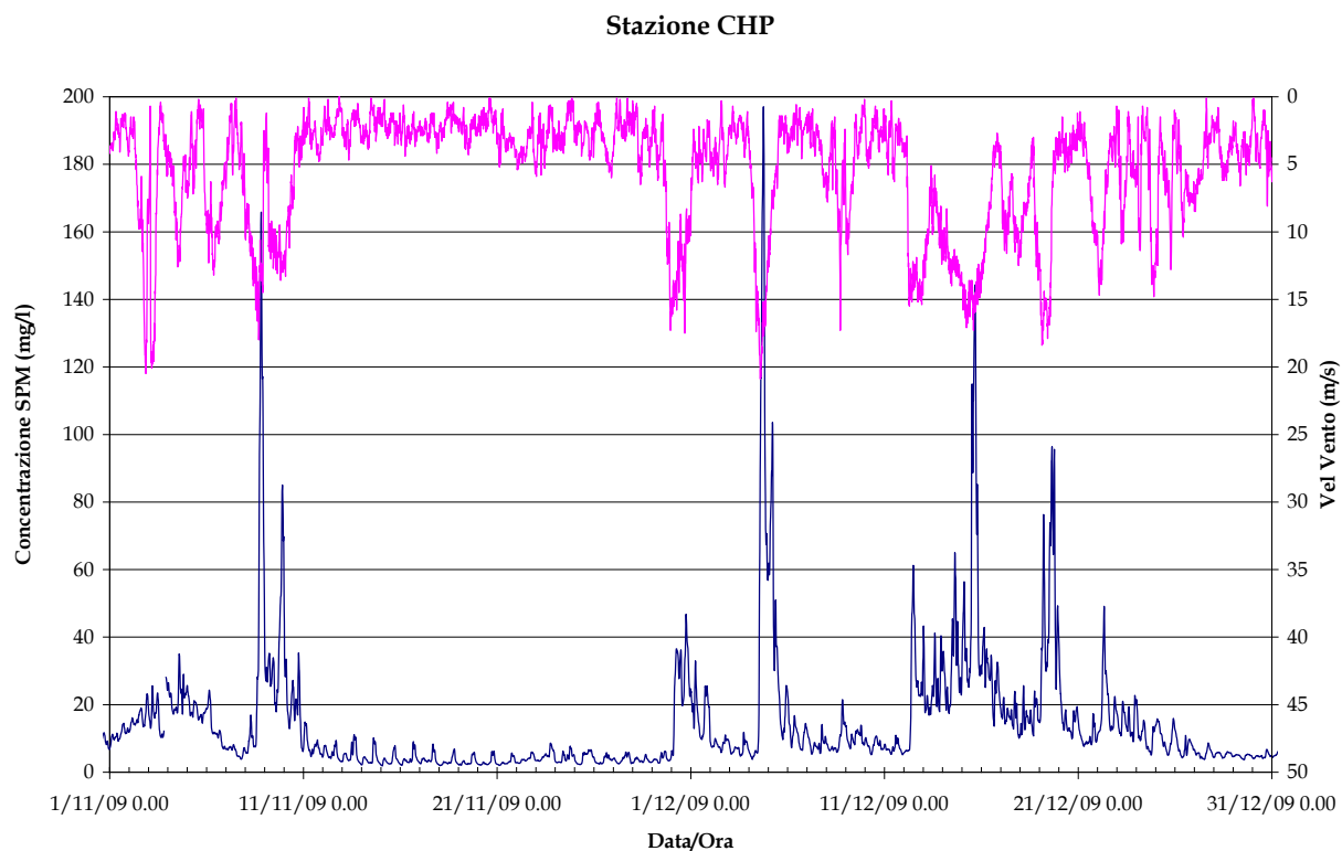
Figura 2.3 (b). Serie temporale della concentrazione di SPM e del livello idrico (in alto) e della velocità del vento (in basso) alla stazione CHP nel periodo Novembre-Dicembre2009.
