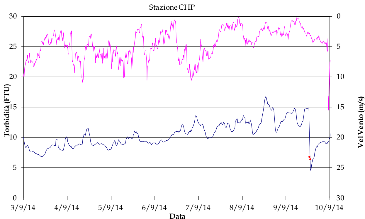
Figura 2.9. Esempio della presenza di deriva progressiva dei valori di torbidità dovuta al fouling nella stazione CHP. I pallini rossi rappresentano i valori di concentrazione misurati nei campioni d'acqua prelevati prima e dopo l'intervento di manutenzione.
