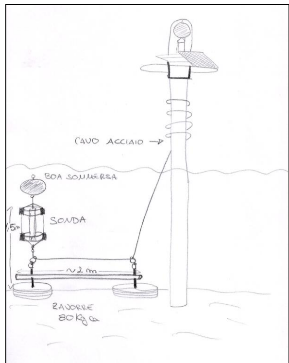
Figura 2.5. Schema del sistema di posizionamento e ancoraggio utilizzato nelle stazioni a mare.
