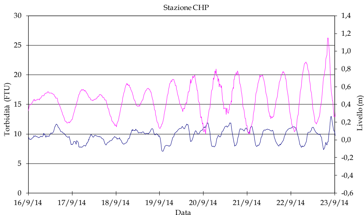
Figura 2.8. Esempio di andamento indisturbato della torbidità nella stazione CHP (linea blu) in relazione all'andamento della marea (linea rosa).
